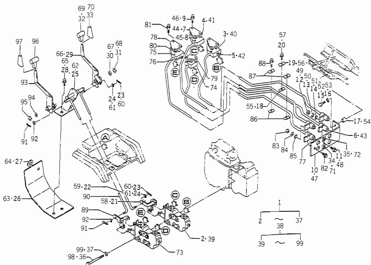
FIG.105 VALVE (SUB/1H) SET SYSTEM (OPTION)
