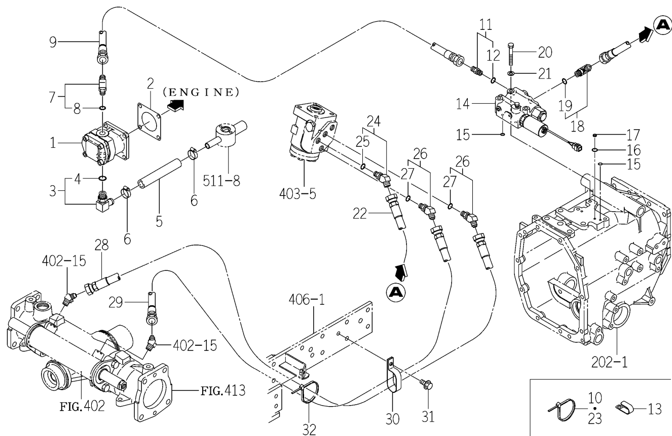
FIG.405 PIPING (SUB) SYSTEM (H TYPE)
