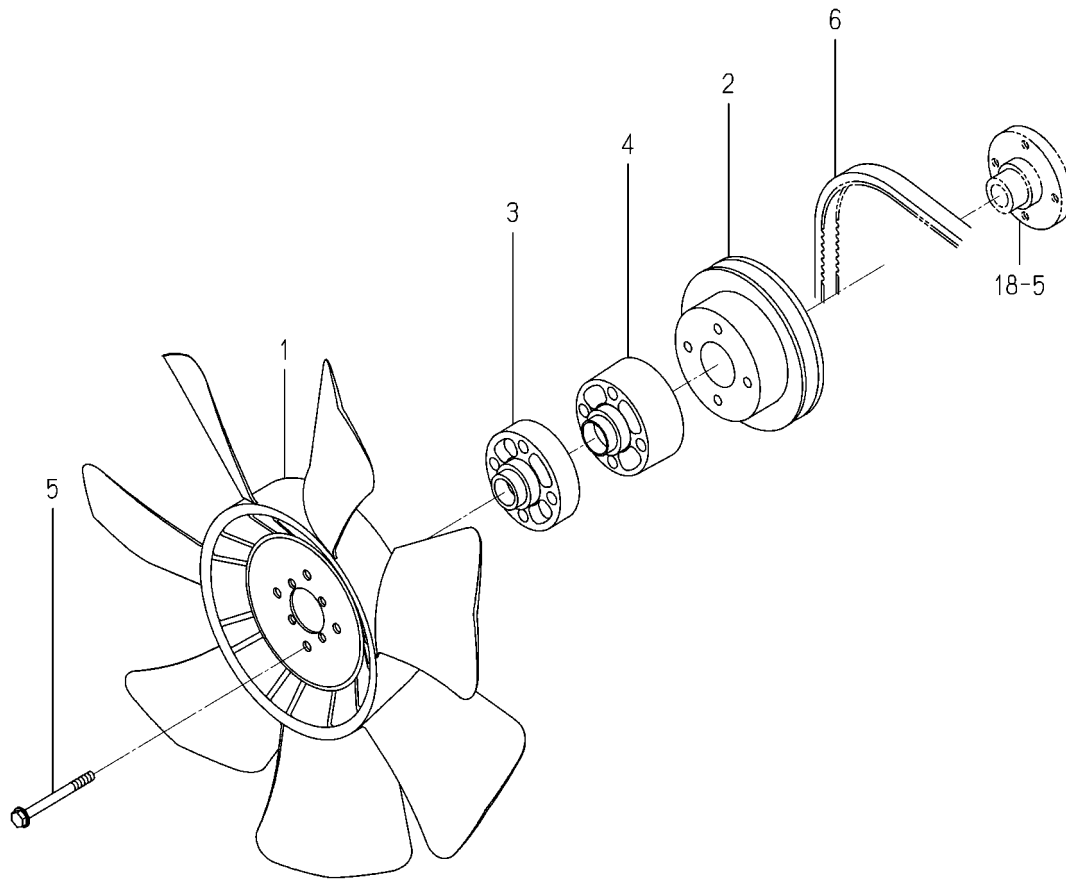
FIG. 19 COOLING FAN
