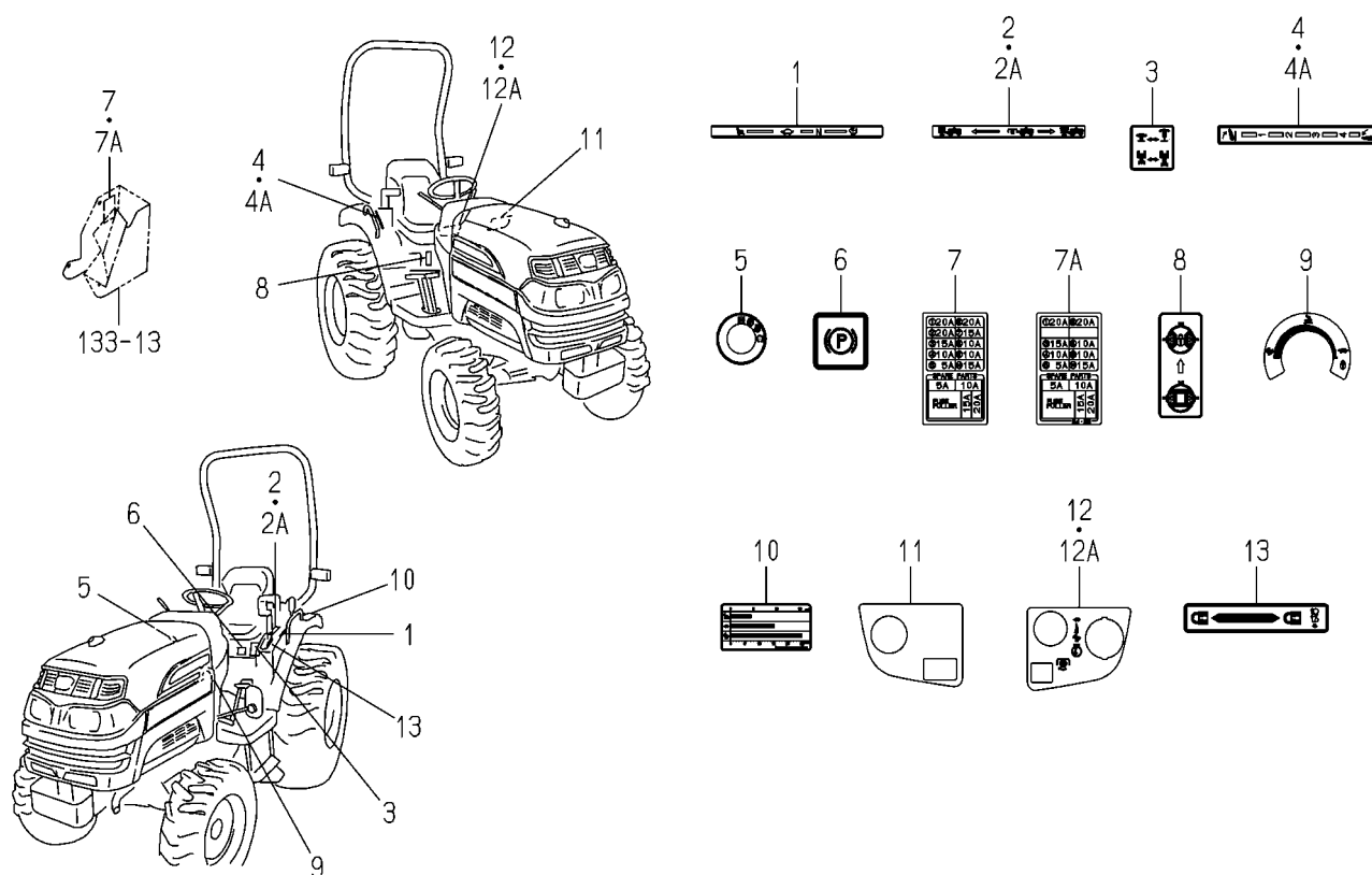
FIG.169 LABEL(CONTROL)(H TYPE)
