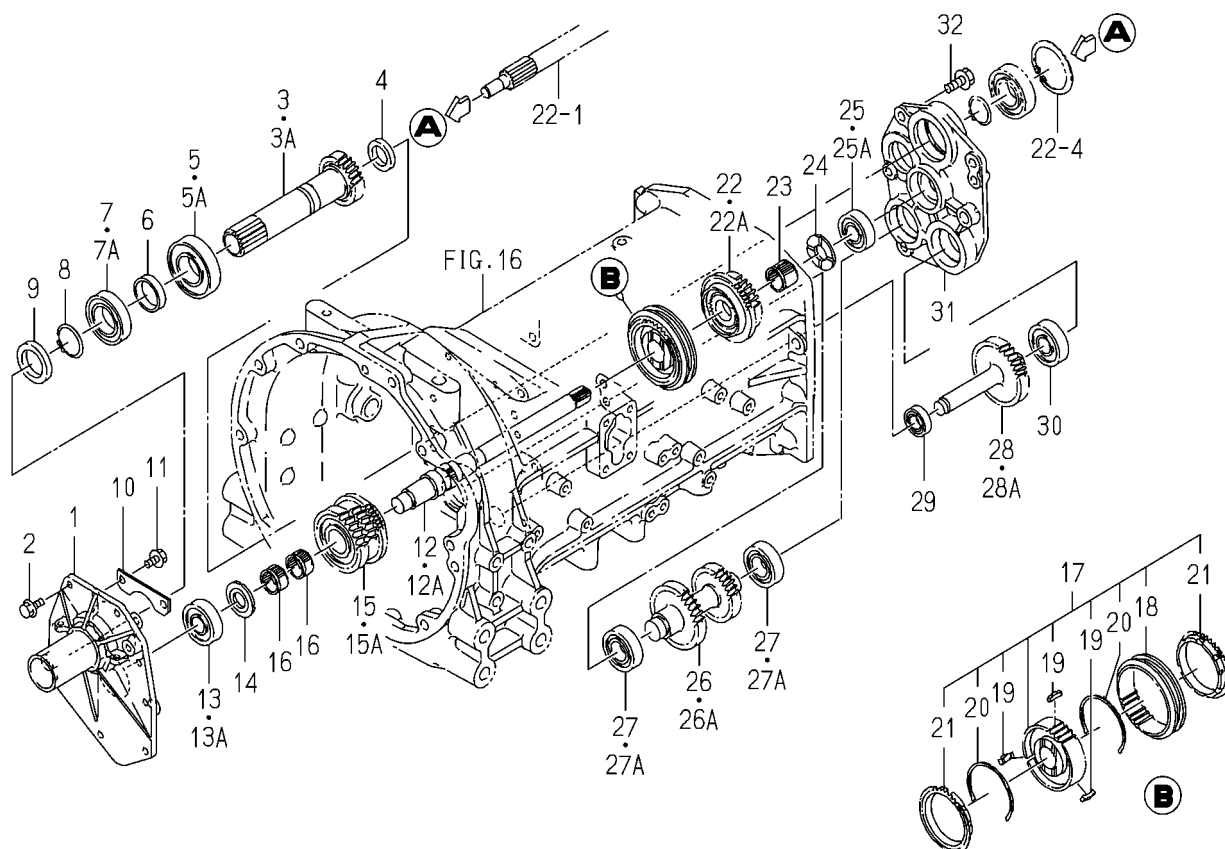
FIG. 20 GEAR(INPUT)SYSTEM(SK TYPE)
