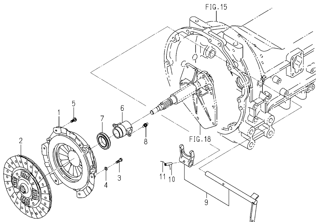
FIG. 11 CLUTCH(MAIN)SYSTEM (V TYPE EXCEPT SK)
