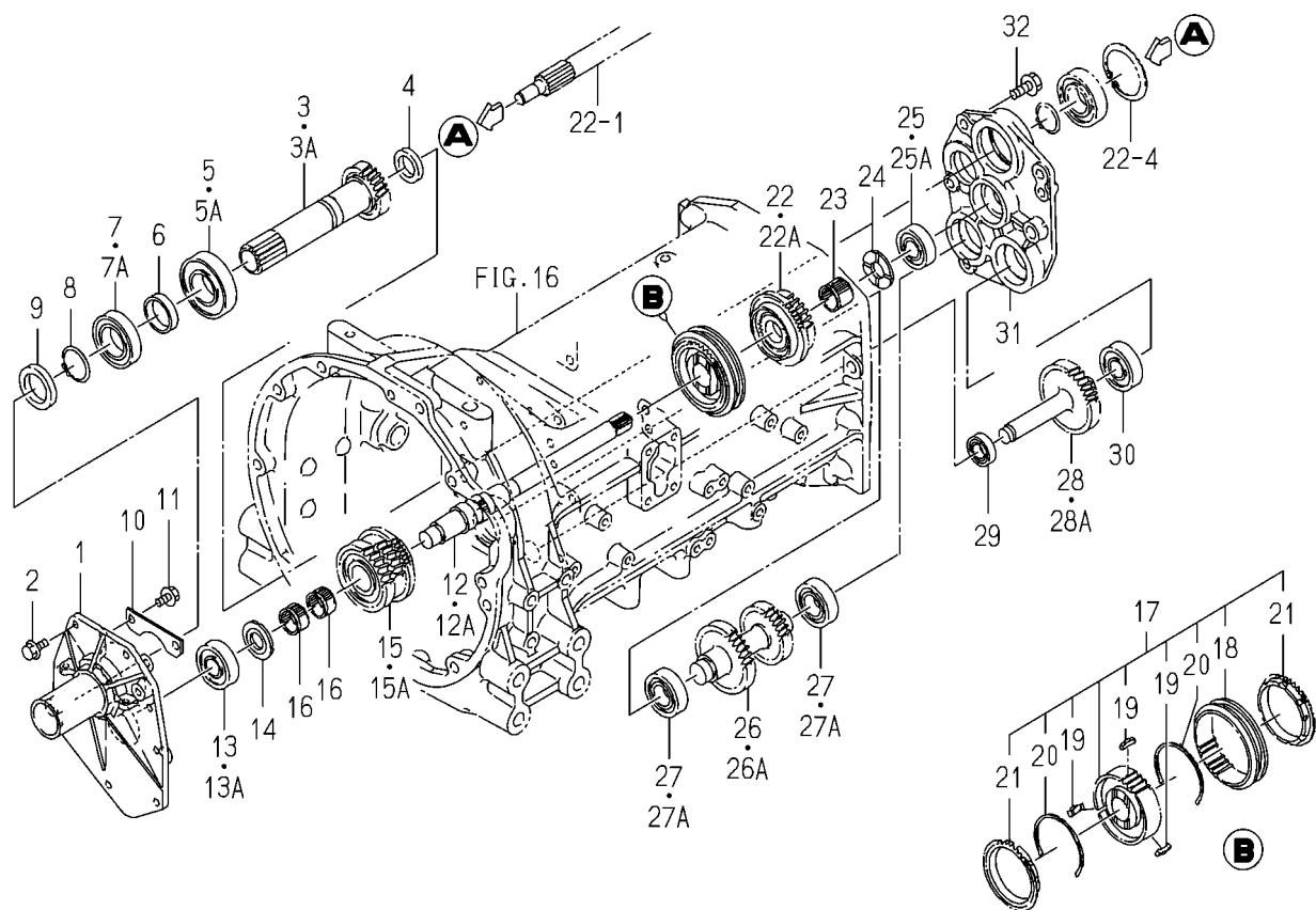
FIG. 20 GEAR(INPUT)SYSTEM(SK TYPE)
