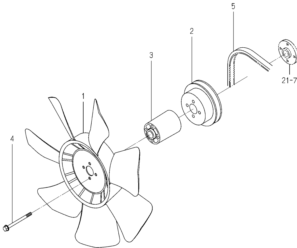
FIG. 22 COOLING FAN
