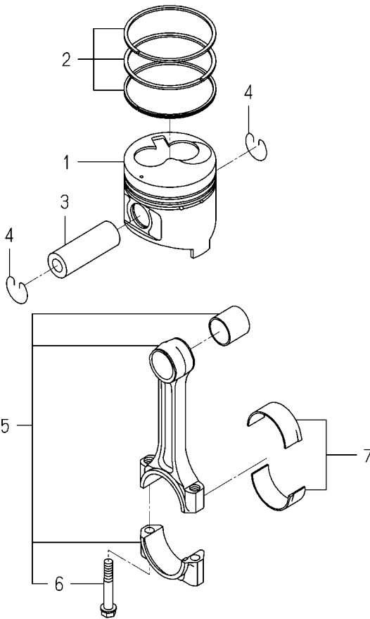
FIG. 14 PISTON
