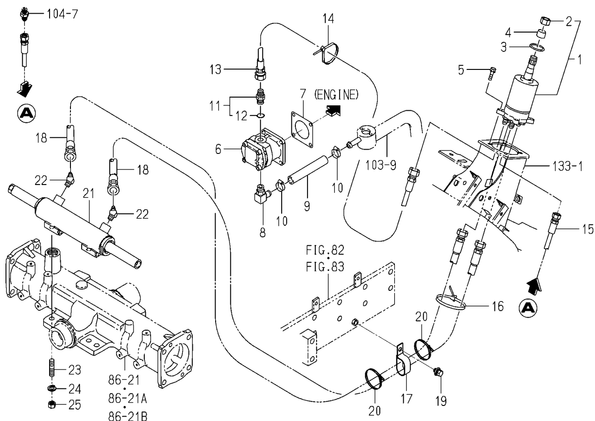
FIG. 81 STEERING(POWER)SYSTEM(HJ TYPE)
