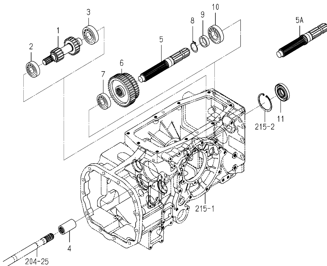
FIG.211 GEAR(PTO)SYSTEM(TG5395)
