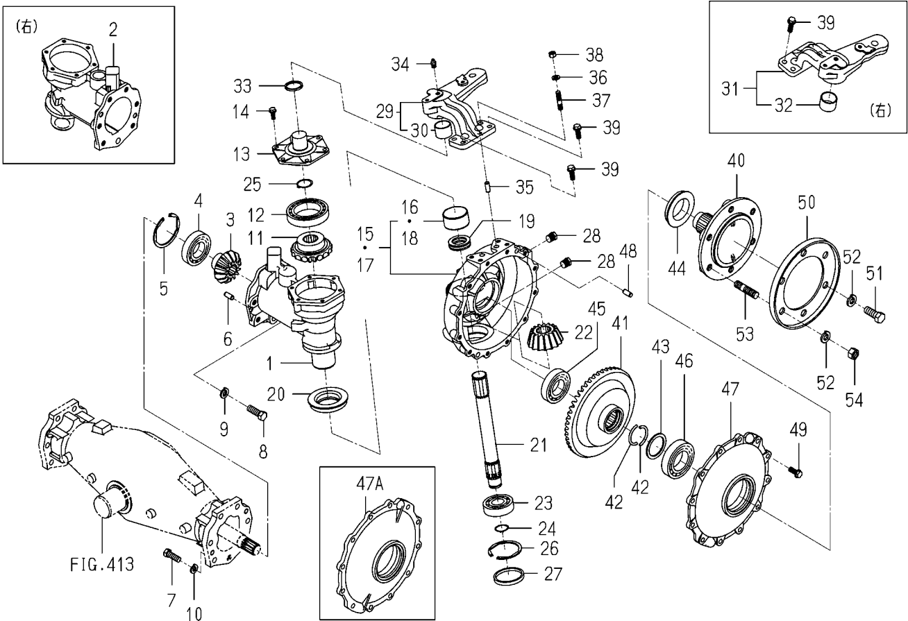
FIG.414 CASE(GEAR/FRONT)SYSTEM(TG5475)
