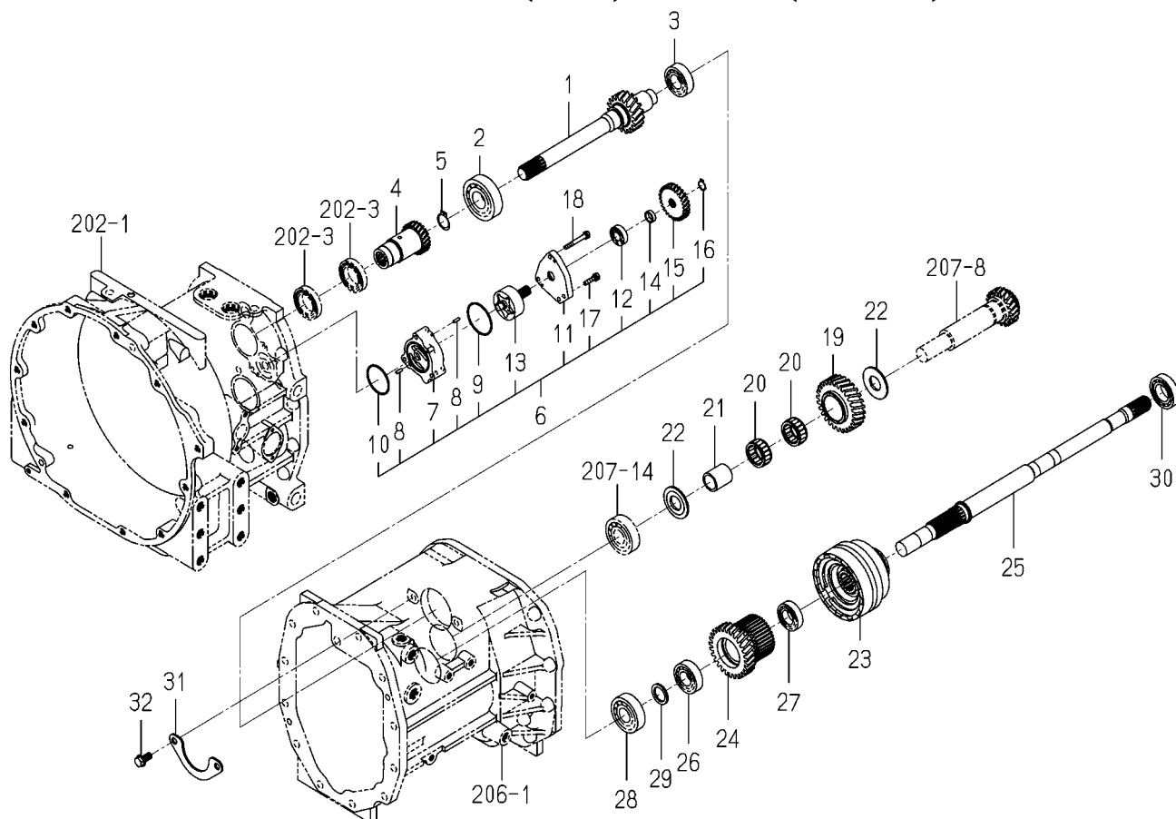
FIG.205 GEAR(PTO)SYSTEM(TG5475)
