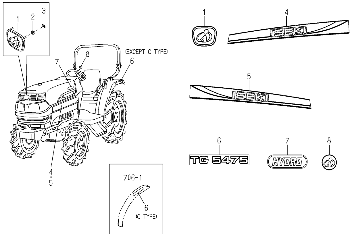
FIG.902 ORNAMENT(TG5475)
