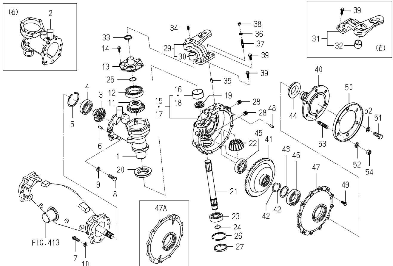
FIG.414 CASE(GEAR/FRONT)SYSTEM(TG5475)
