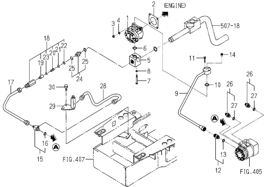
FIG.509 HYD.SYSTEM(SUB)(TG5475)(1/3)
