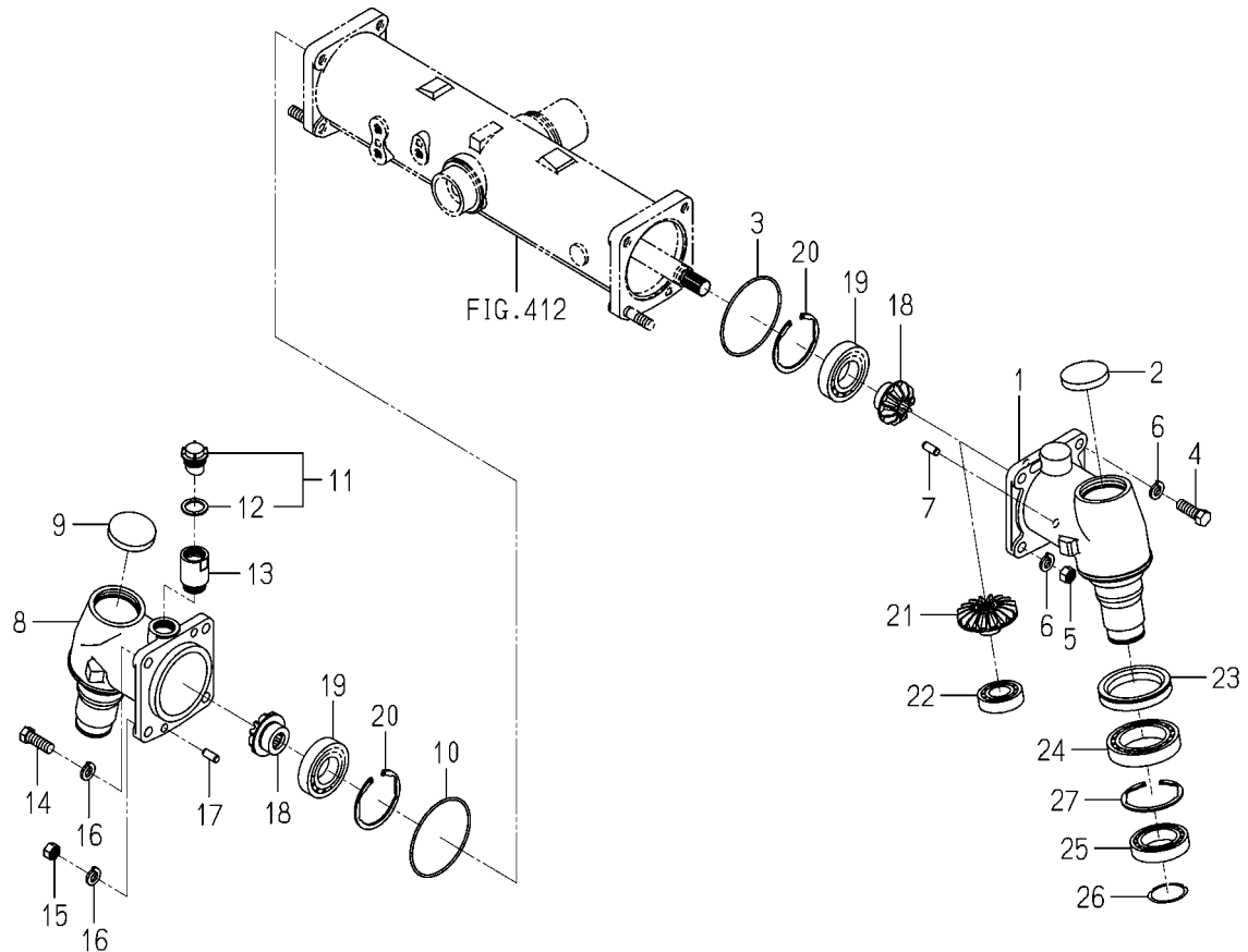
FIG.415 CASE(GEAR/FRONT)SYSTEM(TG5395)(1/2)
