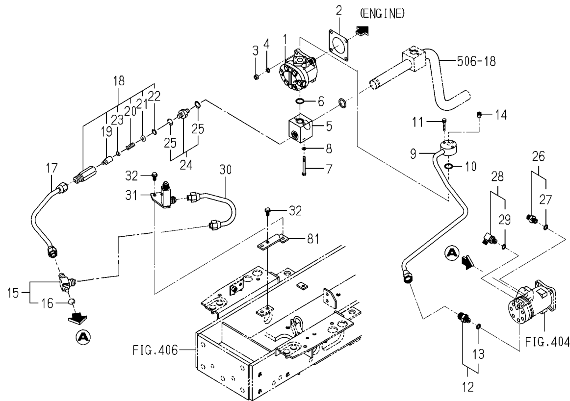
FIG.508 HYD.SYSTEM(SUB)(TG5395)(1/3)
