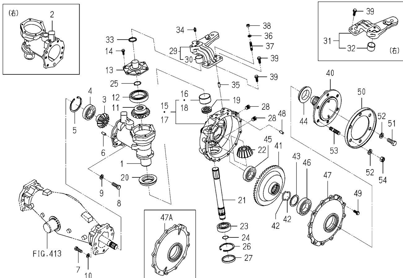
FIG.414 CASE(GEAR/FRONT)SYSTEM(TG5475)
