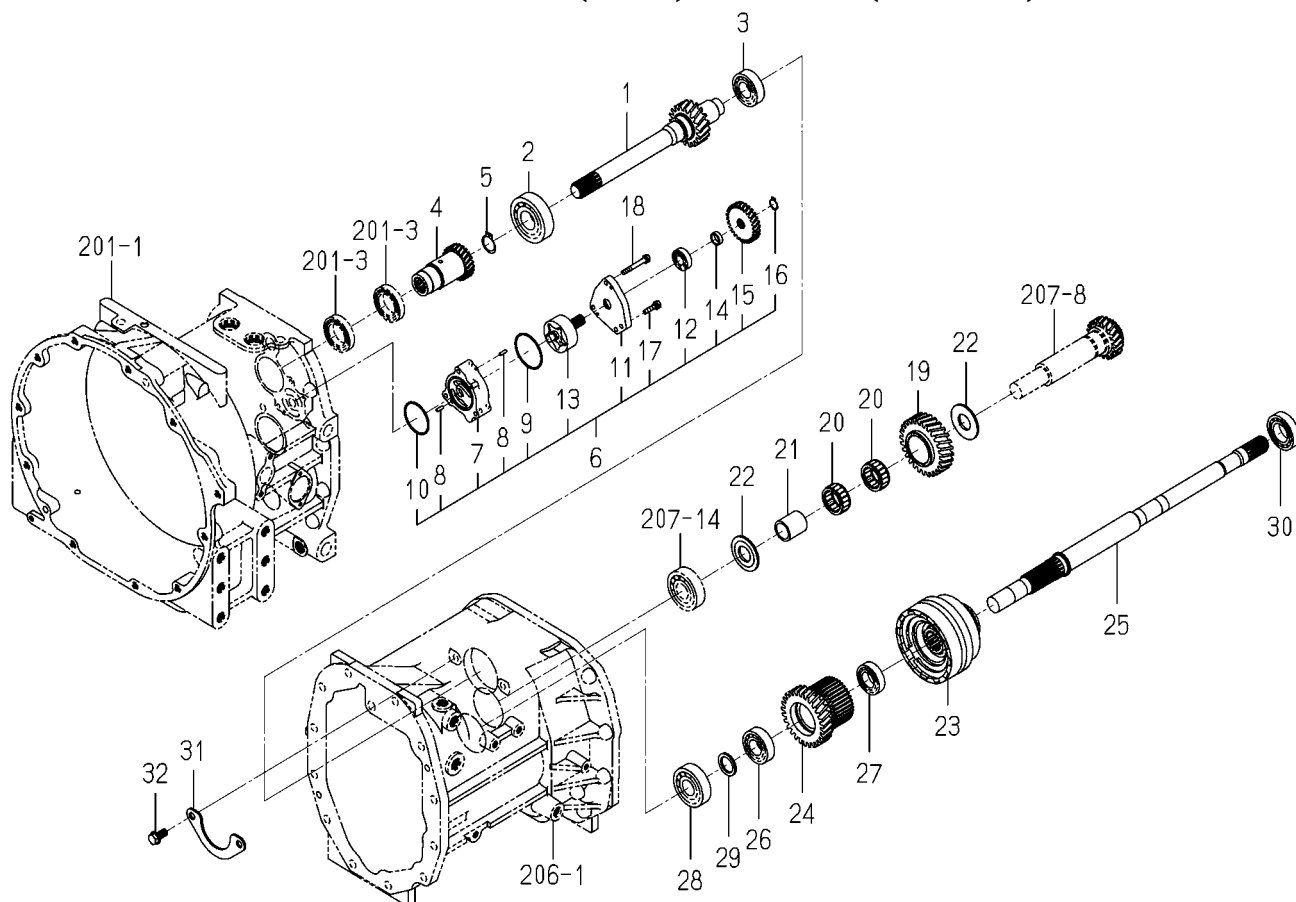
FIG.204 GEAR(PTO)SYSTEM(TG5395)
