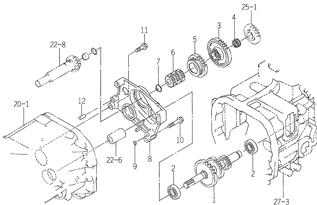
FIG. 24 GEAR (SUB) SYSTEM (H TYPE)
