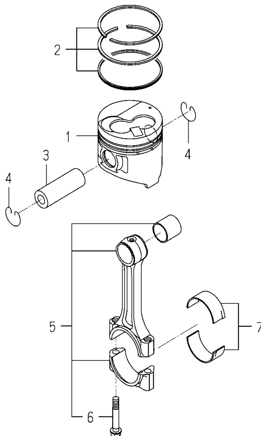
FIG. 13 PISTON
