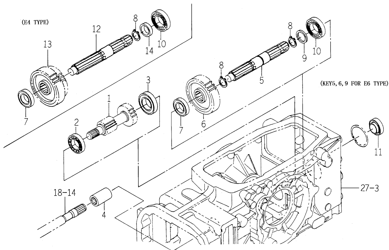
FIG. 26 GEAR (PTO) SYSTEM
