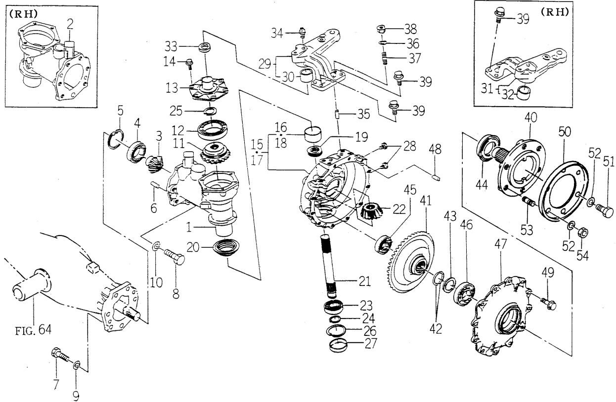
FIG. 66 CASE (GEAR/FRONT) SYSTEM (E4 TYPE)
