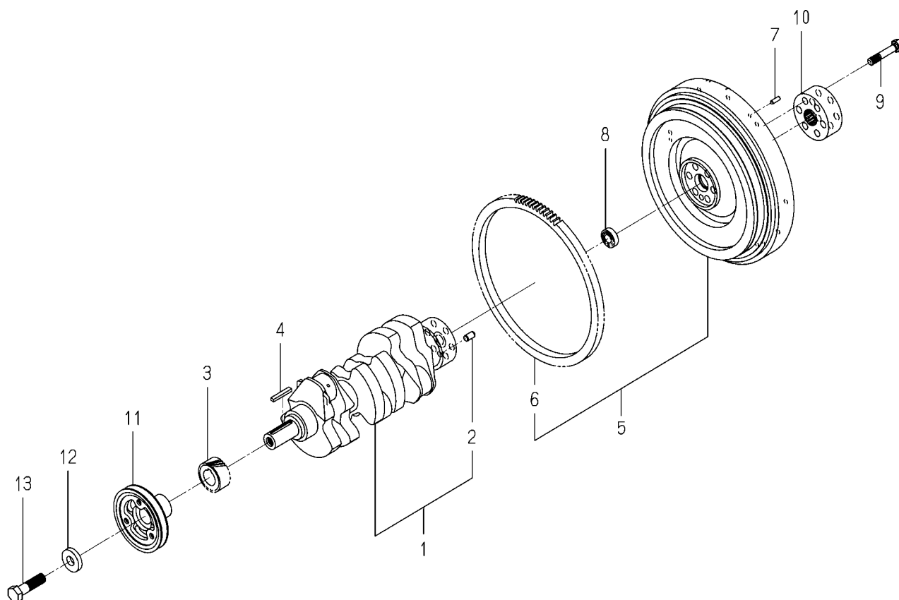
FIG. 15 CRANK SHAFT
