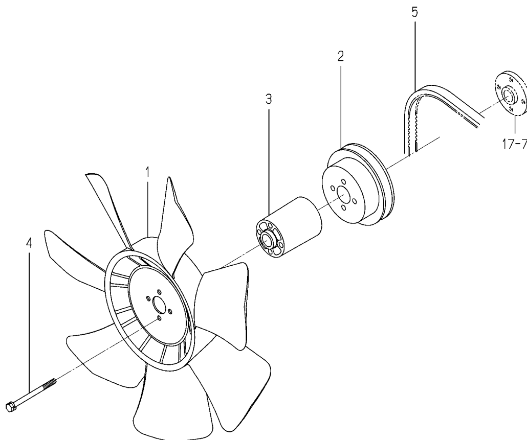
FIG. 18 COOLING FAN
