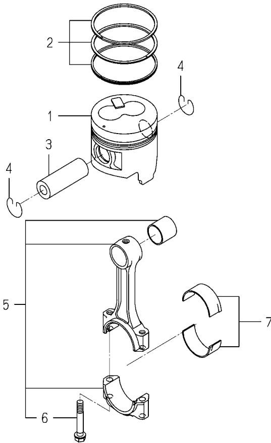
FIG. 14 PISTON
