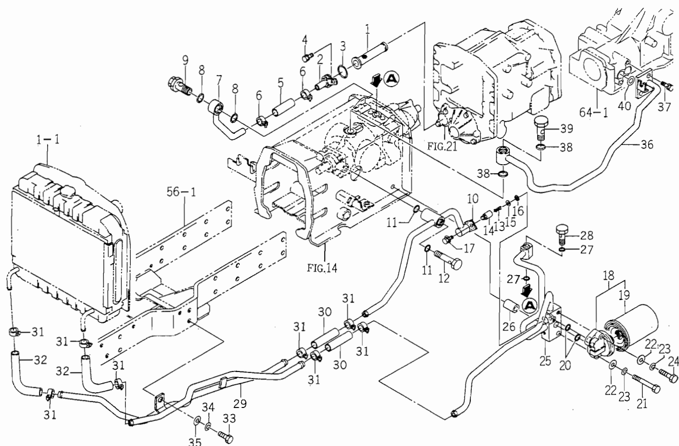
FIG. 40 PIPING (H.S.T.) SYSTEM
