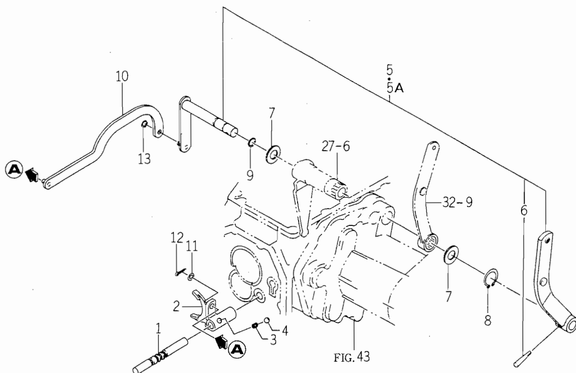
FIG. 20 SUB CHANGE (H.S.T.) SYSTEM
