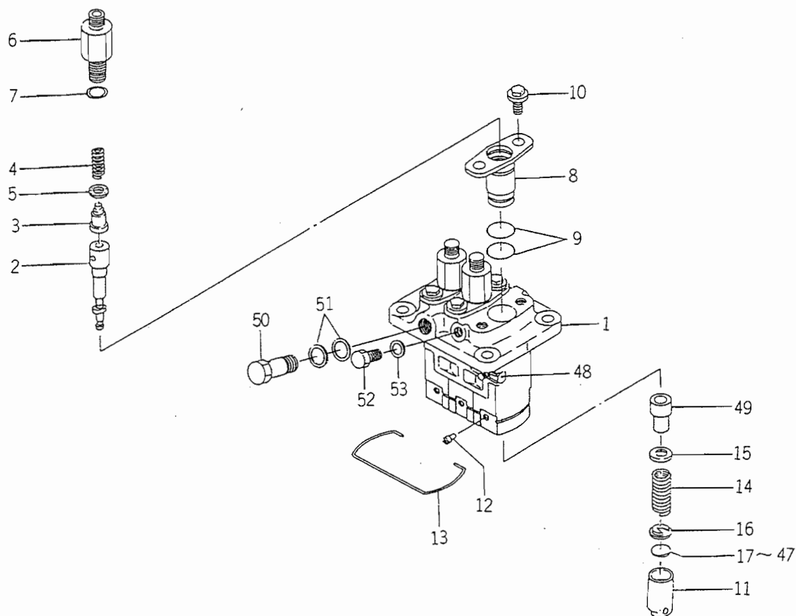
FIG. 25 6215 - 600 - 078 - 00
