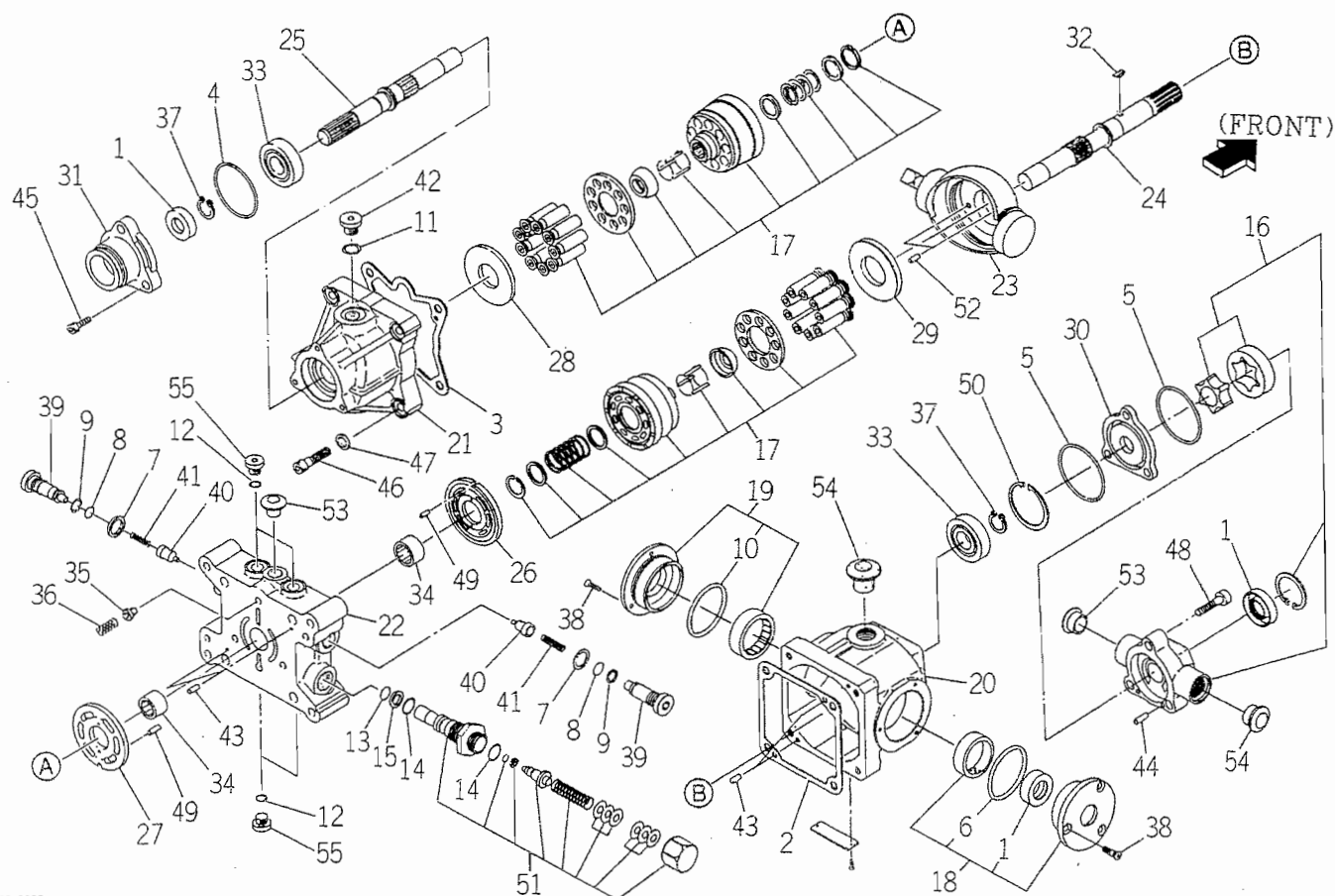
FIG.113 1622 - 202 - 500 - 00
