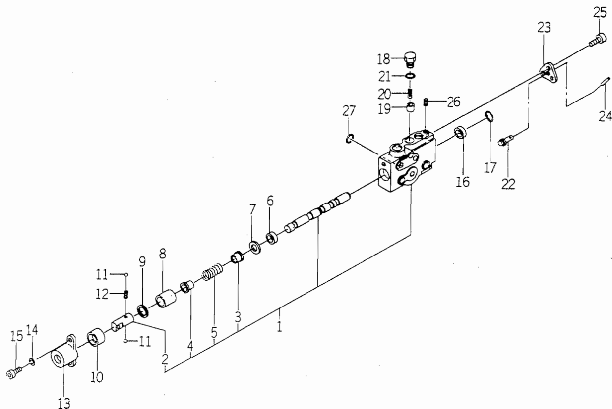
FIG.114 1640 - 530 - 600 - 00
