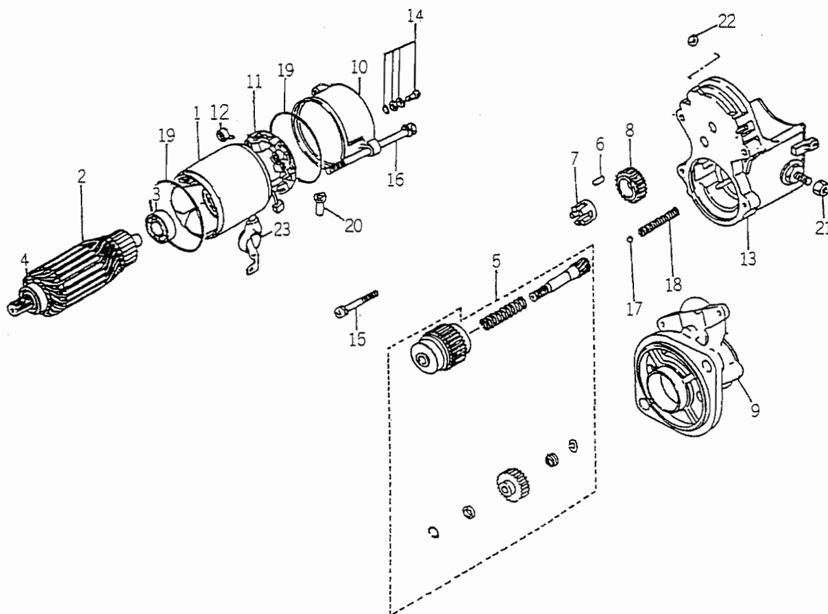
FIG. 26 6281-100-002-10
