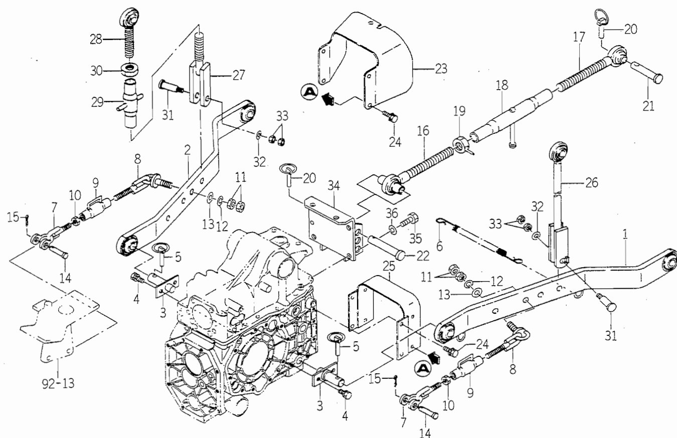
FIG. 83 3P LINK SYSTEM
