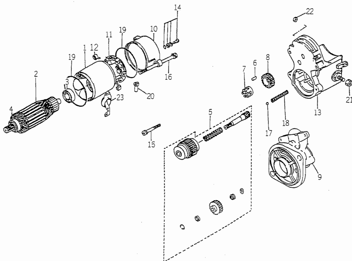
FIG. 26 6281 - 100 - 002 - 10
