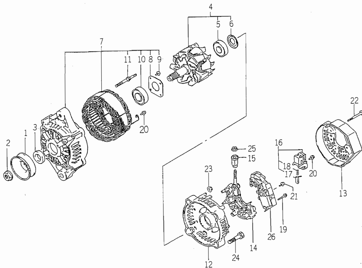
FIG. 27 6281 - 200 - 008 - 10
