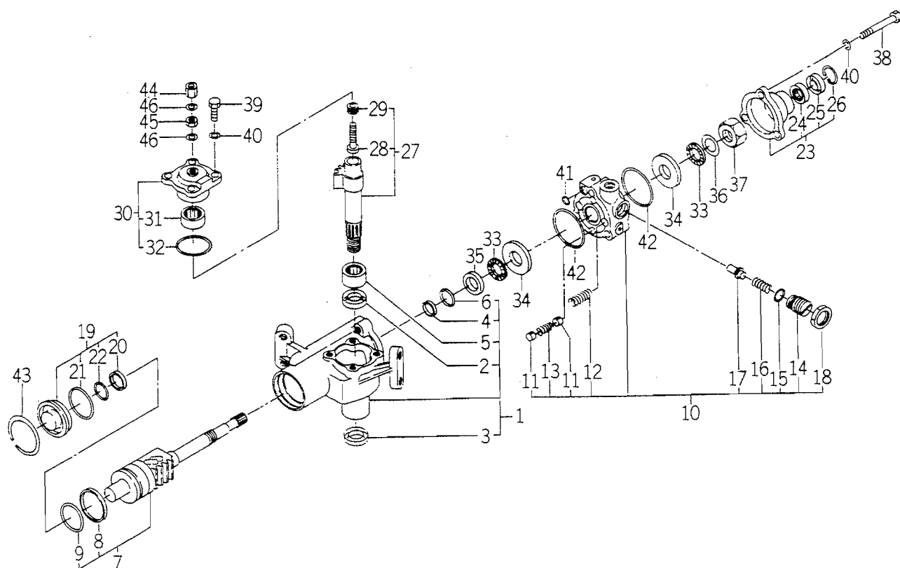
FIG.111 1614 - 407 - 210 - 00
