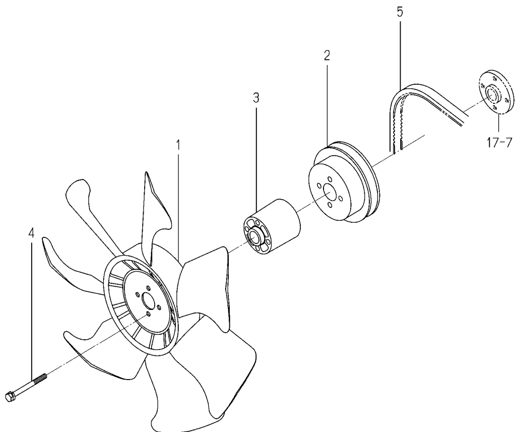
FIG. 18 COOLING FAN
