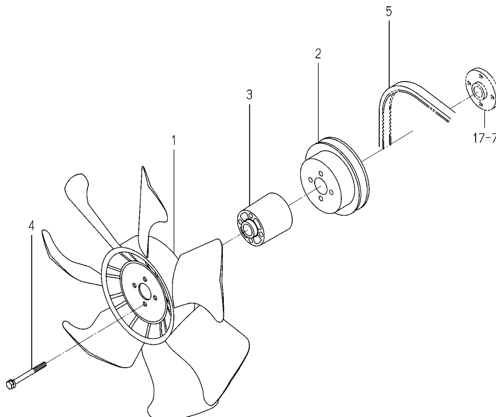
FIG. 18 COOLING FAN
