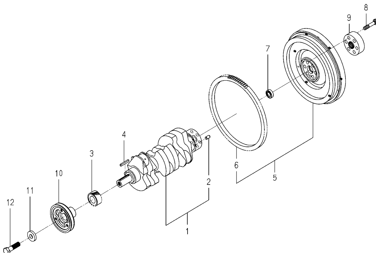
FIG. 15 CRANK SHAFT
