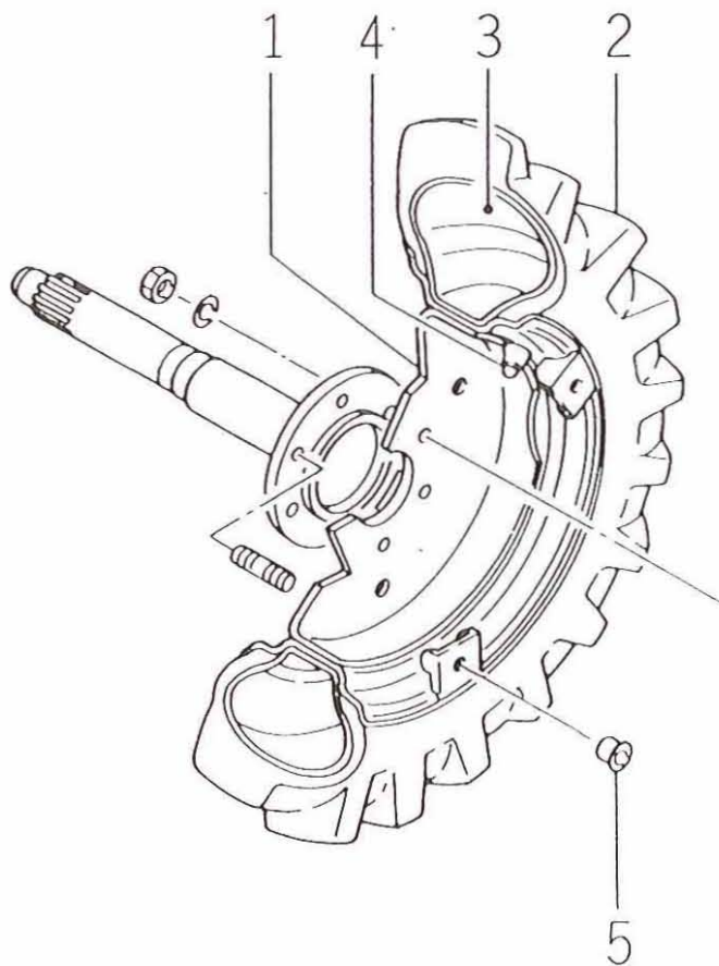
FIG. 52B TIRE
