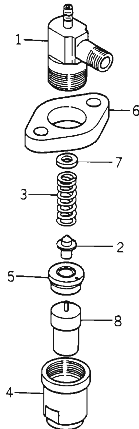
Fig. 8 NOZZLE AND NOZZLE HOLDER Injecteur et corps
