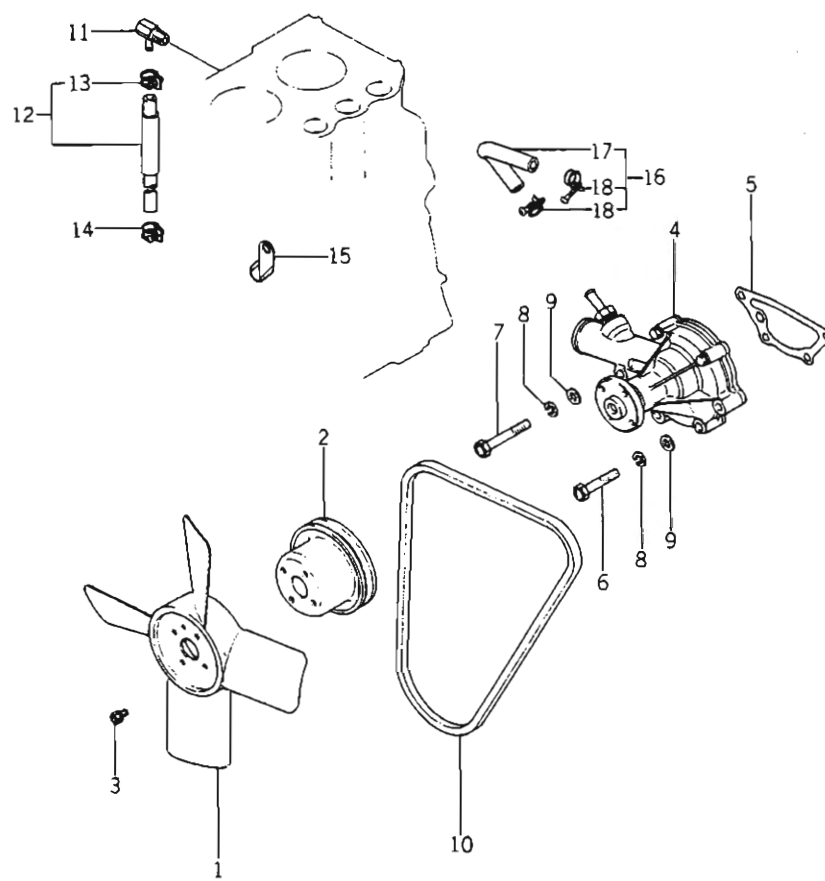
Fig. 12 COOLING PARTS GROUP Système de refroidissement
