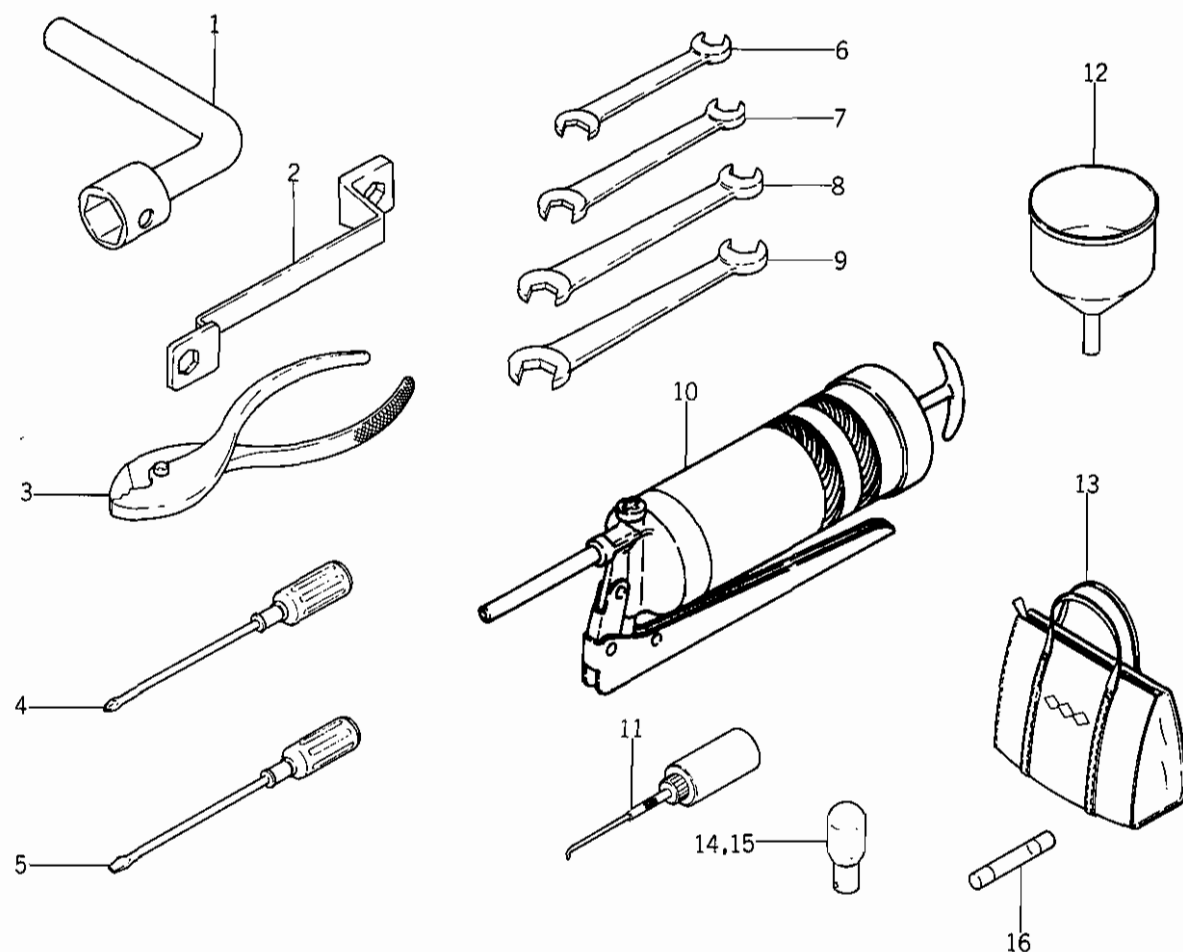
No. 37 工具及びトレーラヒッチ関係 Fig. 37 TOOLS AND TRAILER HITCH SYSTEM
