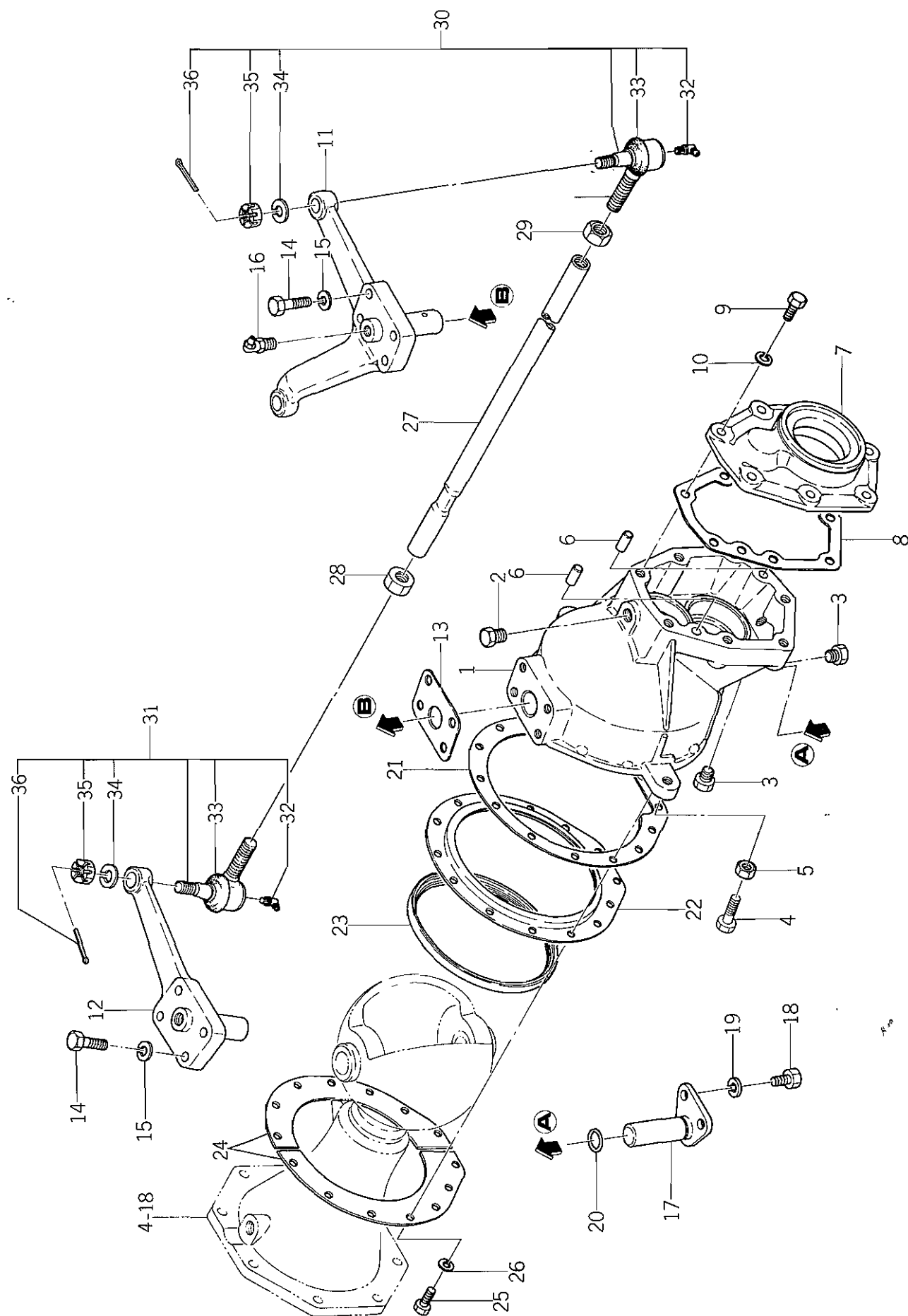
No. 5 フロントアクスルケース及びナックルアーム関係 (F型用) Fig. 5 FRONT AXLE CASE AND KNUCKLE ARM SYSTEM
