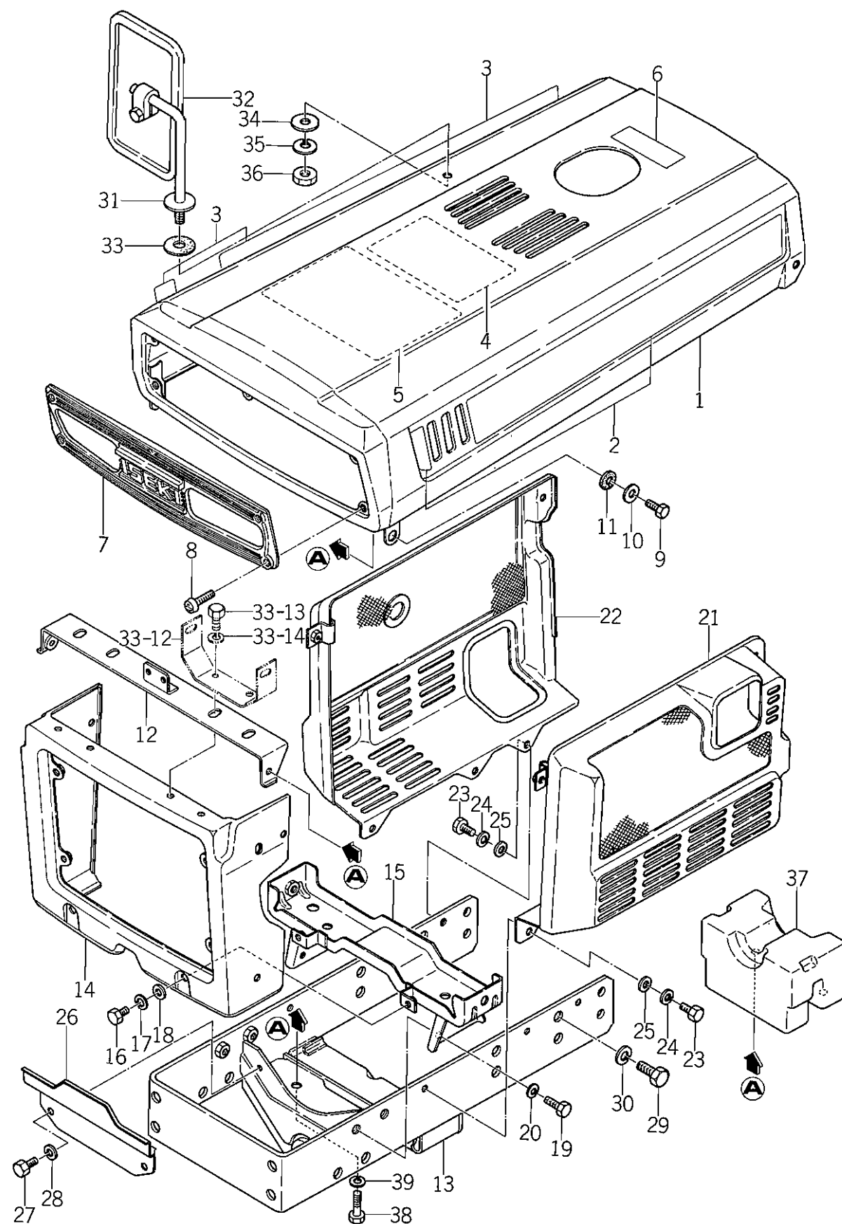
No. 3 ボンネット及びフレーム関係 Fig. 3 BONNET AND FRAME SYSTEM
