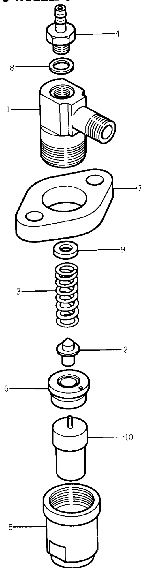
No. 8 ノズルアンドノズルホルダ Fig. 8 NOZZLE & NOZZLE HOLDER
