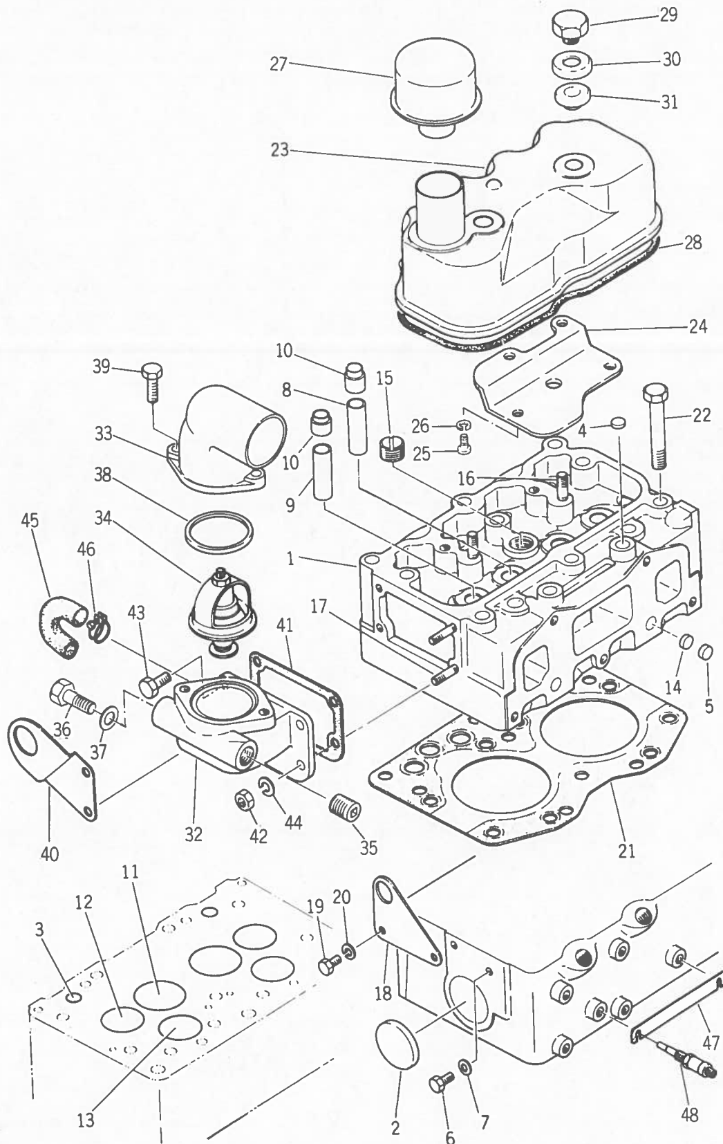
No. 1 シリンダ Fig. 1 CYLINDER
