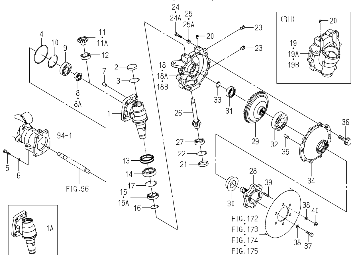
FIG. 95 GEAR(FINAL)SYSTEM
