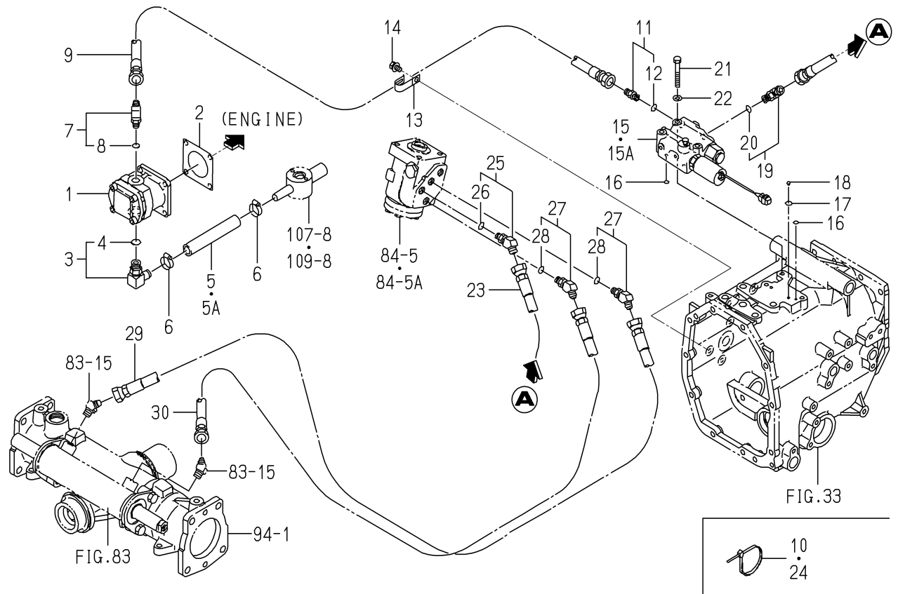
FIG. 86 PIPING(SUB)SYSTEM(H TYPE)
