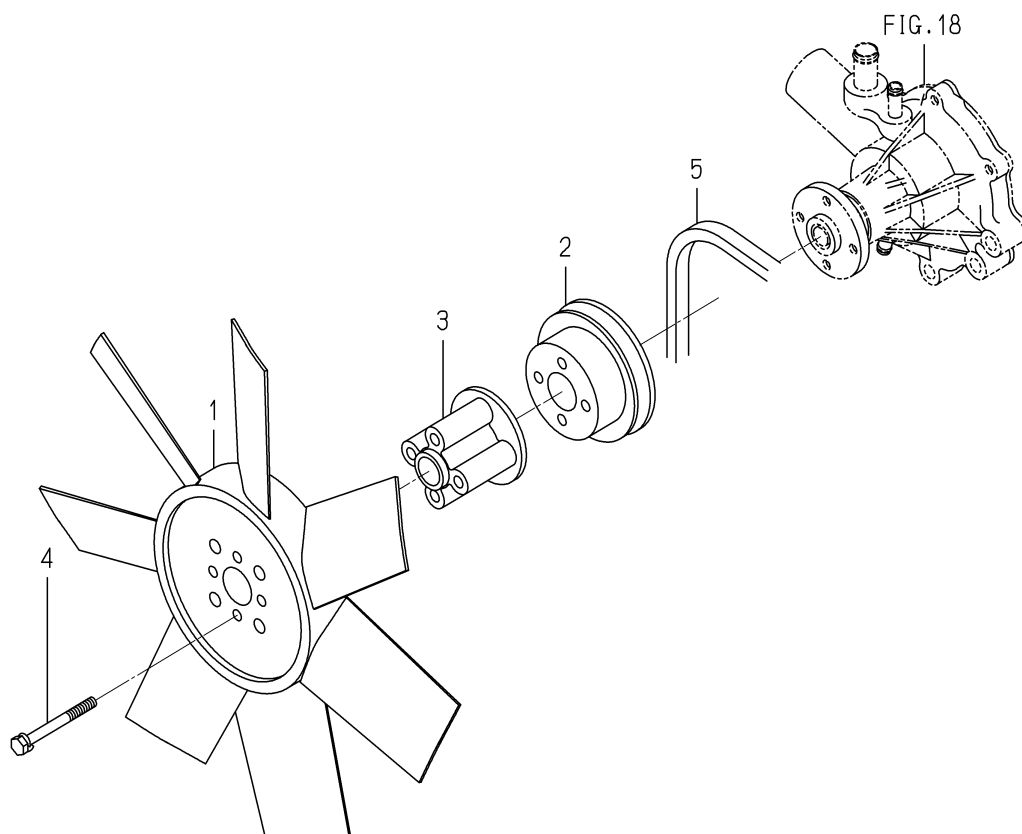
FIG. 19 COOLING FAN
