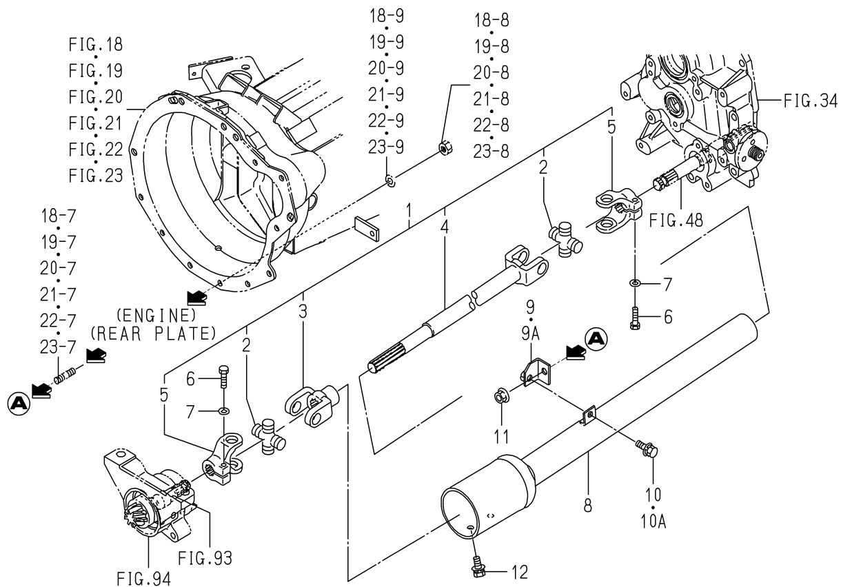
FIG. 92 SHAFT(4WD)SYSTEM
