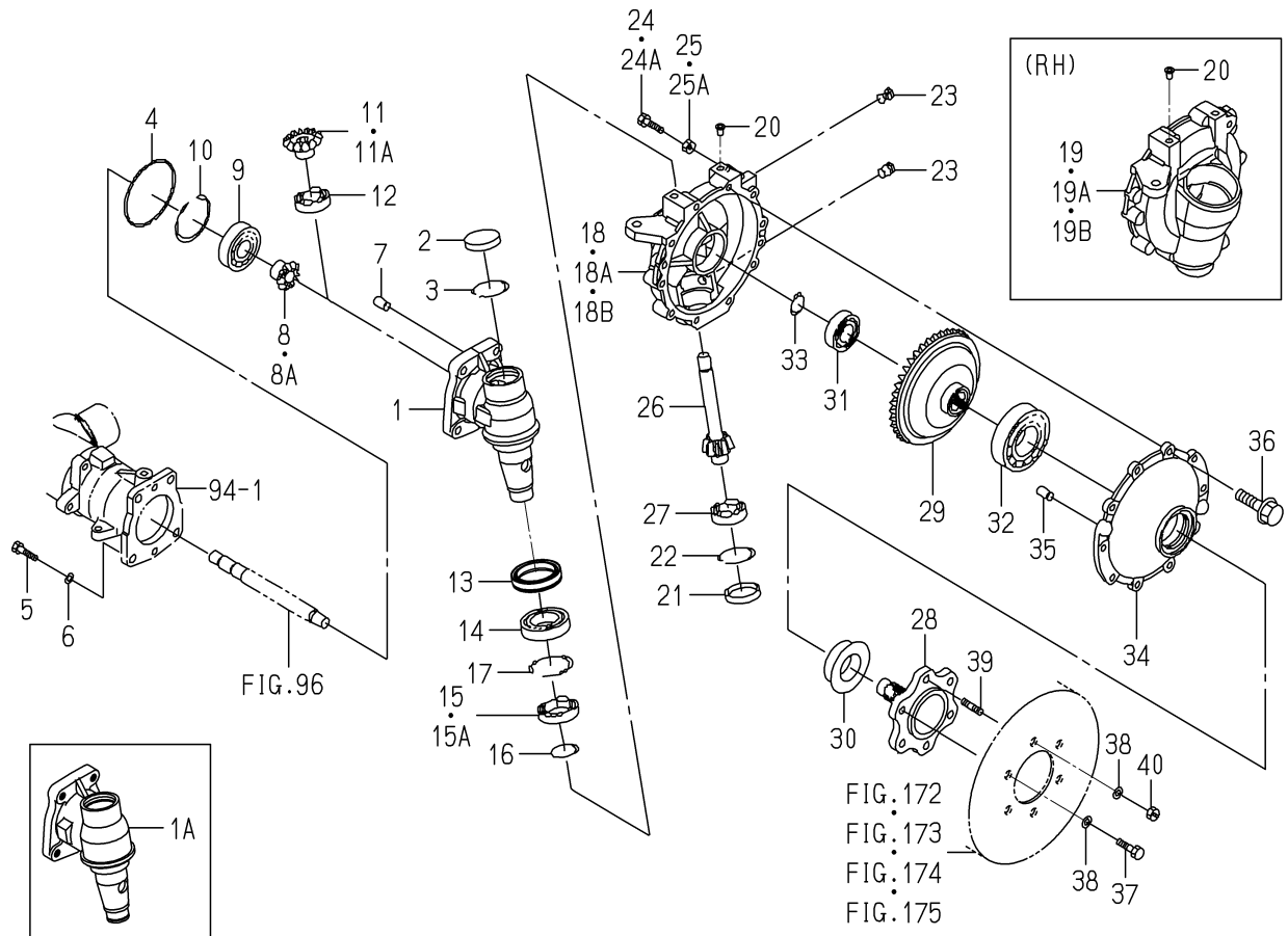
FIG. 95 GEAR(FINAL)SYSTEM
