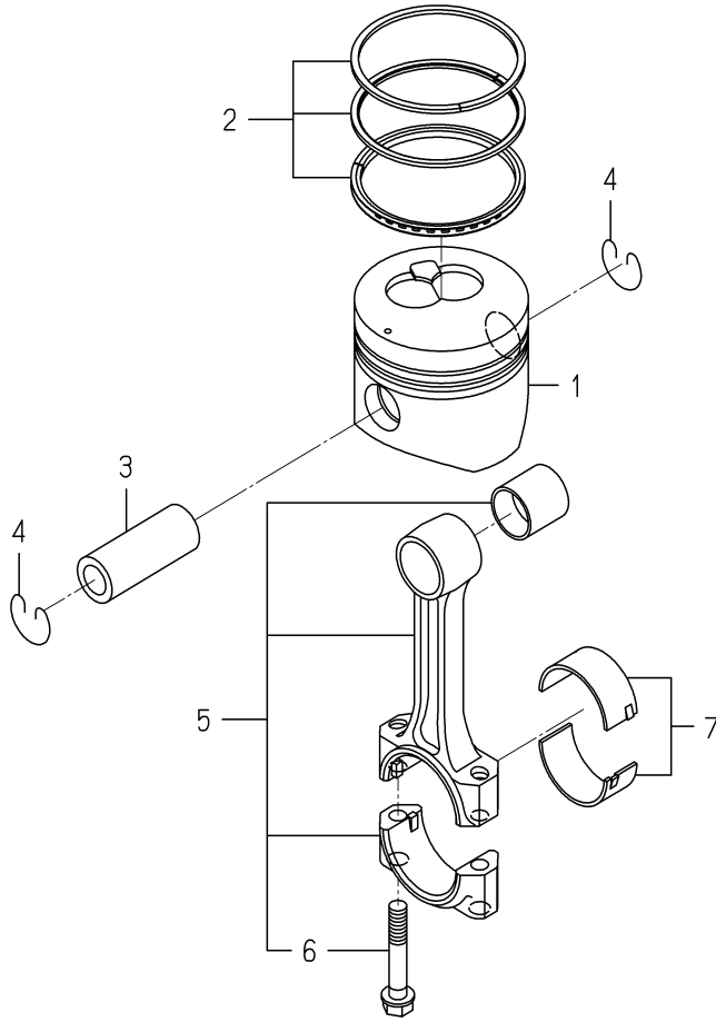
FIG. 14 PISTON
