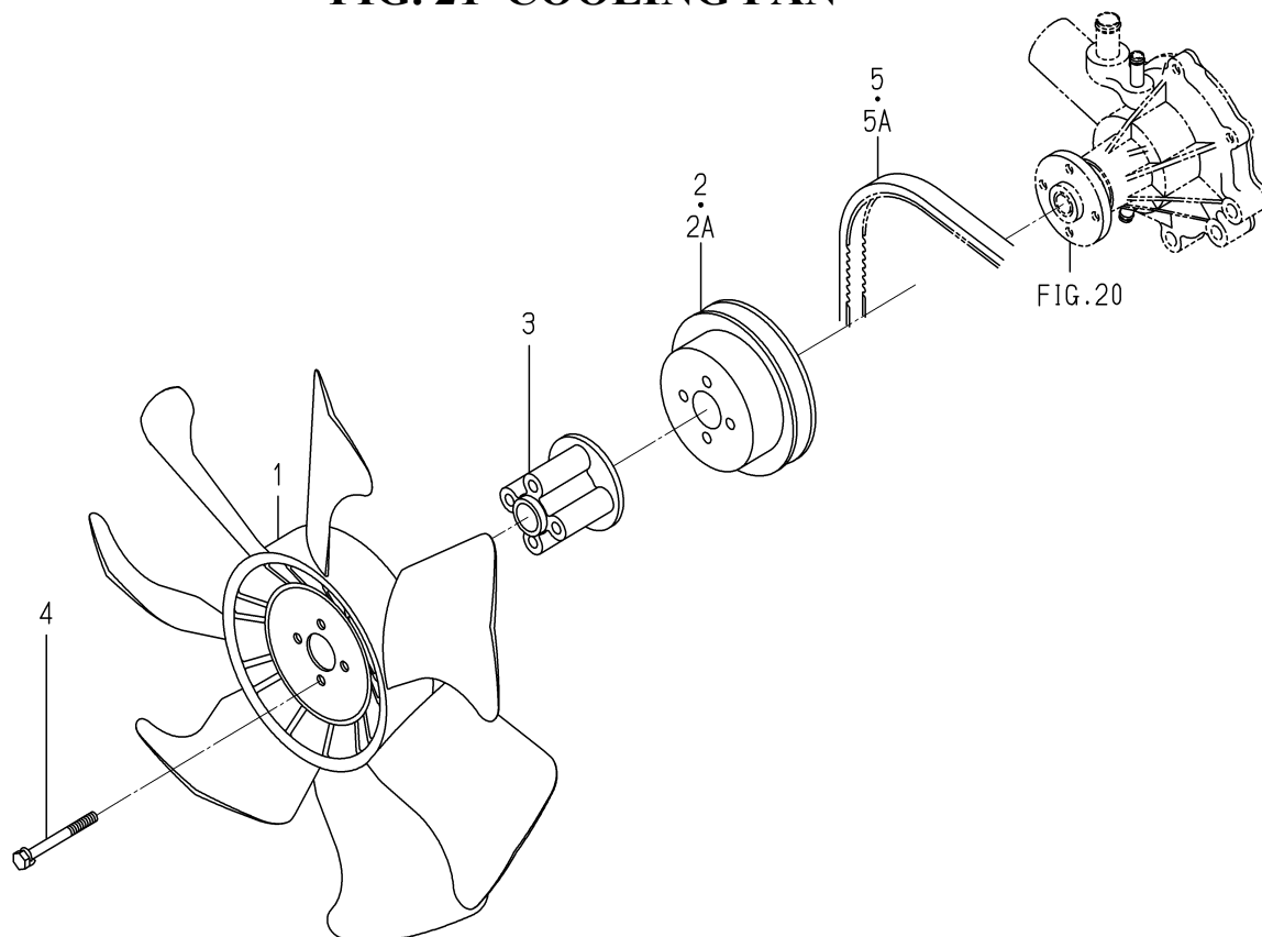
FIG. 21 COOLING FAN
