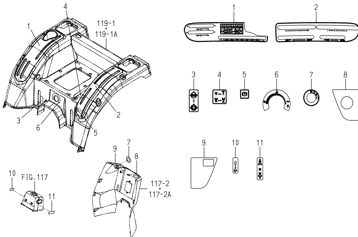
FIG.157 LABEL(CONTROL) (V,W TYPE EXCEPT H)
