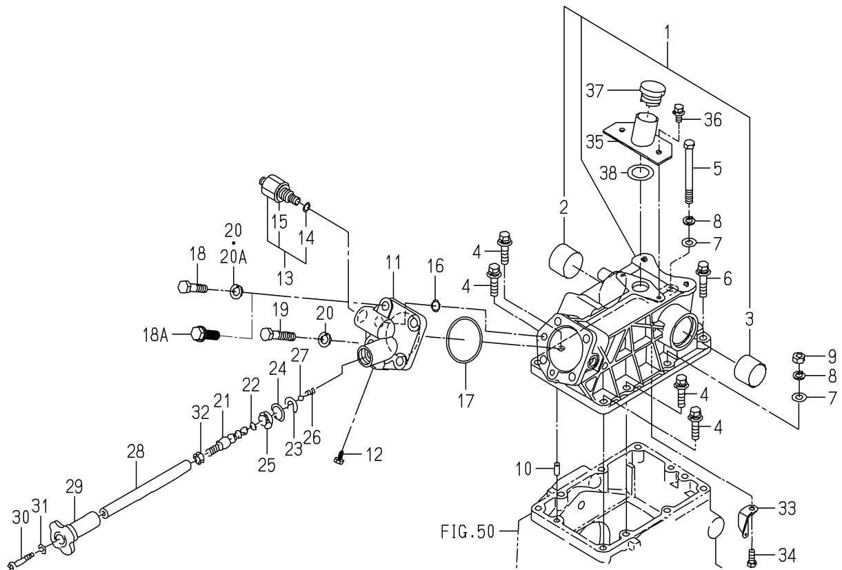
FIG. 98 CASE(CYLINDER)SYSTEM
