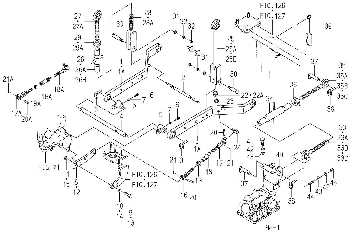
FIG.110 LINK(3P)SYSTEM (D TYPE-3215-NO.1907-, 3245-NO.390-,3265-NO.1090-)
