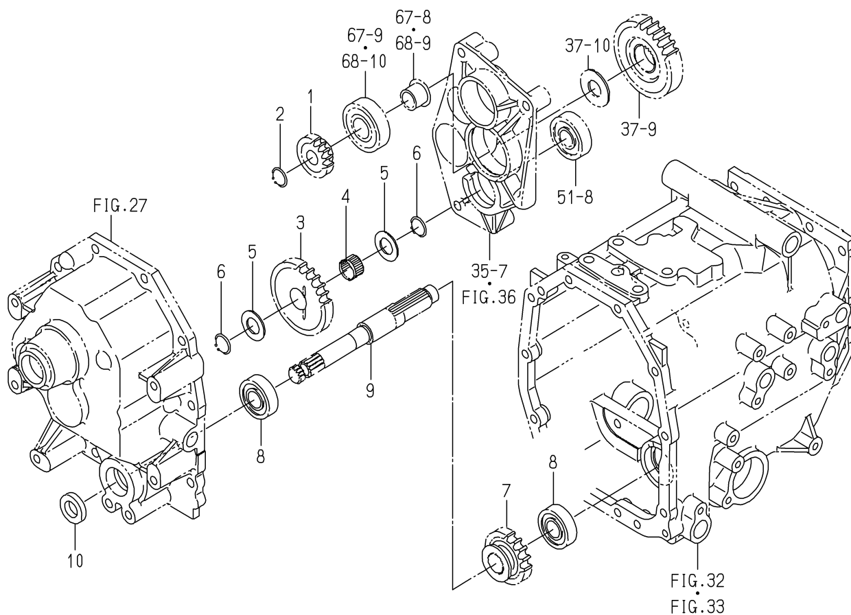
FIG. 48 GEAR(4WD)SYSTEM
