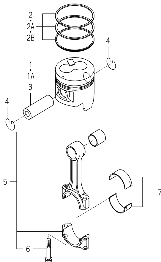
FIG. 16 PISTON
