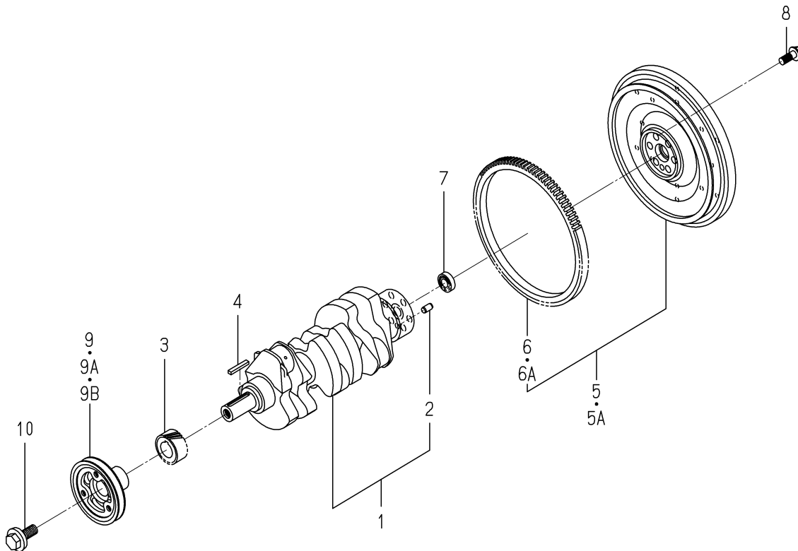
FIG. 18 CRANK SHAFT
