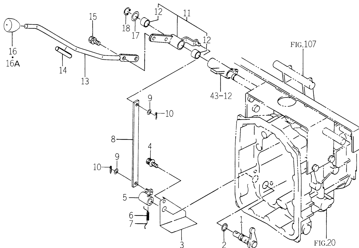
FIG. 31 LEVER (SUB) SYSTEM (H TYPE-TM3200H-No.1-270/TM3240H-No.1-233)
