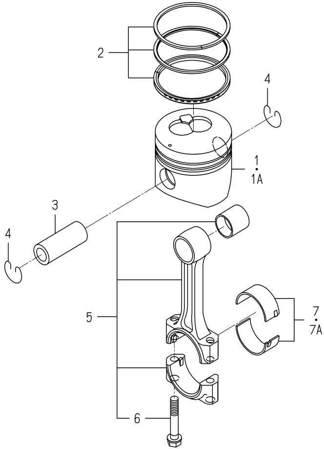
FIG. 15 PISTON
