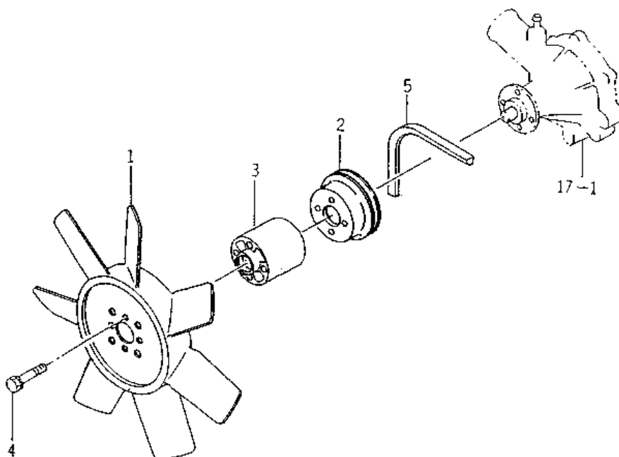
FIG. 18 COOLING FAN
