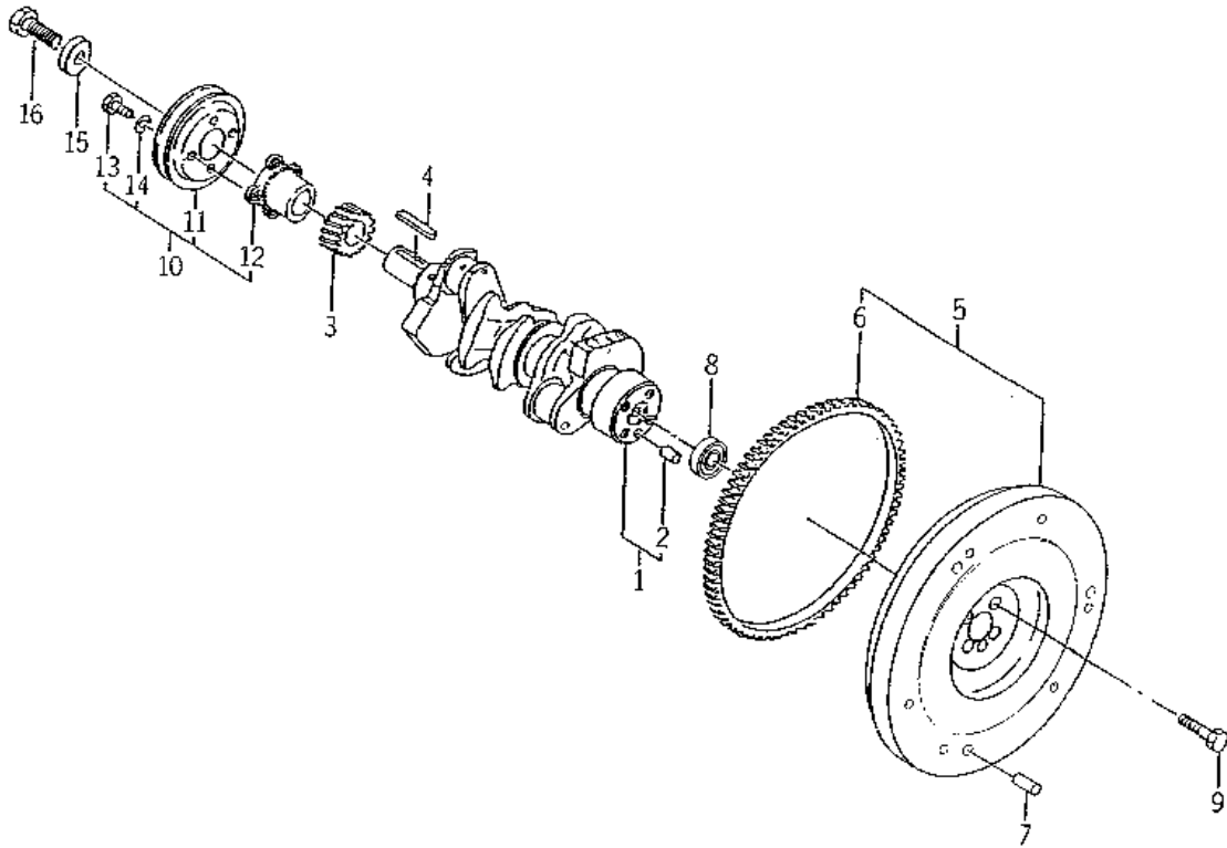
FIG. 15 CRANK SHAFT
