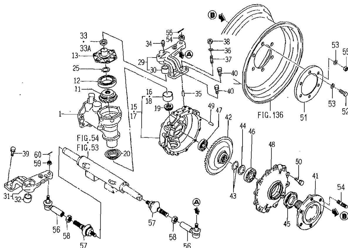
FIG. 59 CASE (GEAR/FRONT),TIE ROD SYSTEM(2/2)
