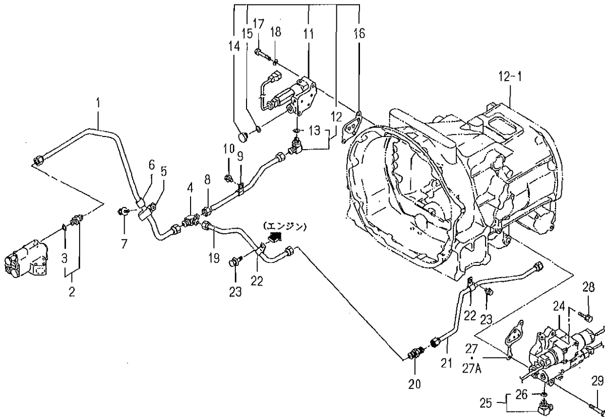
FIG. 76 PIPING (SUB) SYSTEM (P TYPE)
