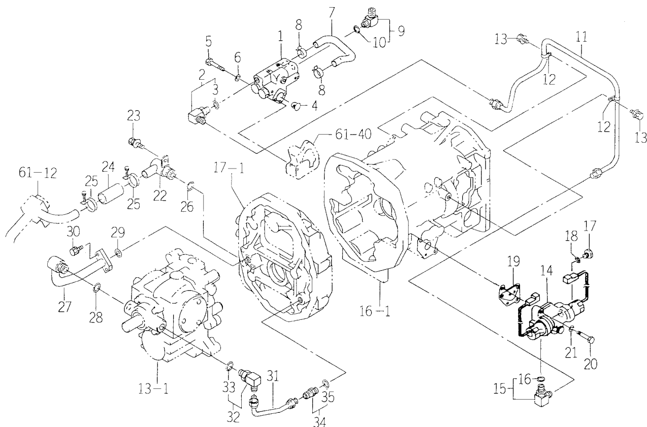
FIG. 62 PIPING (SUB) SYSTEM
