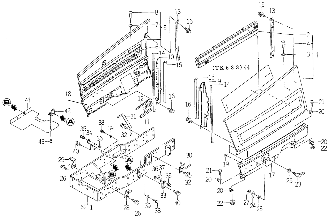
FIG. 88 FAN COVER SYSTEM
