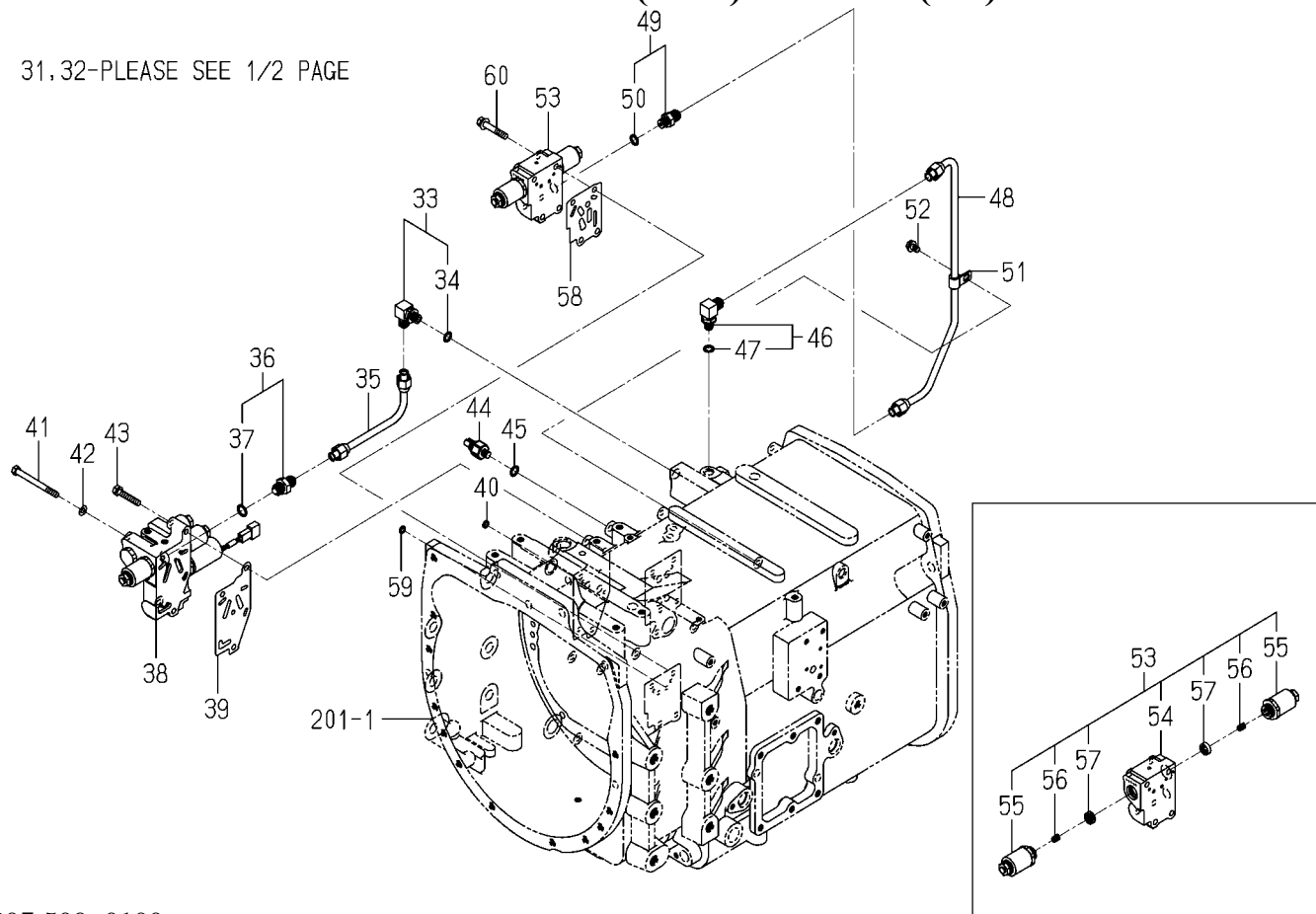
FIG.504 PIPING(SUB)SYSTEM(2/2)
