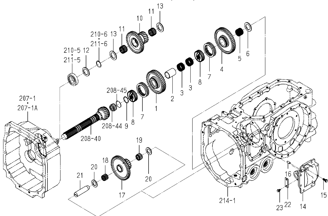
FIG.209 GEAR(SUB)SYSTEM
