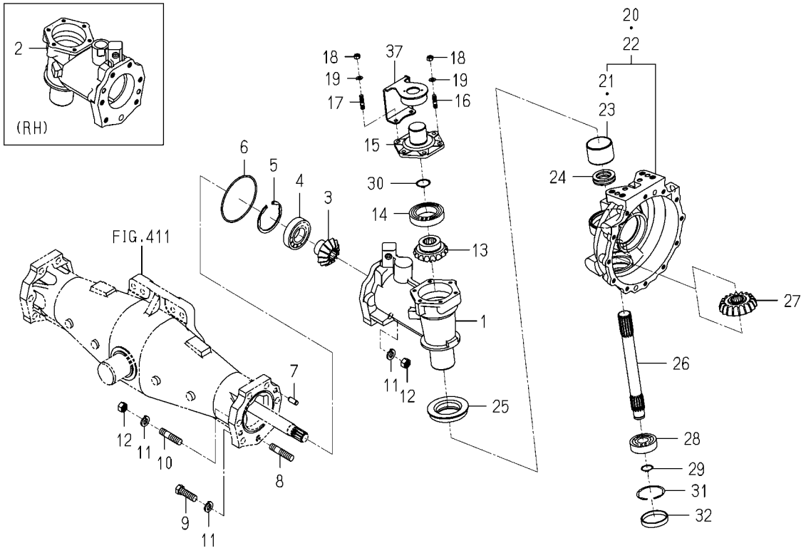
FIG.414 CASE(1/2) (GEAR/FINAL/FRONT)SYSTEM (8080)
