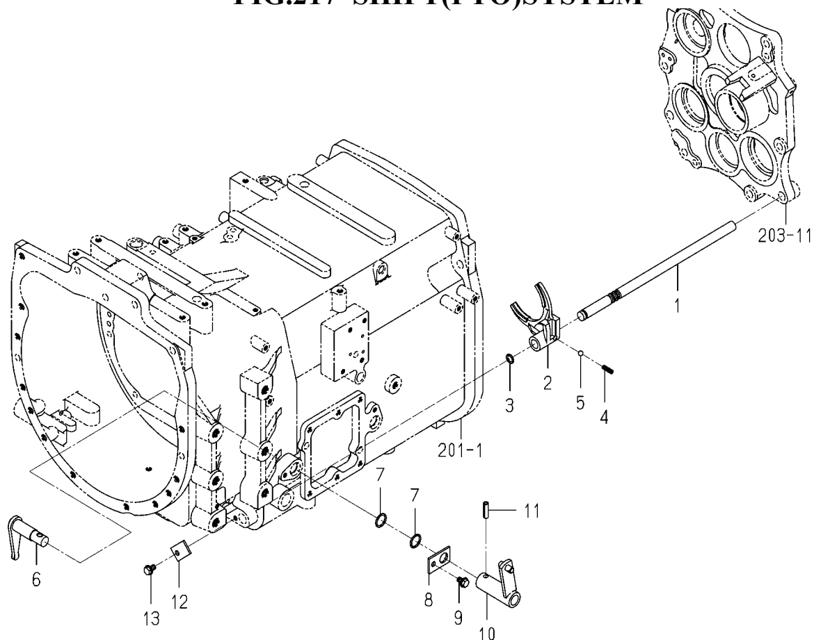
FIG.217 SHIFT(PTO)SYSTEM
