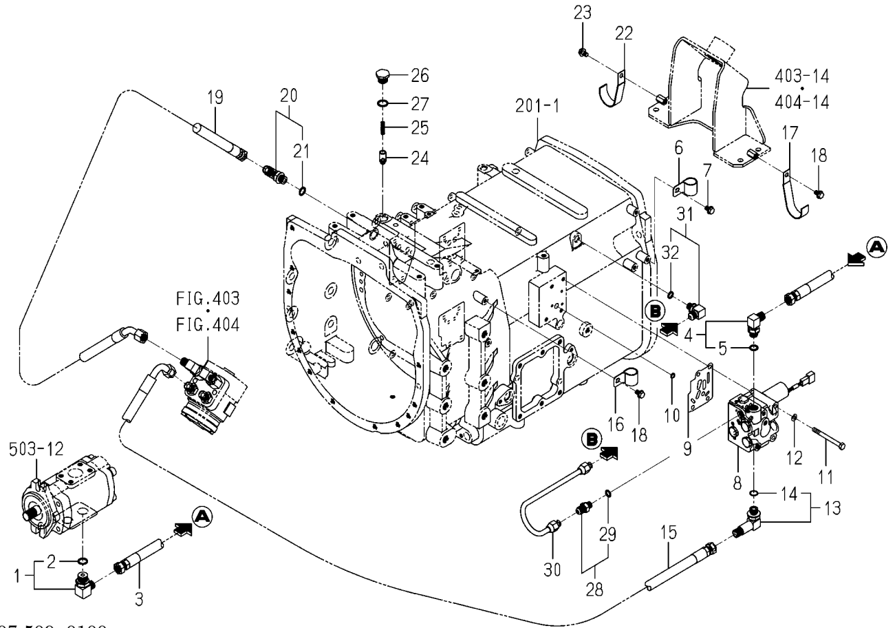
FIG.504 PIPING(SUB)SYSTEM(1/2)
