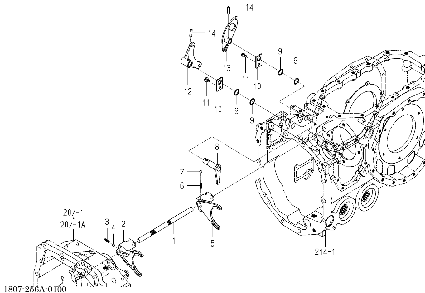
FIG.216 SHIFT(SUB)SYSTEM
