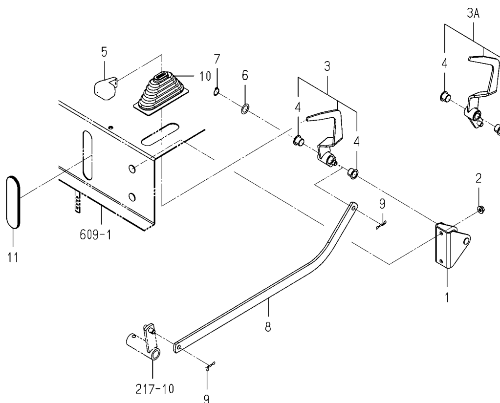
FIG.221 LEVER(PTO)SYSTEM
