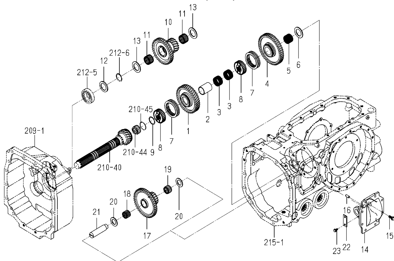
FIG.211 GEAR(SUB)SYSTEM
