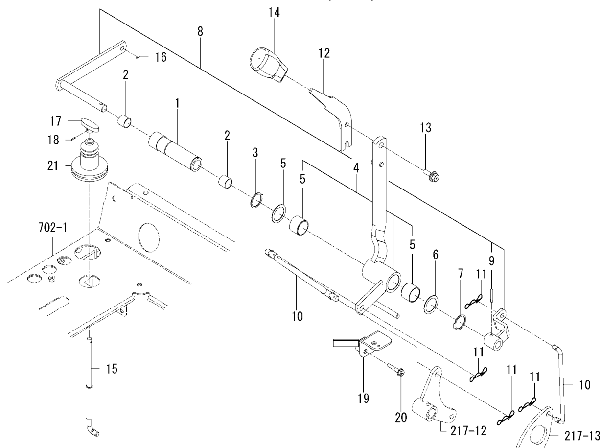
FIG.222 LEVER(SUB)SYSTEM
