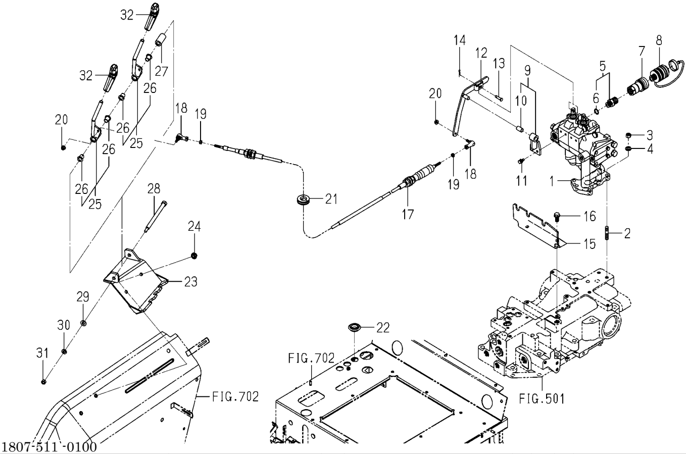
FIG.508 VALVE(REMOTE)SYSTEM
