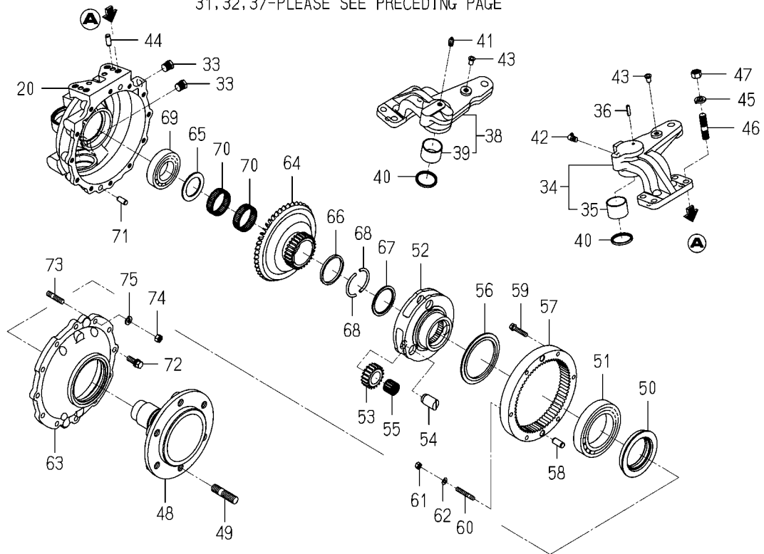
FIG.414 CASE(2/2) (GEAR/FINAL/FRONT)SYSTEM(8080)
