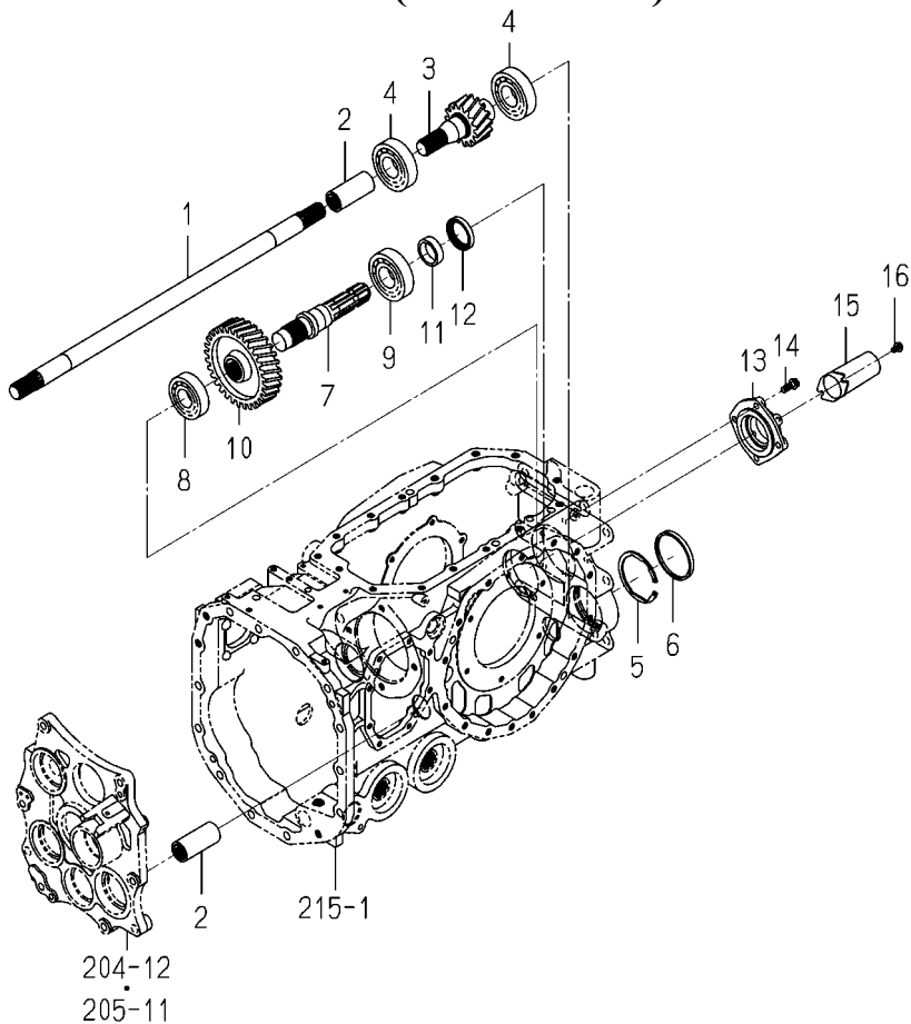
FIG.214 GEAR(PTO/REAR)SYSTEM
