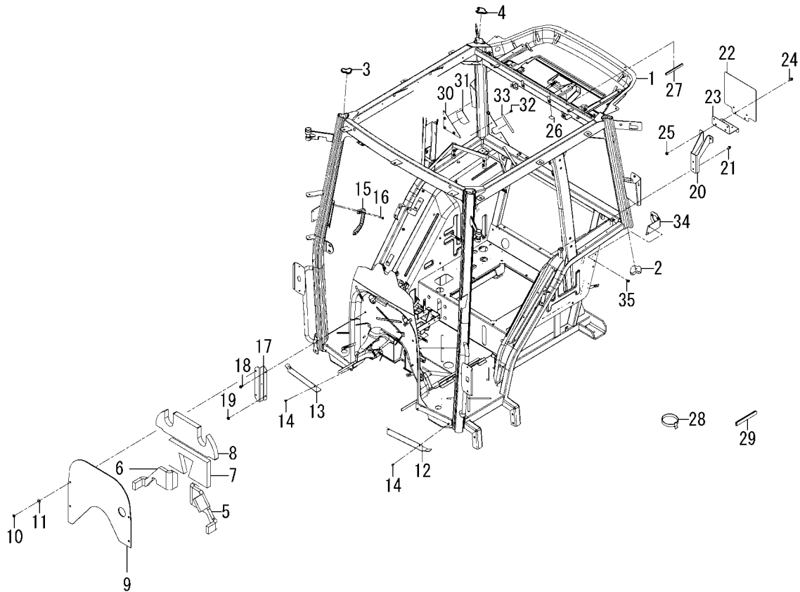
FIG.702 FRAME(CABIN)SYSTEM
