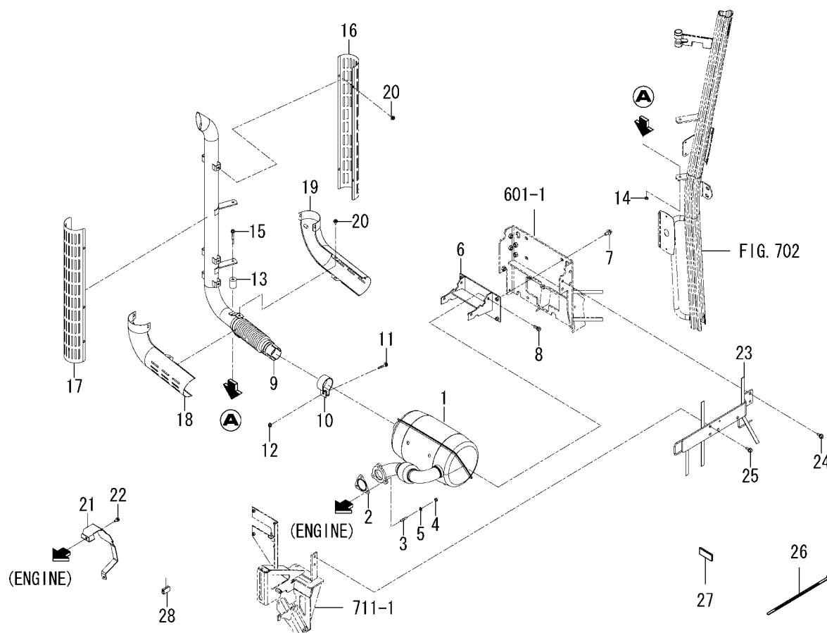
FIG.102 MUFLER SYSTEM
