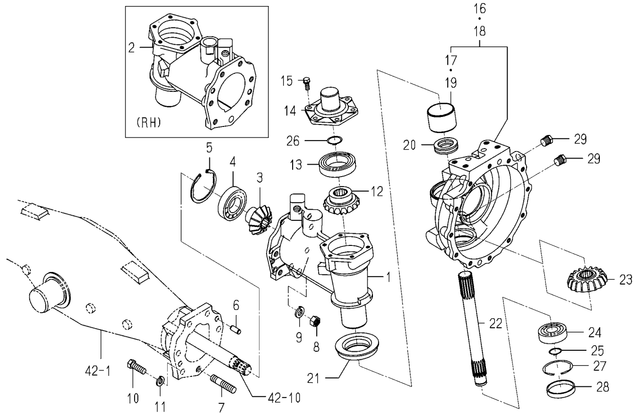
FIG. 43 CASE (GEAR/FRONT) SYSTEM(1/3)
