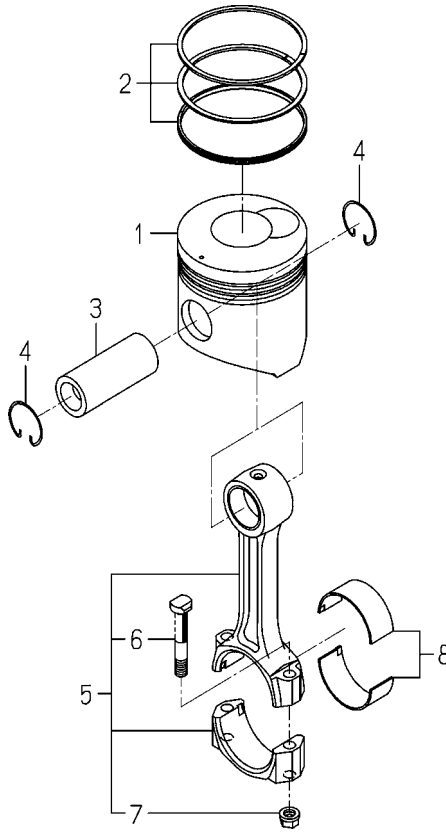
FIG. 14 PISTON
