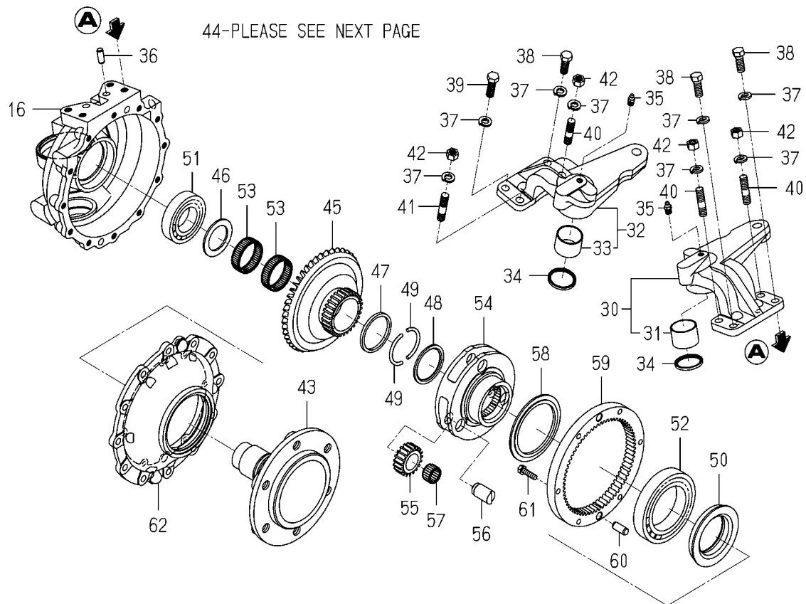
FIG. 43 CASE (GEAR/FRONT) SYSTEM(2/3)
