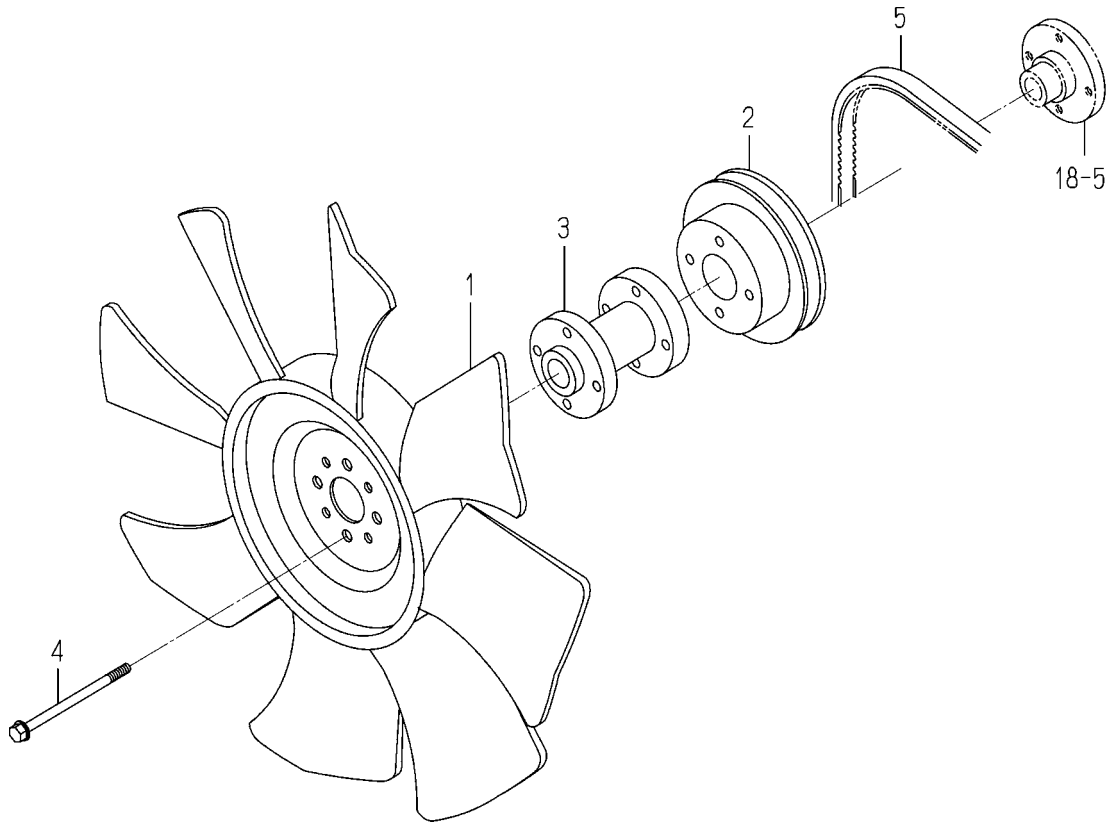
FIG. 19 COOLING FAN
