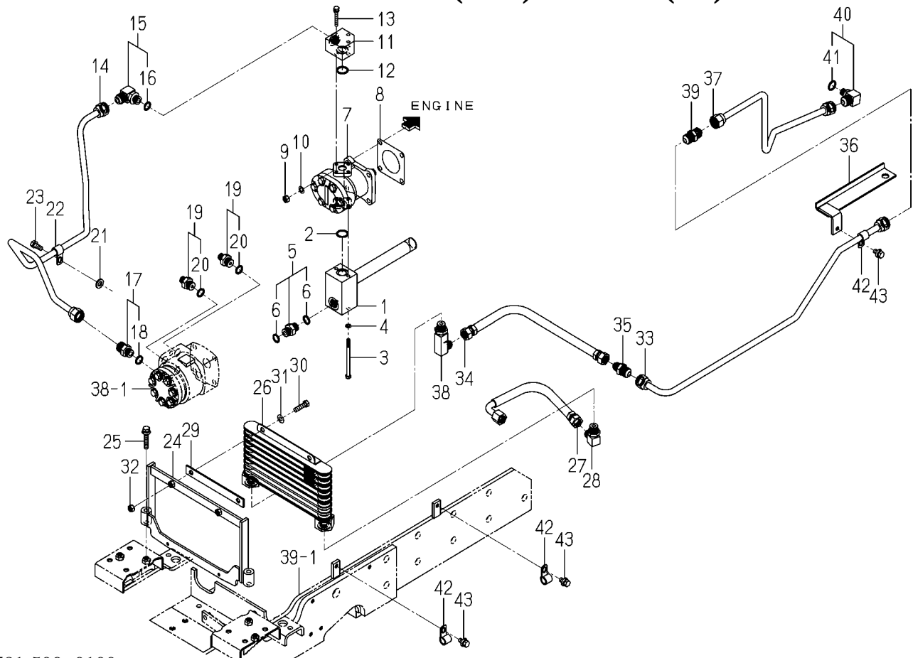
FIG. 49 PIPING (SUB) SYSTEM(1/4)
