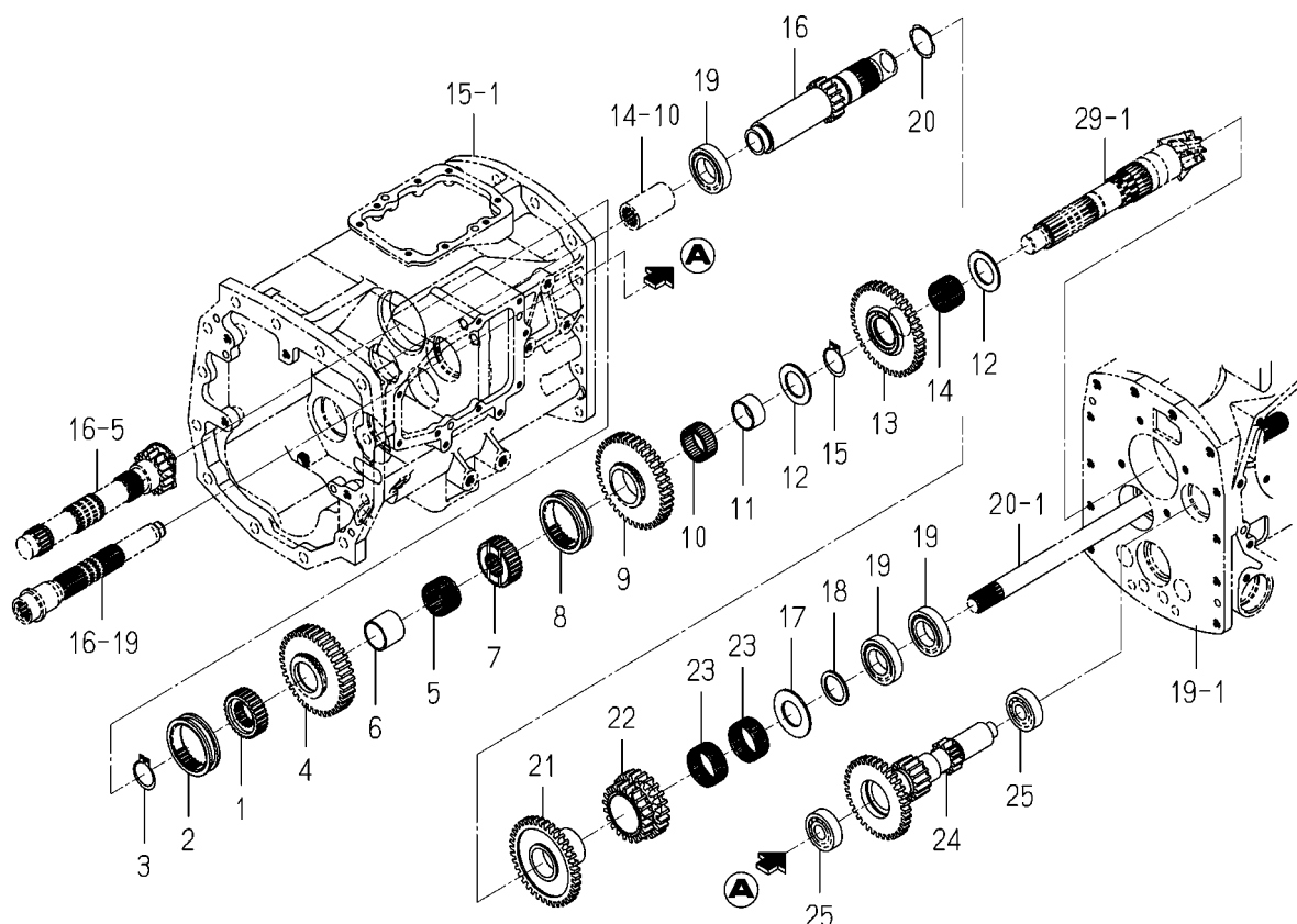
FIG. 17 GEAR (SUB) SYSTEM
