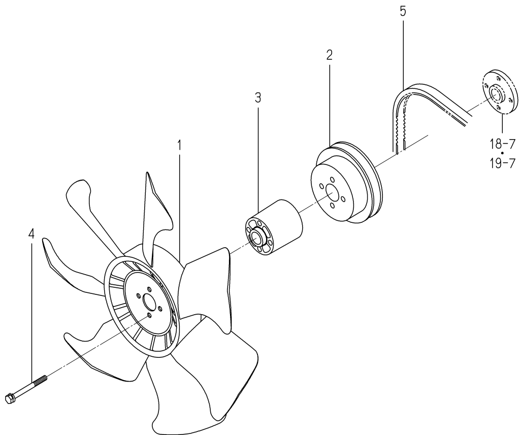
FIG. 20 COOLING FAN
