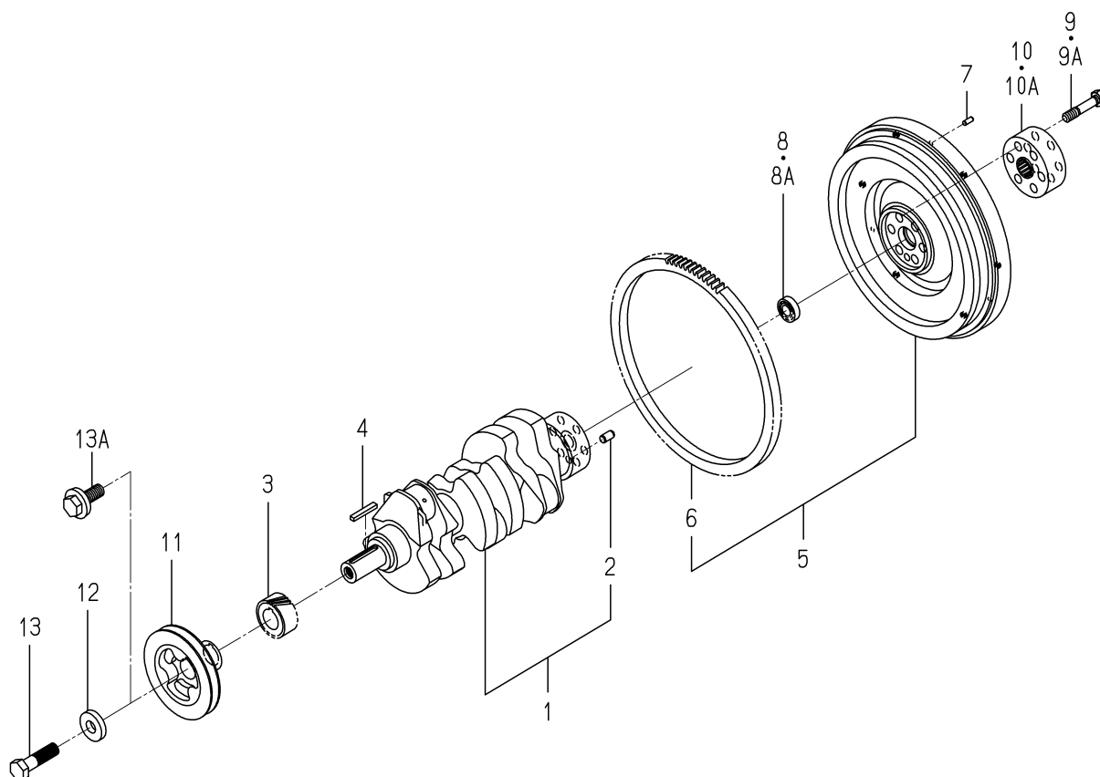
FIG. 20 CRANK SHAFT
