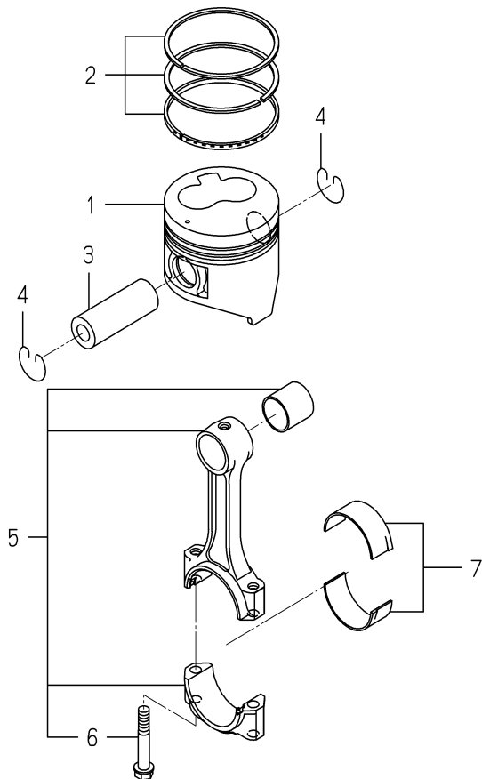
FIG. 14 PISTON
