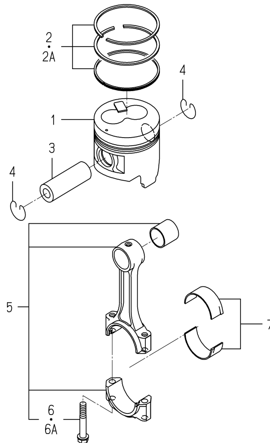
FIG. 17 PISTON
