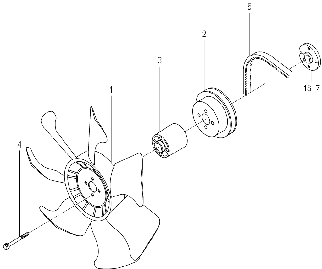
FIG. 19 COOLING FAN
