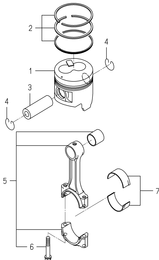
FIG. 14 PISTON
