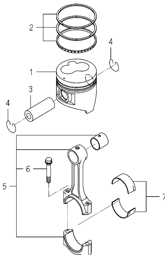
FIG. 13 PISTON
