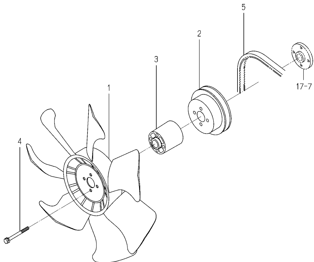
FIG. 18 COOLING FAN
