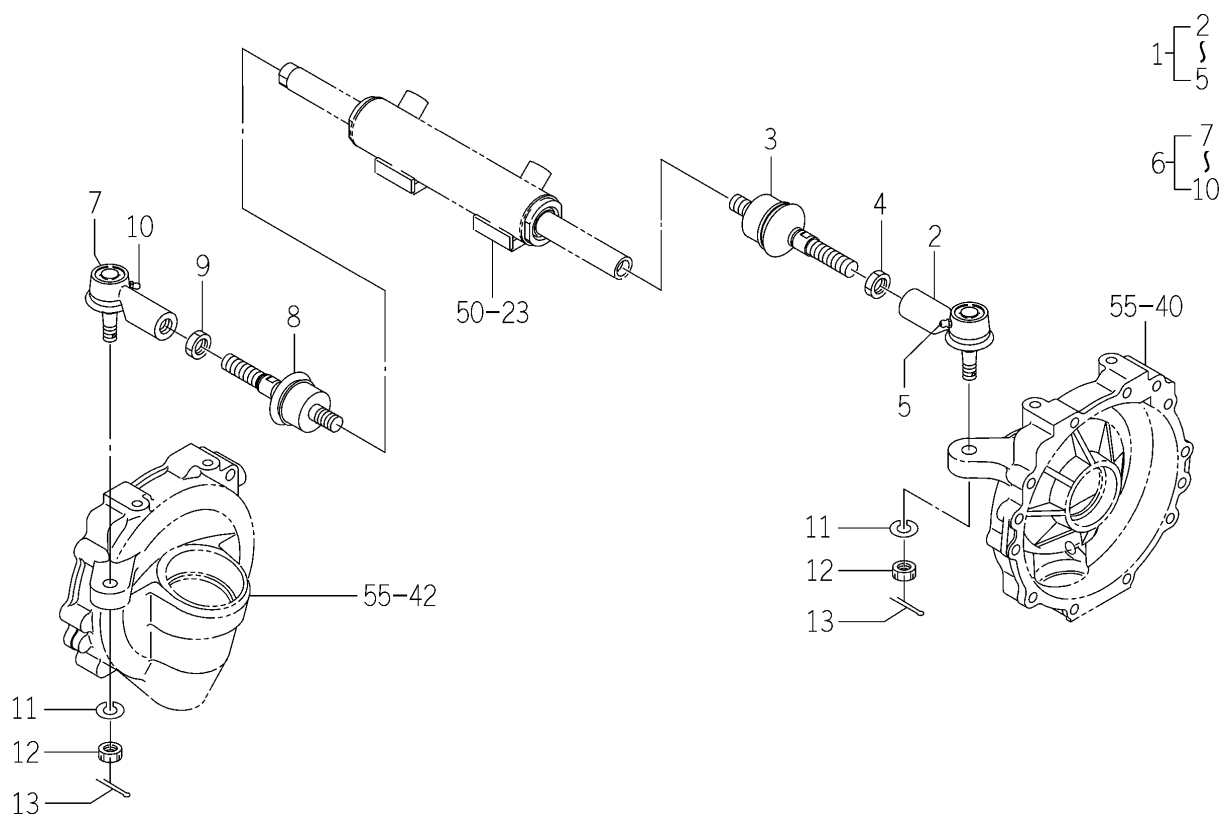
FIG. 59 TIE ROD SYSTEM (V TYPE)
