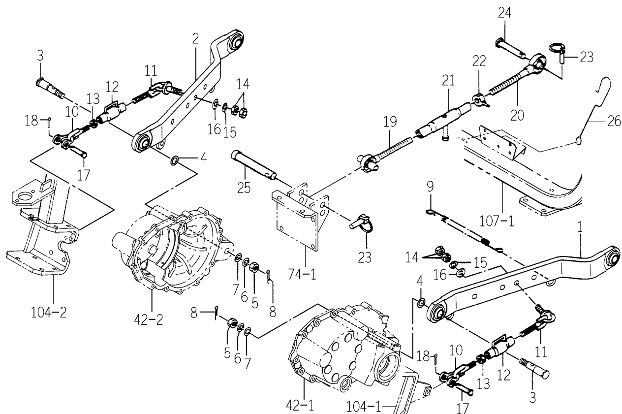
FIG. 72 3P LINK SYSTEM
