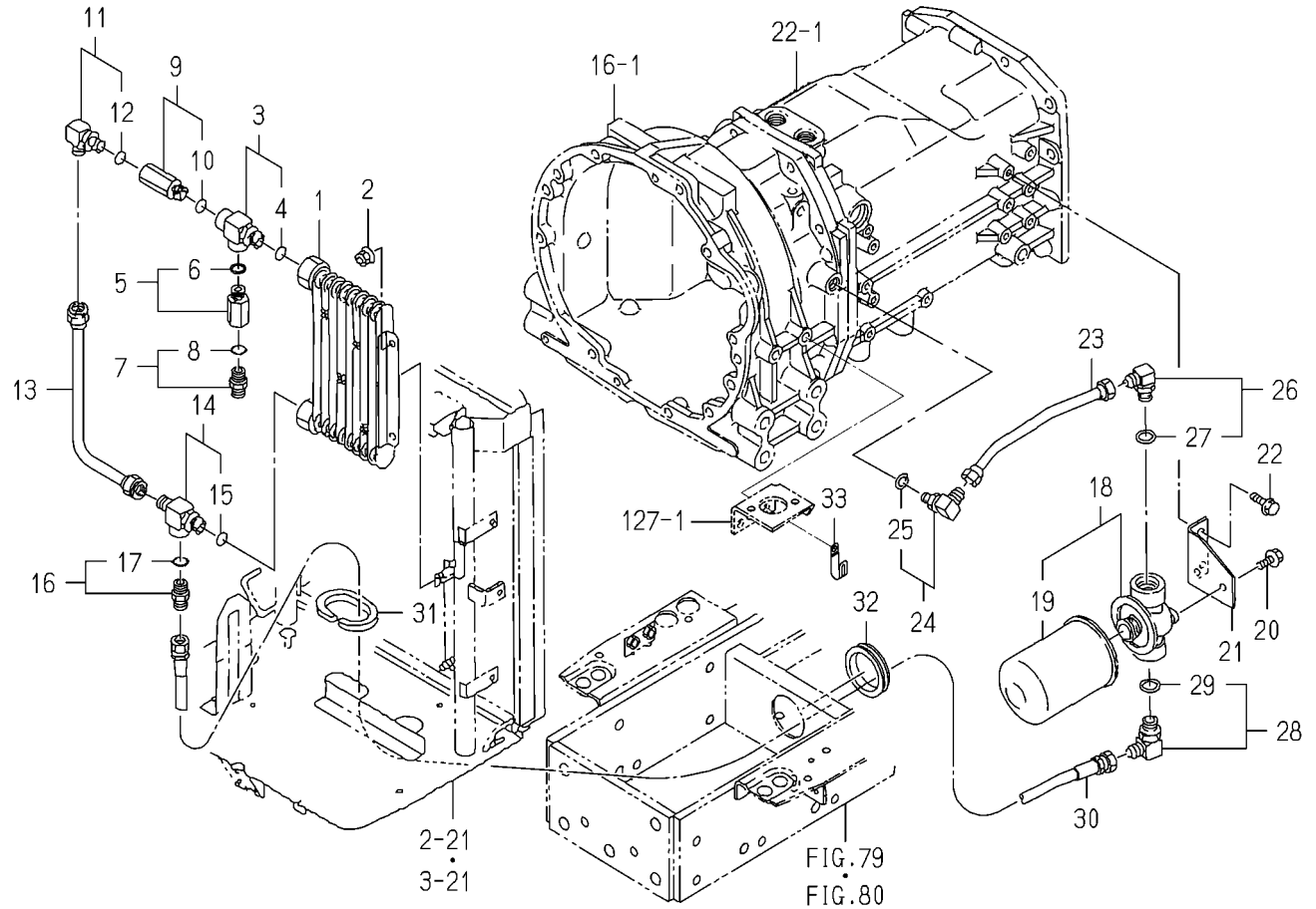
FIG.105 PIPING(SUB)SYSTEM(H TYPE)
