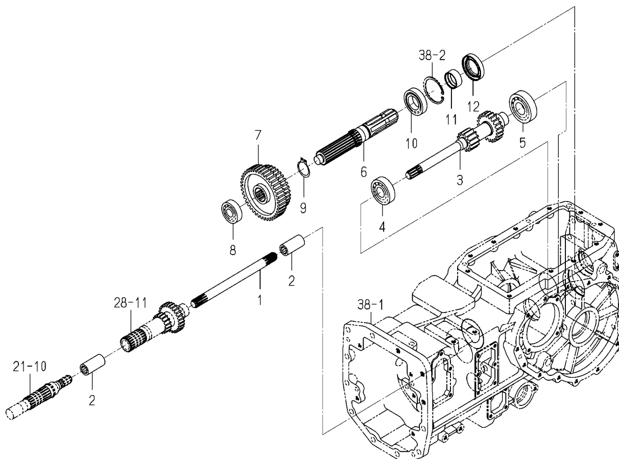
FIG. 33 GEAR(PTO)SYSTEM(H TYPE)
