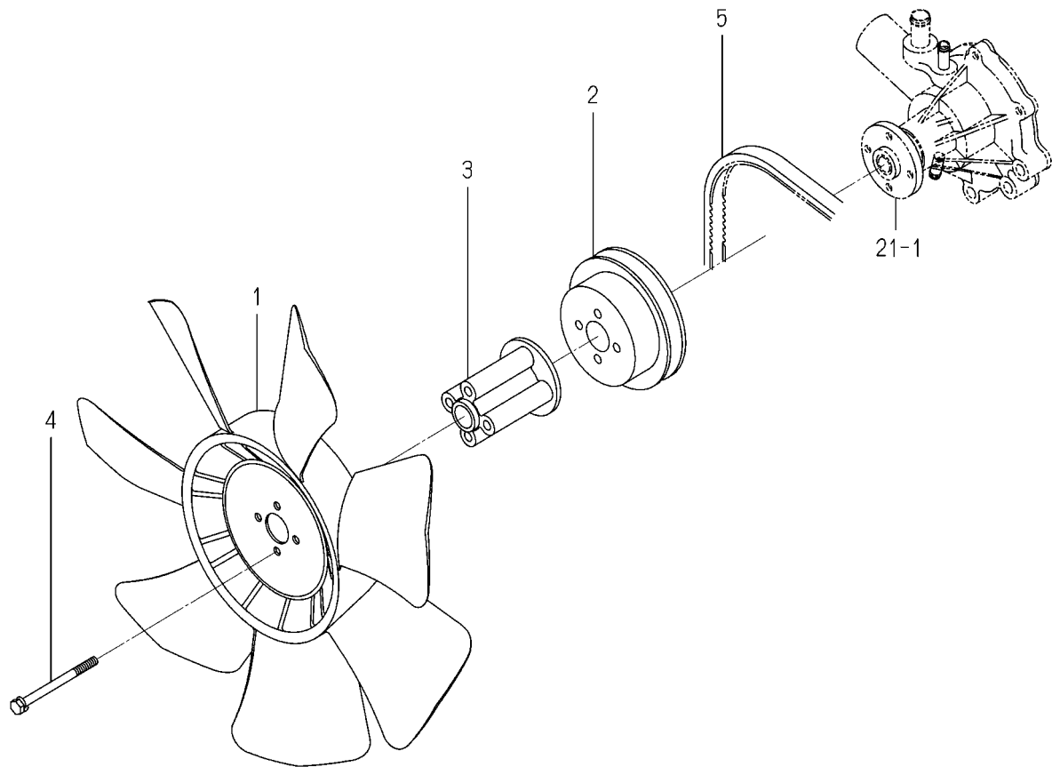
FIG. 23 COOLING FAN
