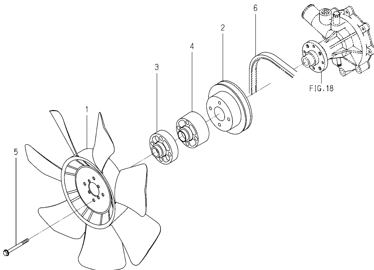
FIG. 19 COOLING FAN
