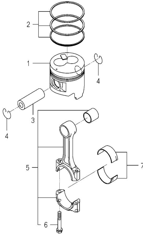
FIG. 15 PISTON
