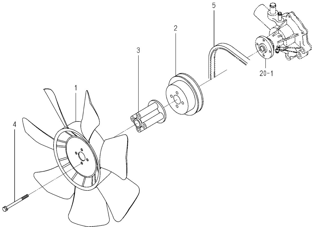
FIG. 21 COOLING FAN
