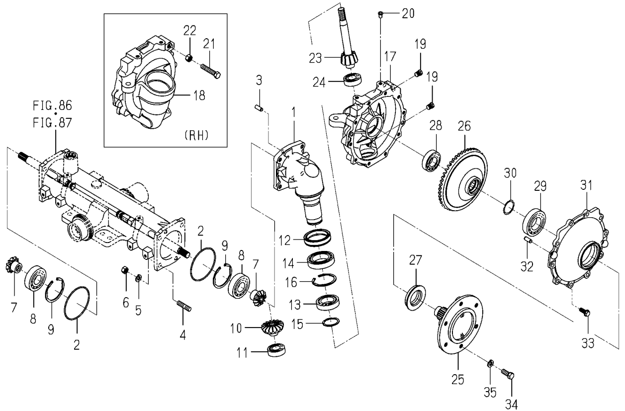
FIG. 88 GEAR(FINAL)SYSTEM
