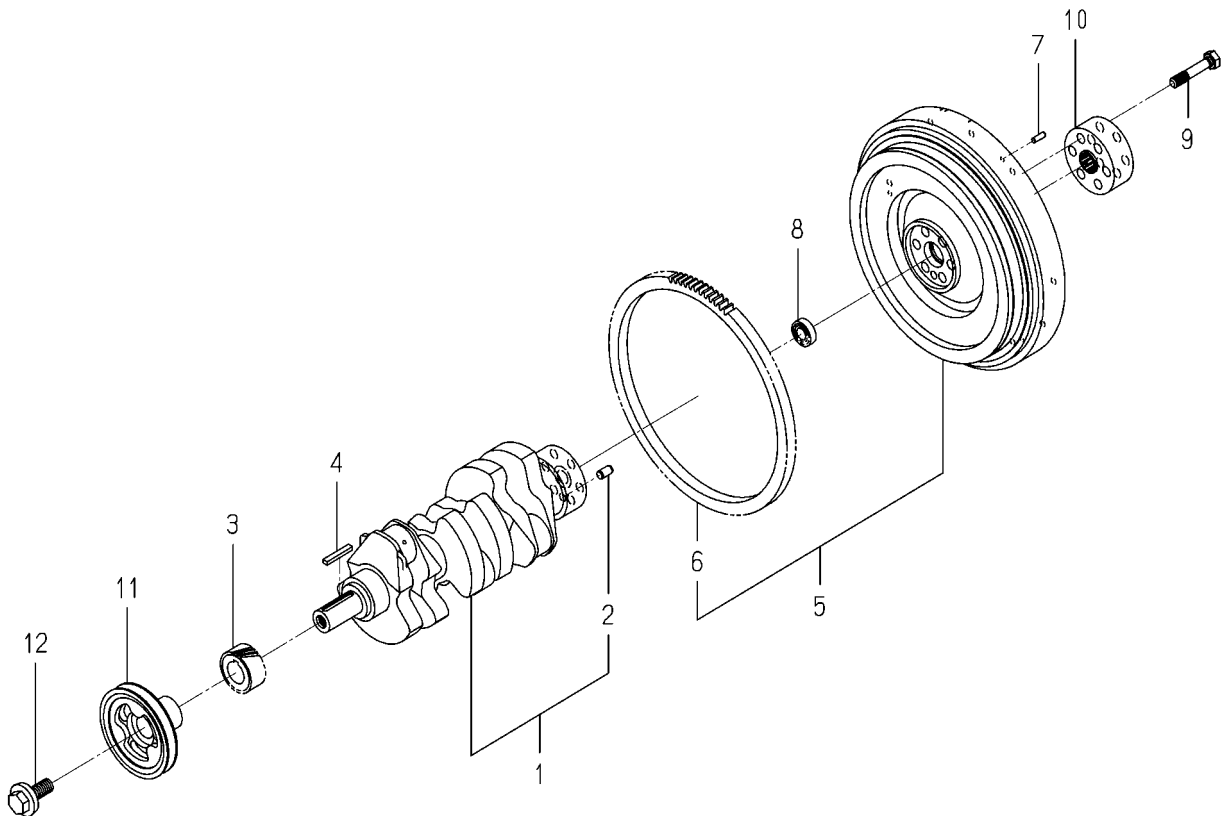
FIG. 19 CRANK SHAFT
