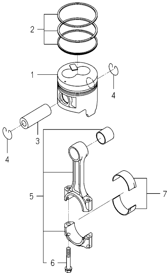
FIG. 15 PISTON
