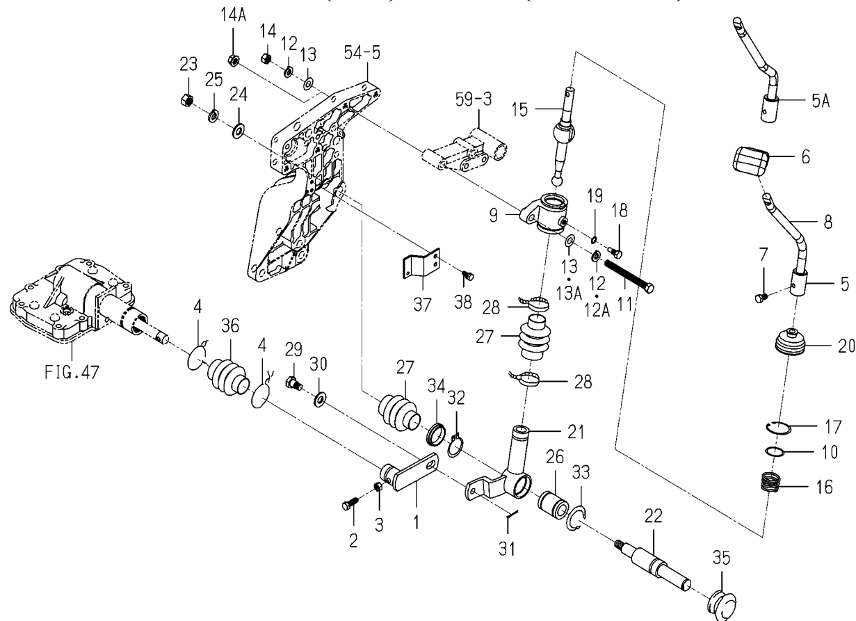
FIG. 55 LEVER(SUB)SYSTEM(6675 TYPE)
