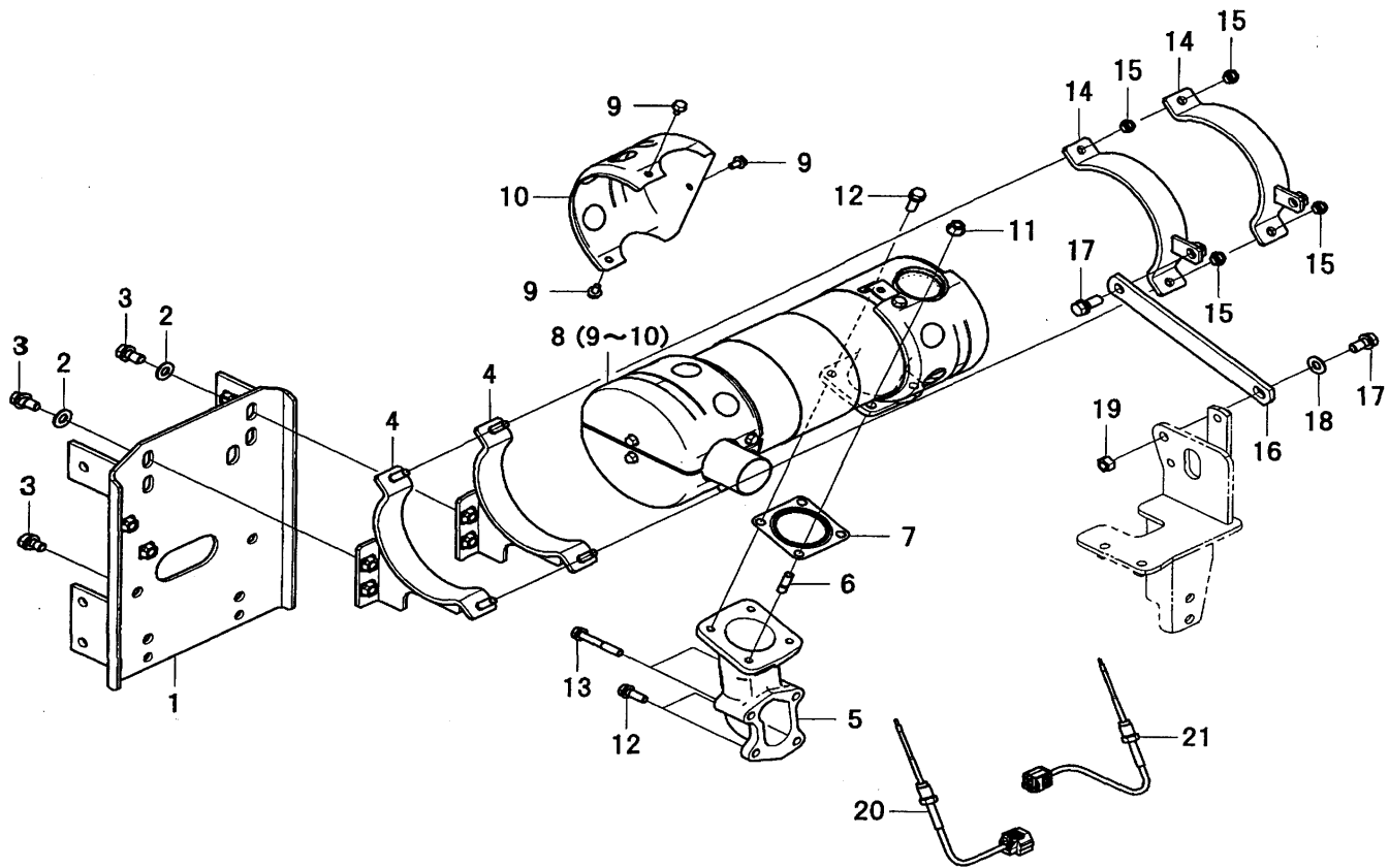
FIG.011 DOC
