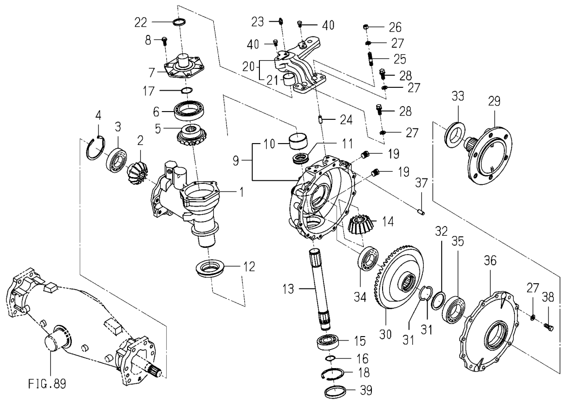
FIG. 90 CASE(GEAR/FRONT)SYSTEM(1/2)
