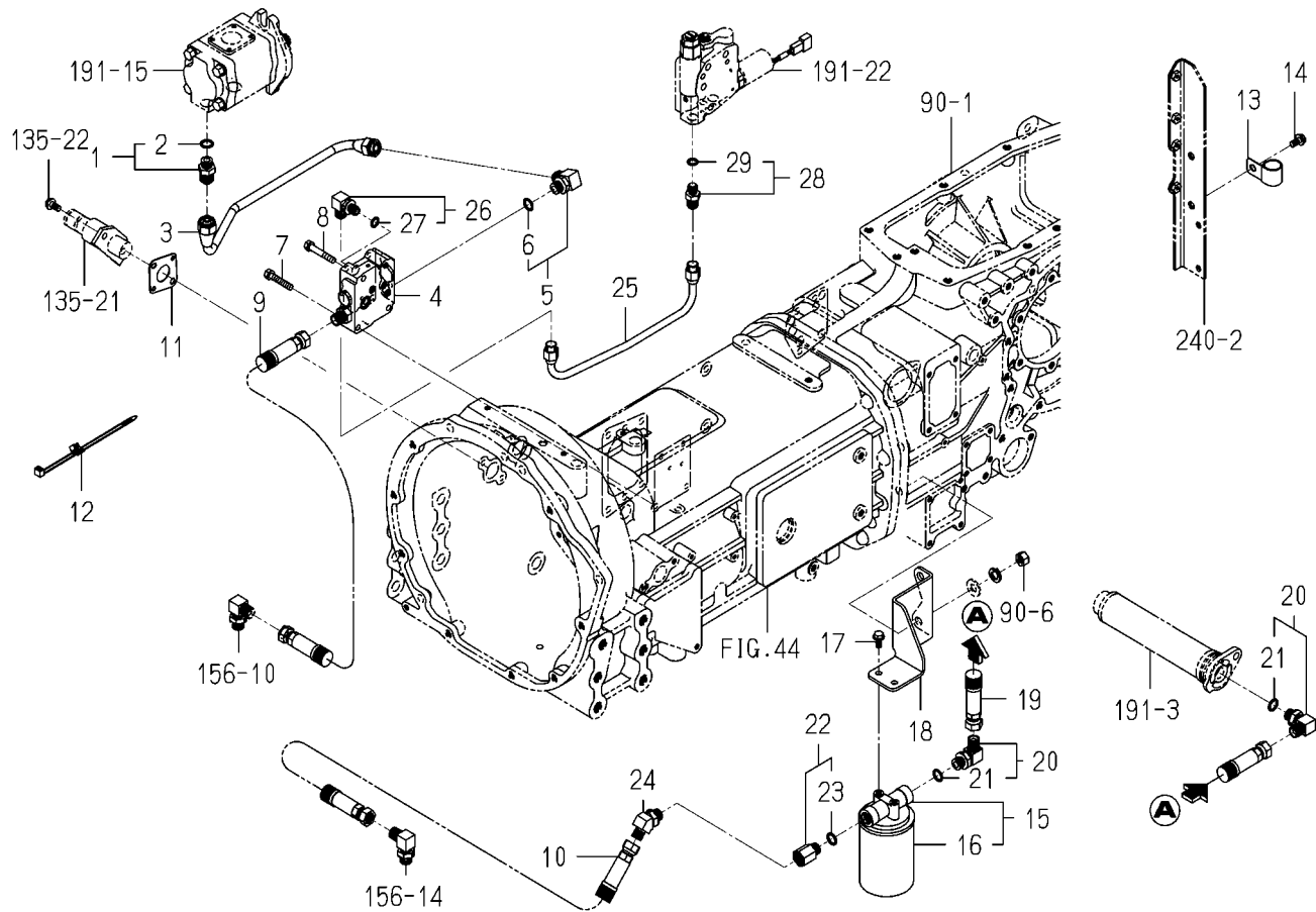
FIG.197 PIPING(SUB)SYSTEM(6375-SD TYPE)
