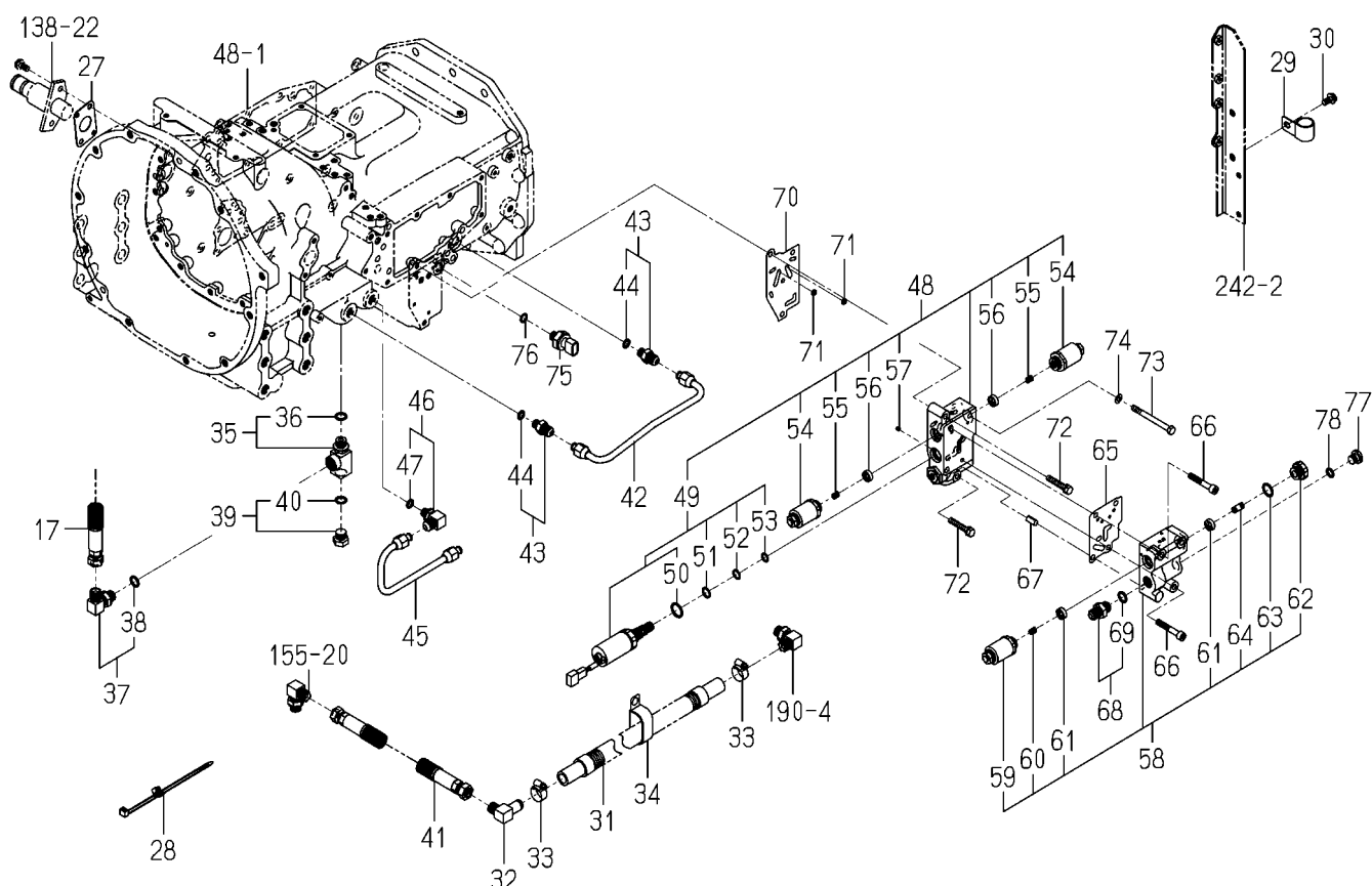
FIG.196 PIPING(SUB)SYSTEM(6495-G TYPE)(2/2)
