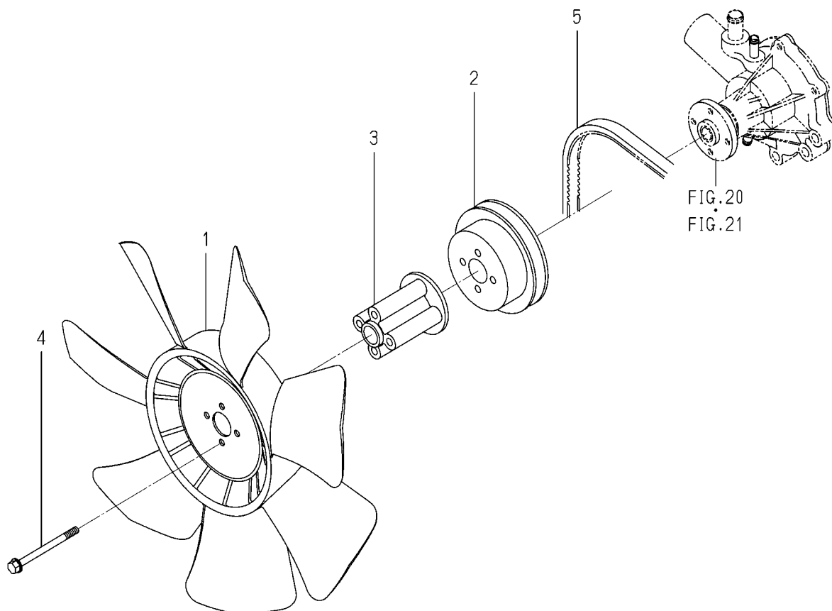
FIG. 22 COOLING FAN
