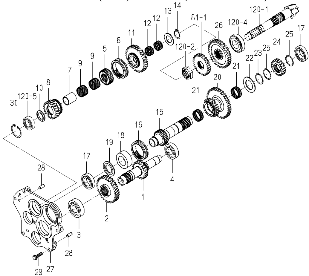
FIG. 76 GEAR(SUB)SYSTEM(6495-G TYPE)
