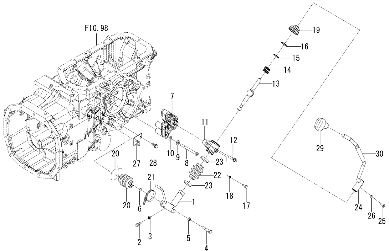
FIG.111 LEVER(SUB)SYSTEM(6375-G TYPE)
