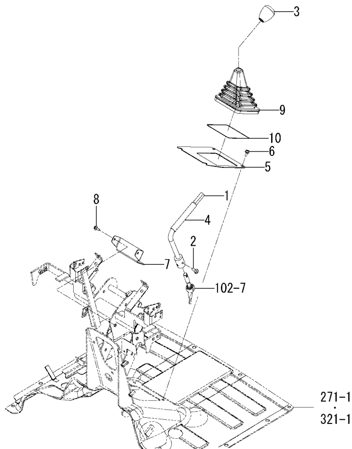
FIG.118 LEVER(PTO)SYSTEM(6495-G TYPE)
