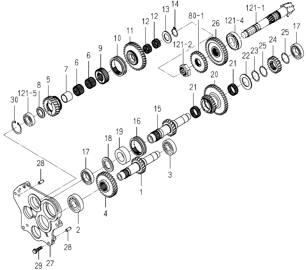
FIG. 73 GEAR(SUB)SYSTEM(6375-G TYPE)
