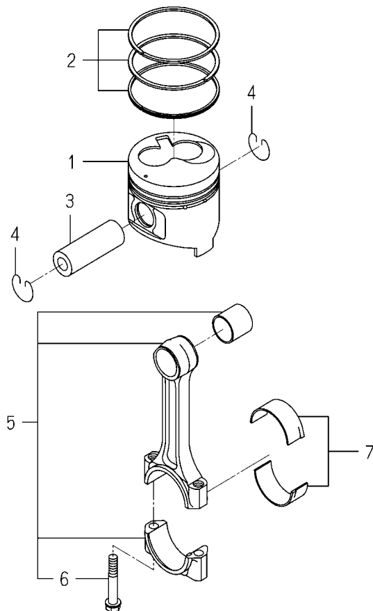
FIG. 20 PISTON
