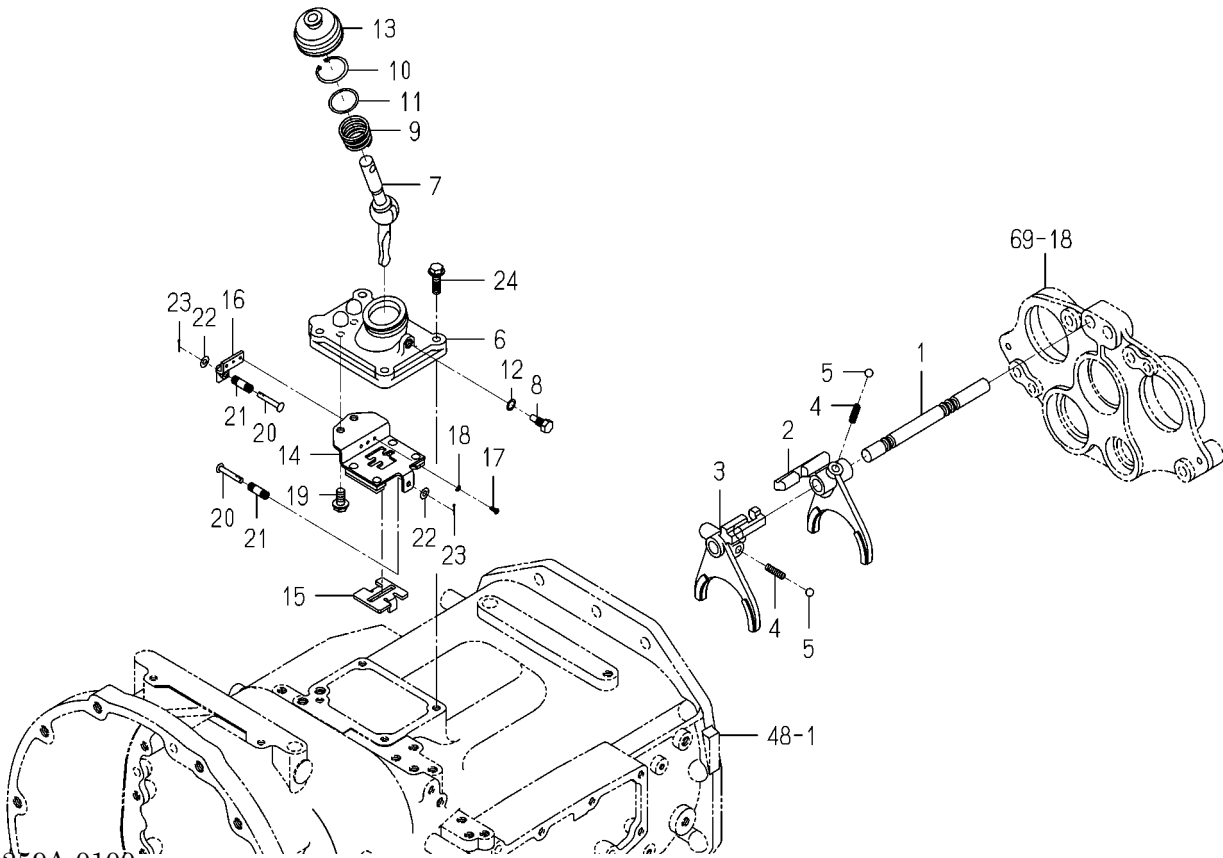
FIG.102 FORK(SHIFT/PTO)SYSTEM (6495-G TYPE)
