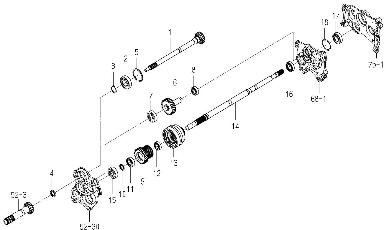
FIG. 61 GEAR(PTO)SYSTEM(6375-SD TYPE)
