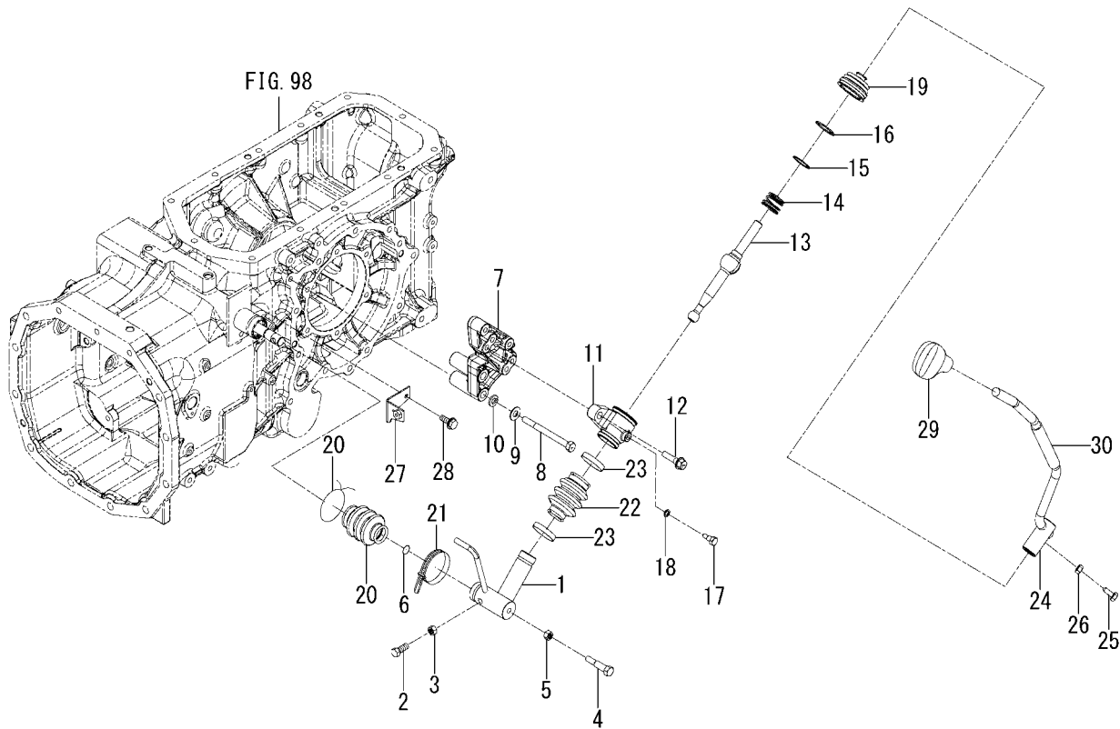
FIG.112 LEVER(SUB)SYSTEM(6495-G TYPE)
