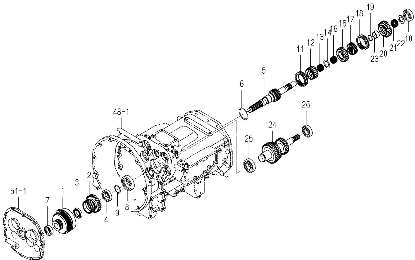
FIG. 59 GEAR(PTO)SYSTEM(6495-G TYPE)
