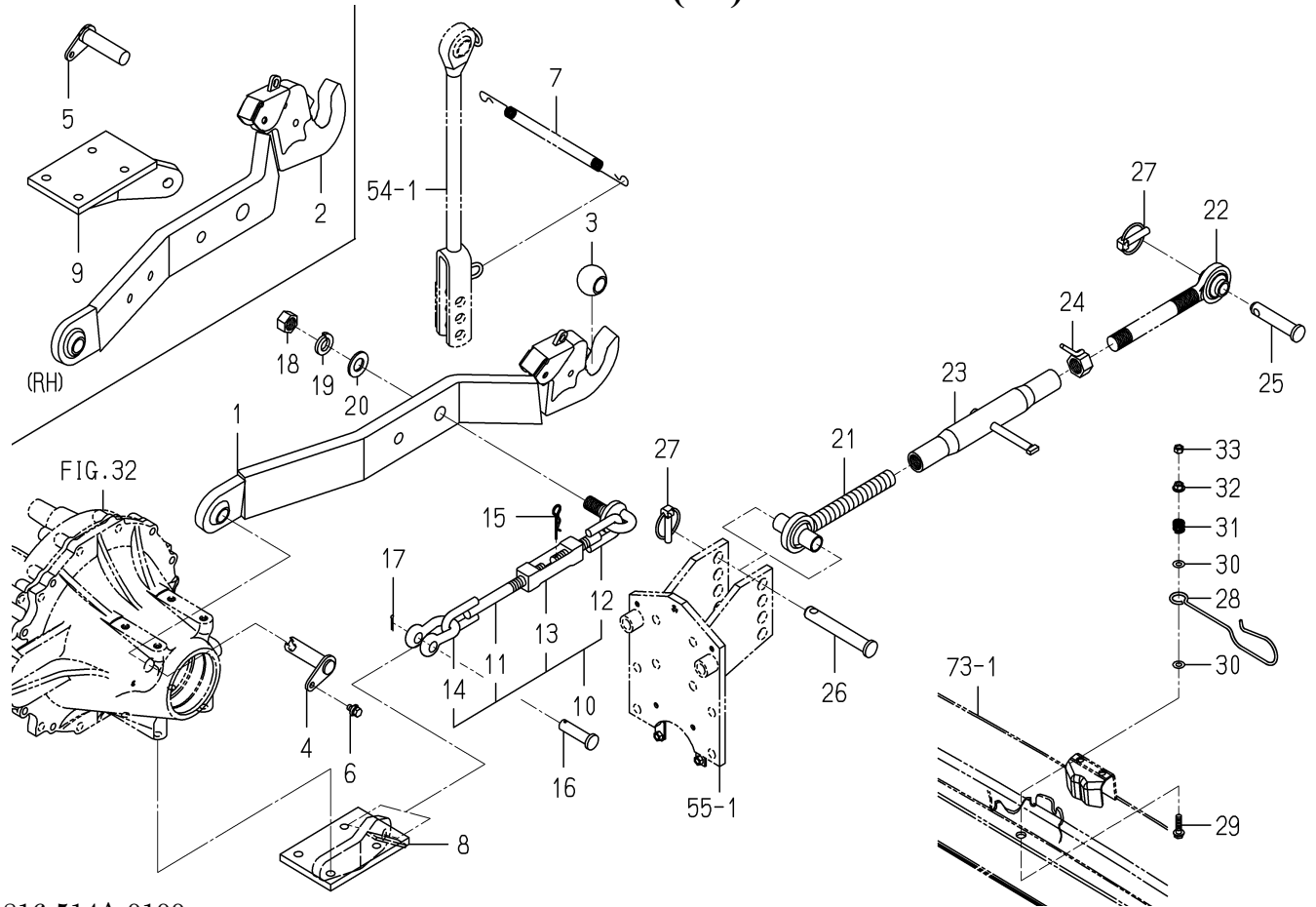
FIG. 53 LINK(3P)SYSTEM
