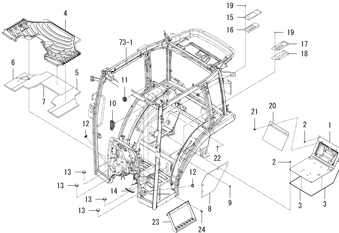
FIG. 64 FLOOR(REAR)SYSTEM
