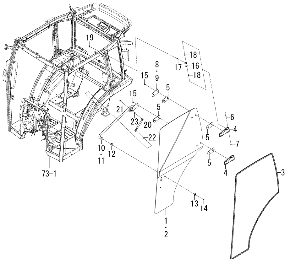
FIG. 76 DOOR SYSTEM
