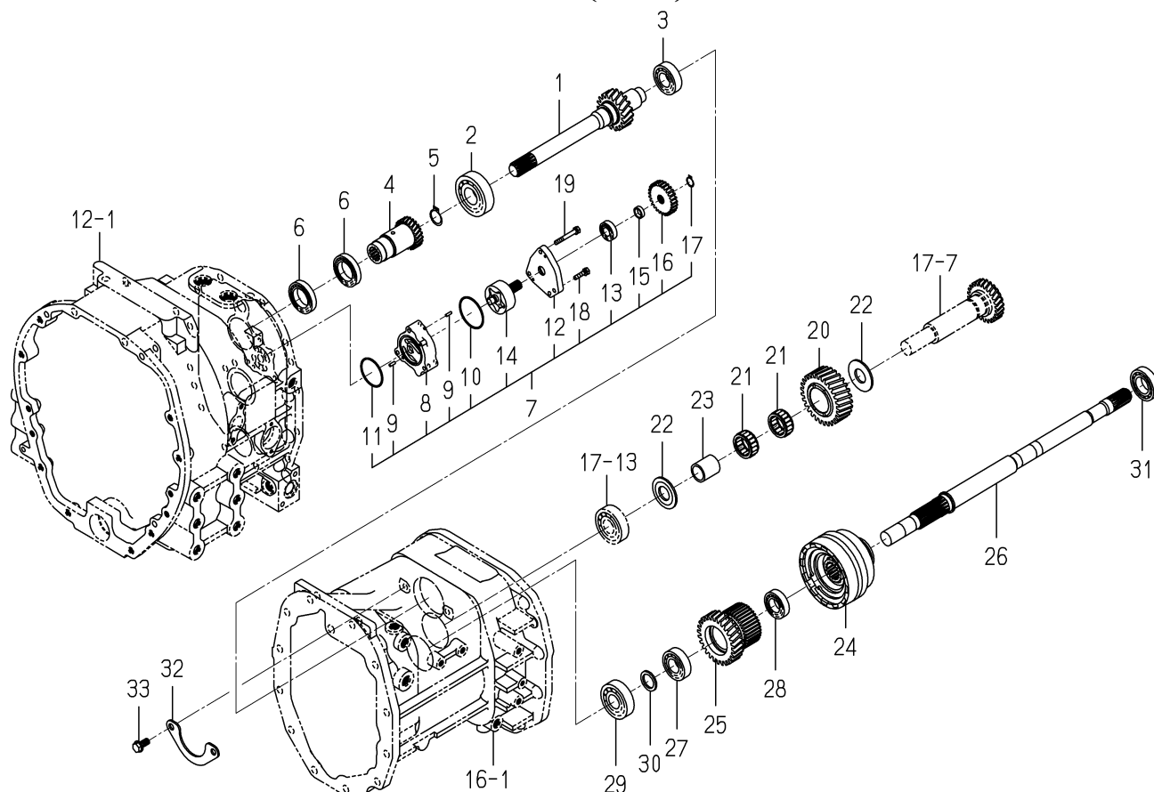
FIG. 15 GEAR(PTO)SYSTEM
