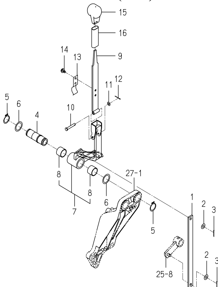
FIG. 29 LEVER(PTO)SYSTEM
