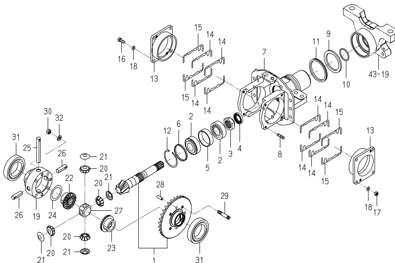
FIG. 42 CASE(BEVEL)SYSTEM
