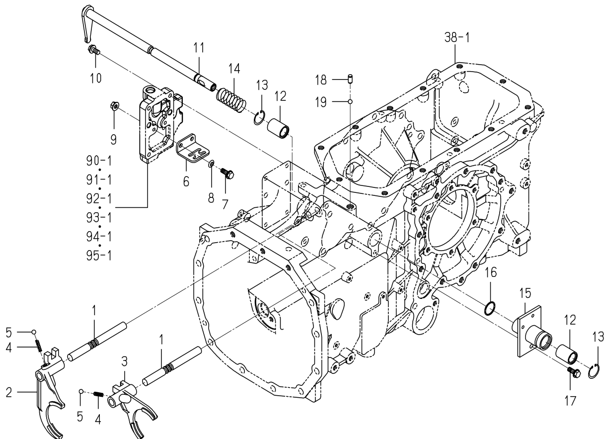
FIG. 41 FORK(SHIFT/SUB)SYSTEM
