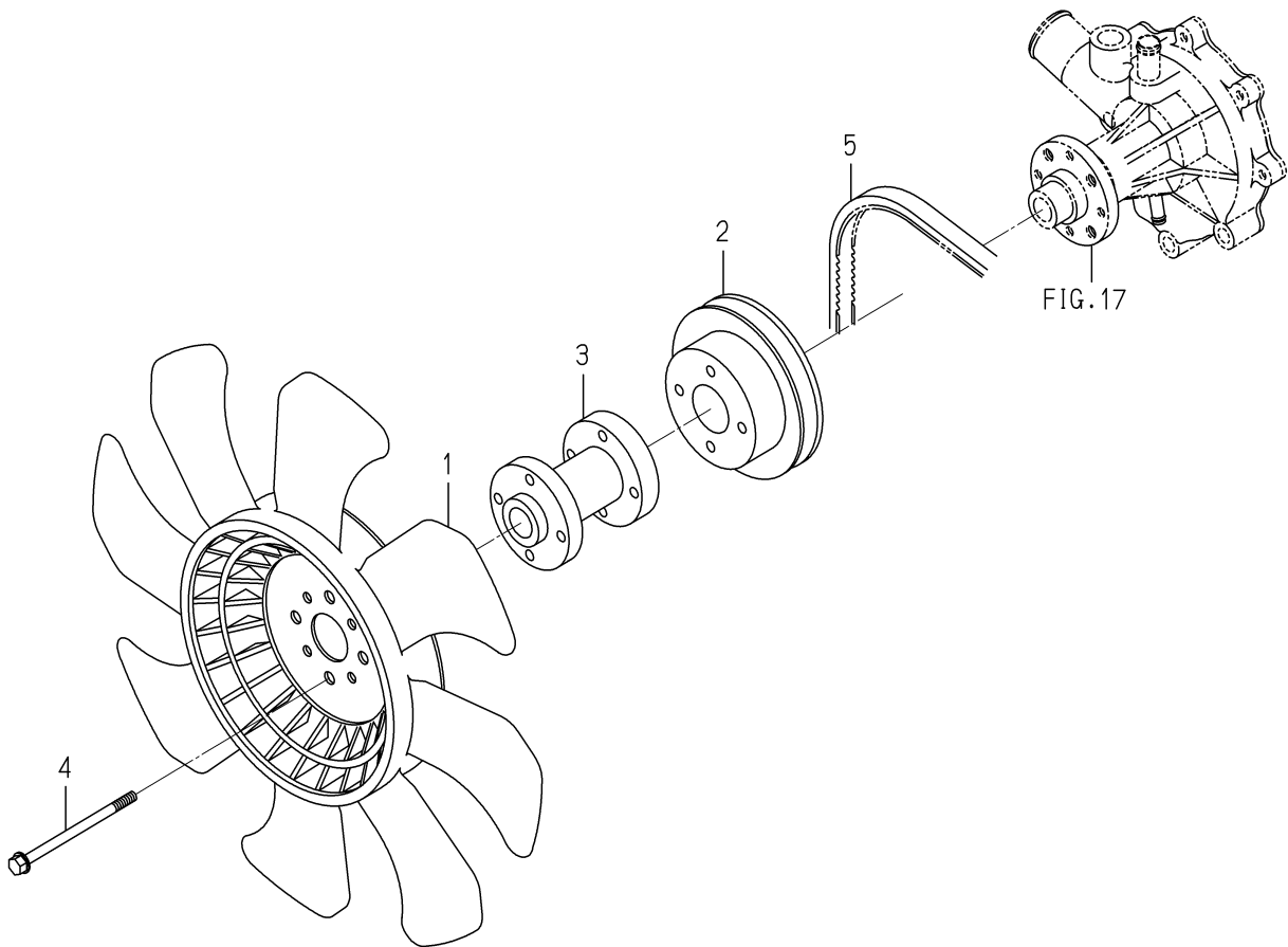
FIG. 18 COOLING FAN
