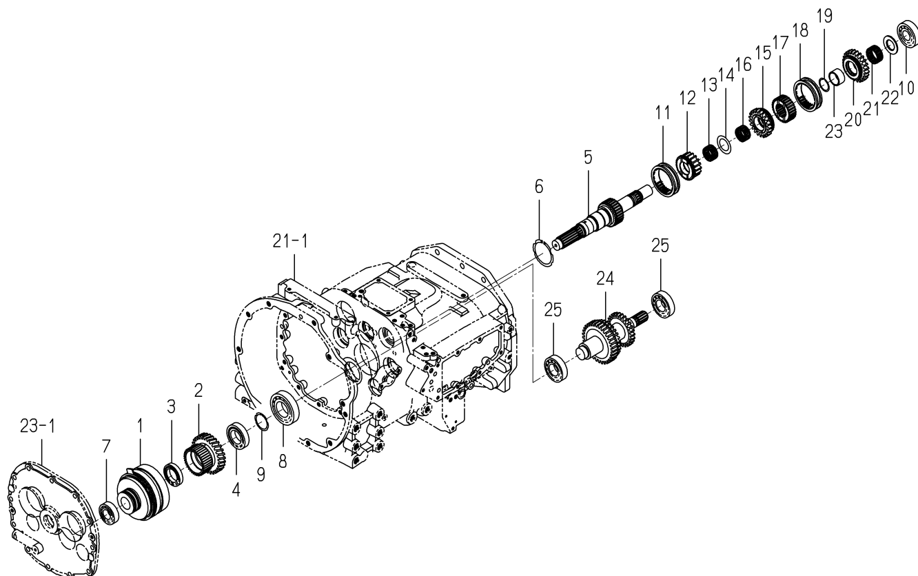
FIG. 25 GEAR(PTO)SYSTEM(6370 TYPE)
