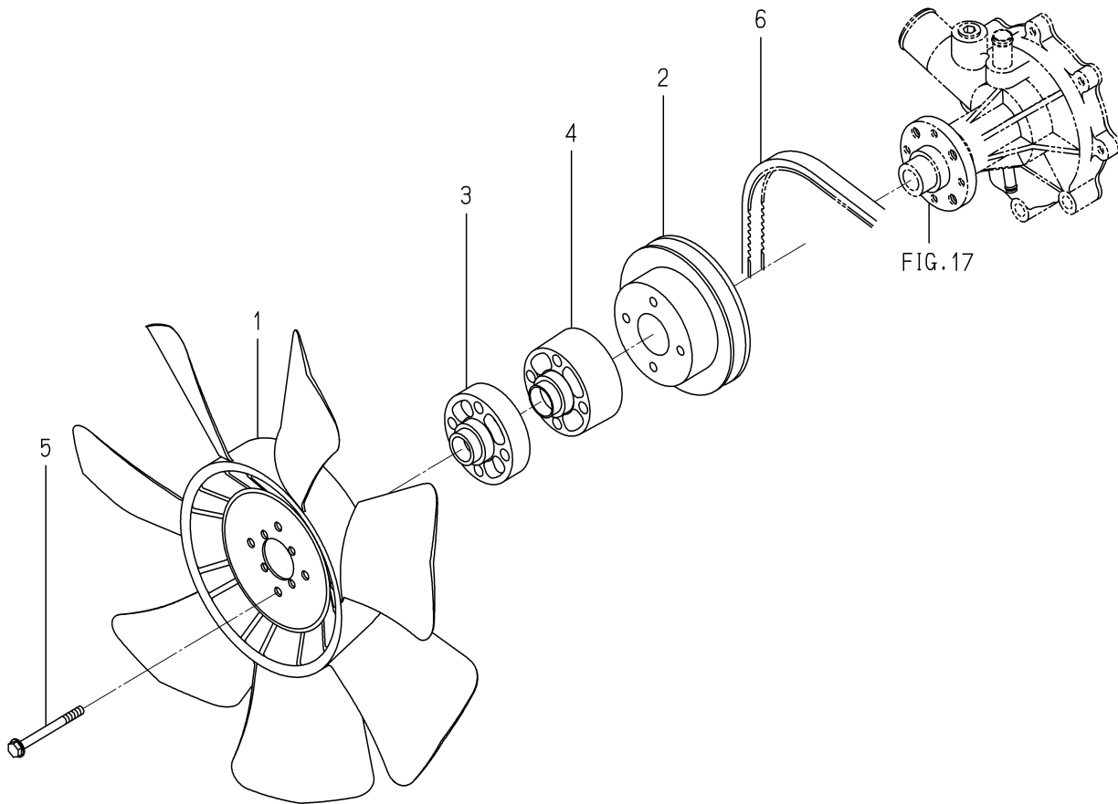
FIG. 18 COOLING FAN
