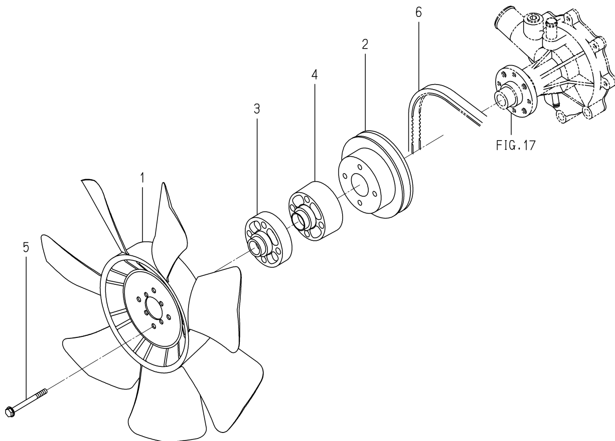
FIG. 18 COOLING FAN
