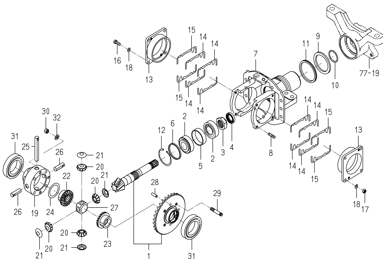
FIG. 75 CASE(BEVEL)SYSTEM(6490 TYPE)
