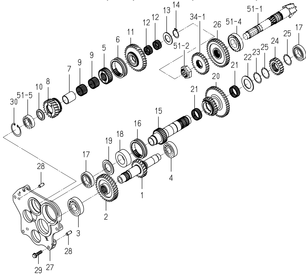
FIG. 32 GEAR(SUB)SYSTEM(6490 TYPE)
