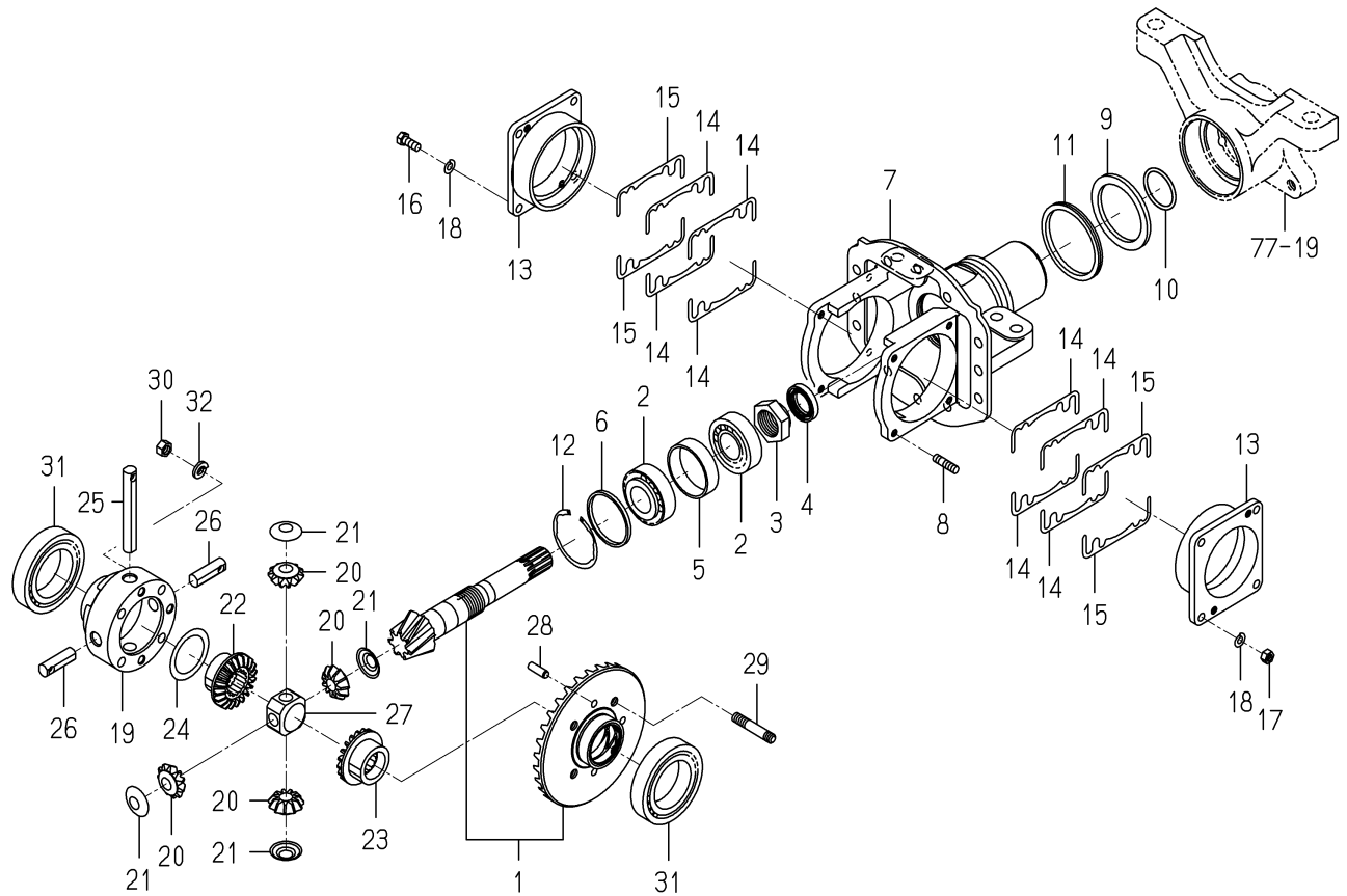
FIG. 75 CASE(BEVEL)SYSTEM(6490 TYPE)
