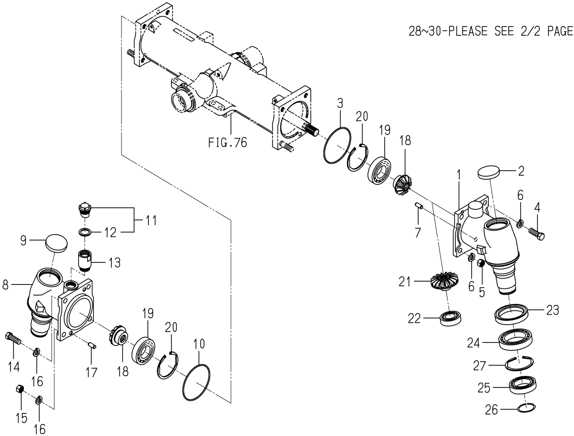
FIG. 78 CASE(GEAR/FRONT)SYSTEM(6370 TYPE)(1/2)
