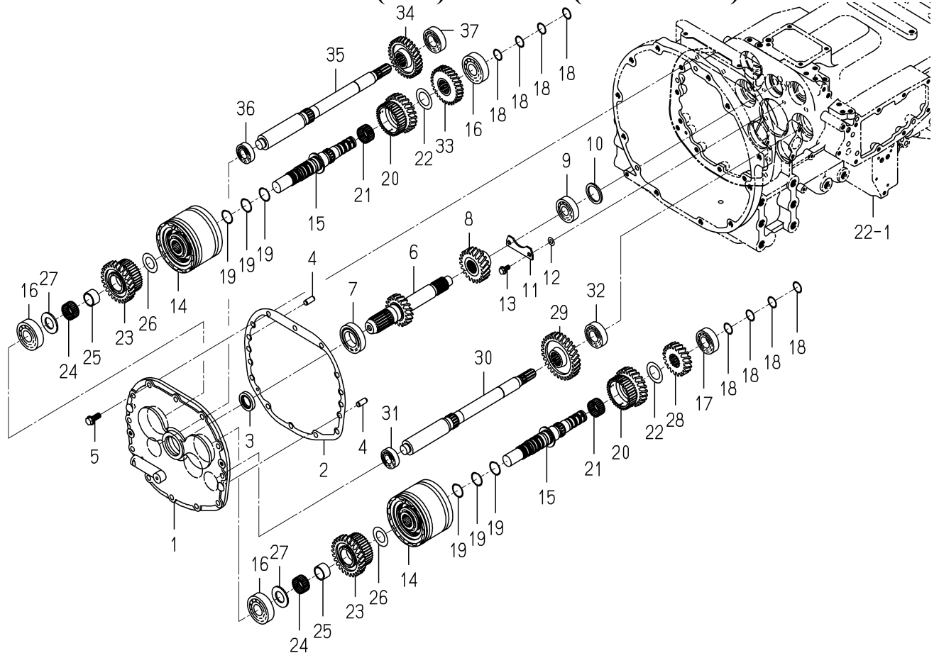
FIG. 24 GEAR(H/L)SYSTEM(6490 TYPE)
