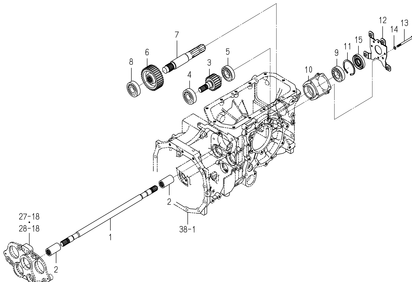
FIG. 35 GEAR(PTO)SYSTEM
