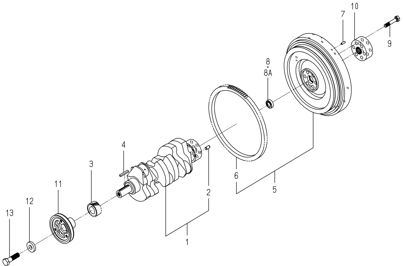
FIG. 18 CRANK SHAFT
