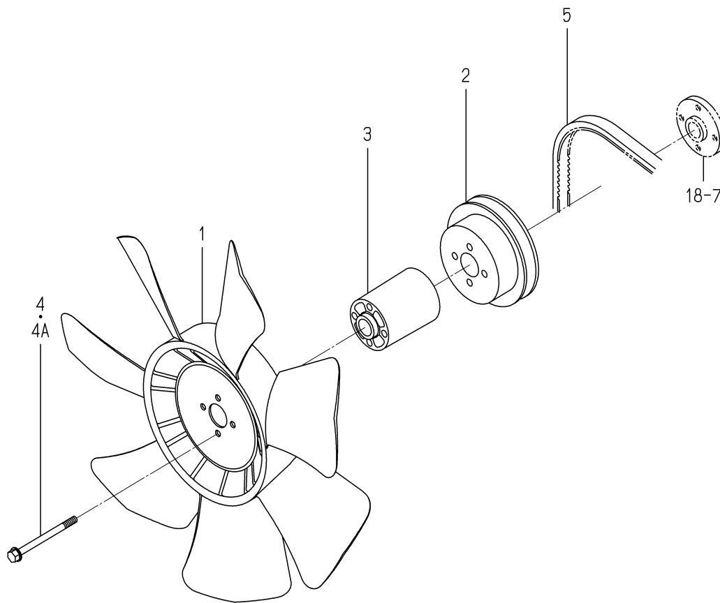
FIG. 19 COOLING FAN
