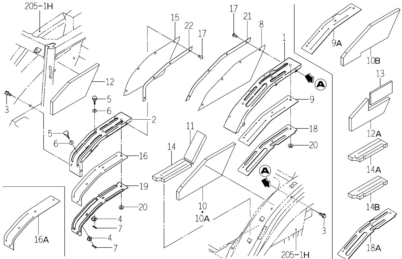
FIG.144 LEVER GUIDE SYSTEM (QC TYPE-TG5330E4-No.730-/TG5390E4-No.1009-)
