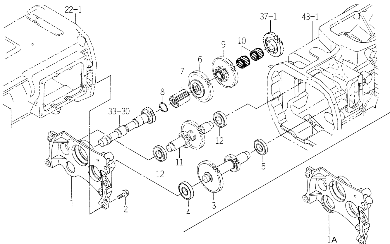
FIG. 36 GEAR (SUB) SYSTEM (Q TYPE)
