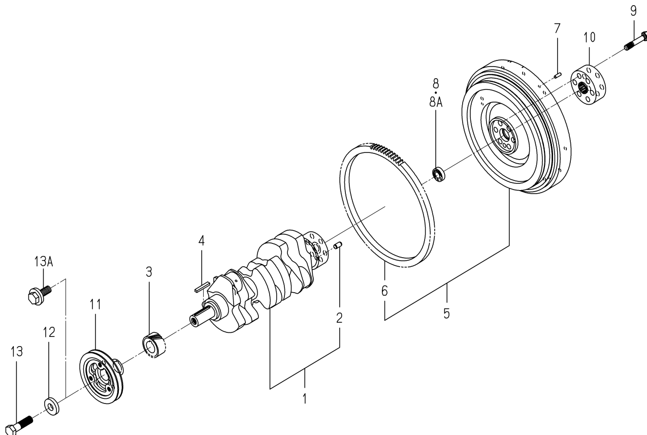
FIG. 18 CRANK SHAFT
