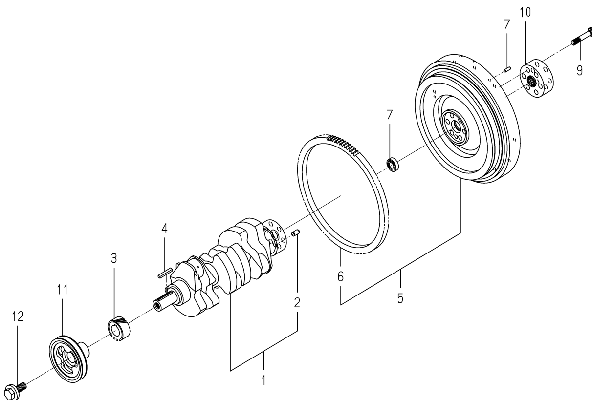
FIG. 19 CRANK SHAFT
