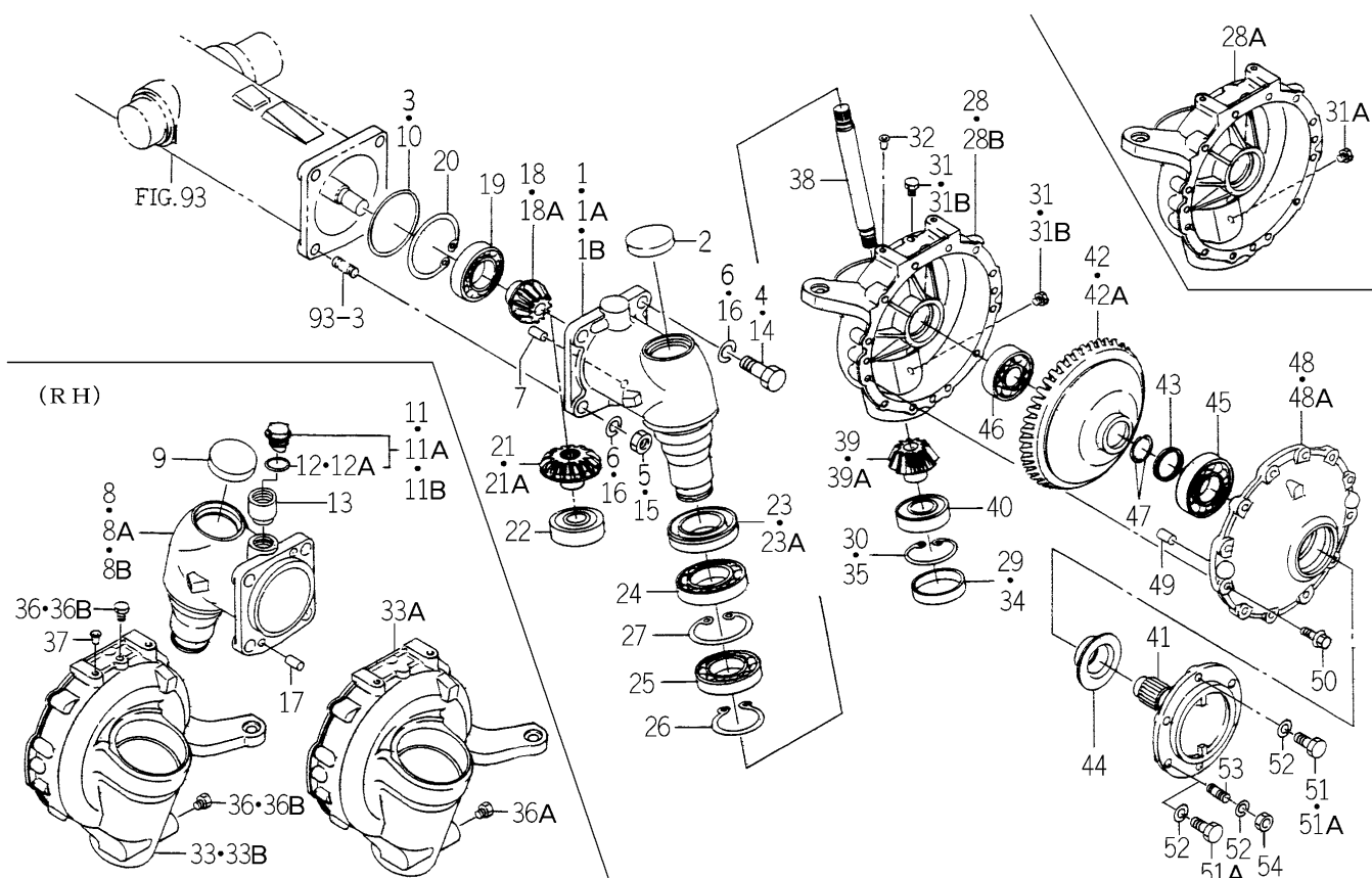
FIG. 95 CASE (GEAR/FRONT) SYSTEM
