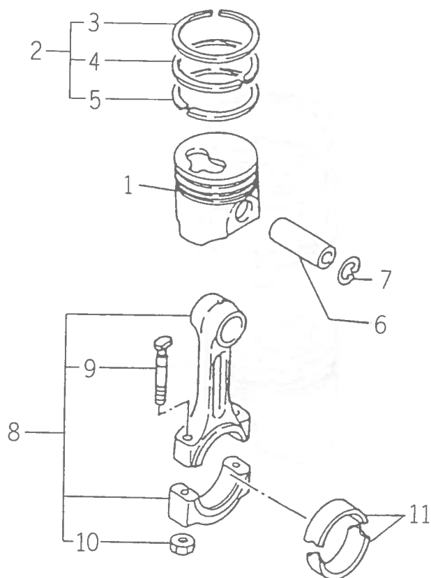
FIG. 14 PISTON
