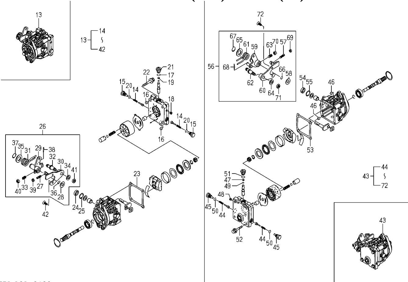
FIG. 10 PUMP(HST)SYSTEM(2/6)
