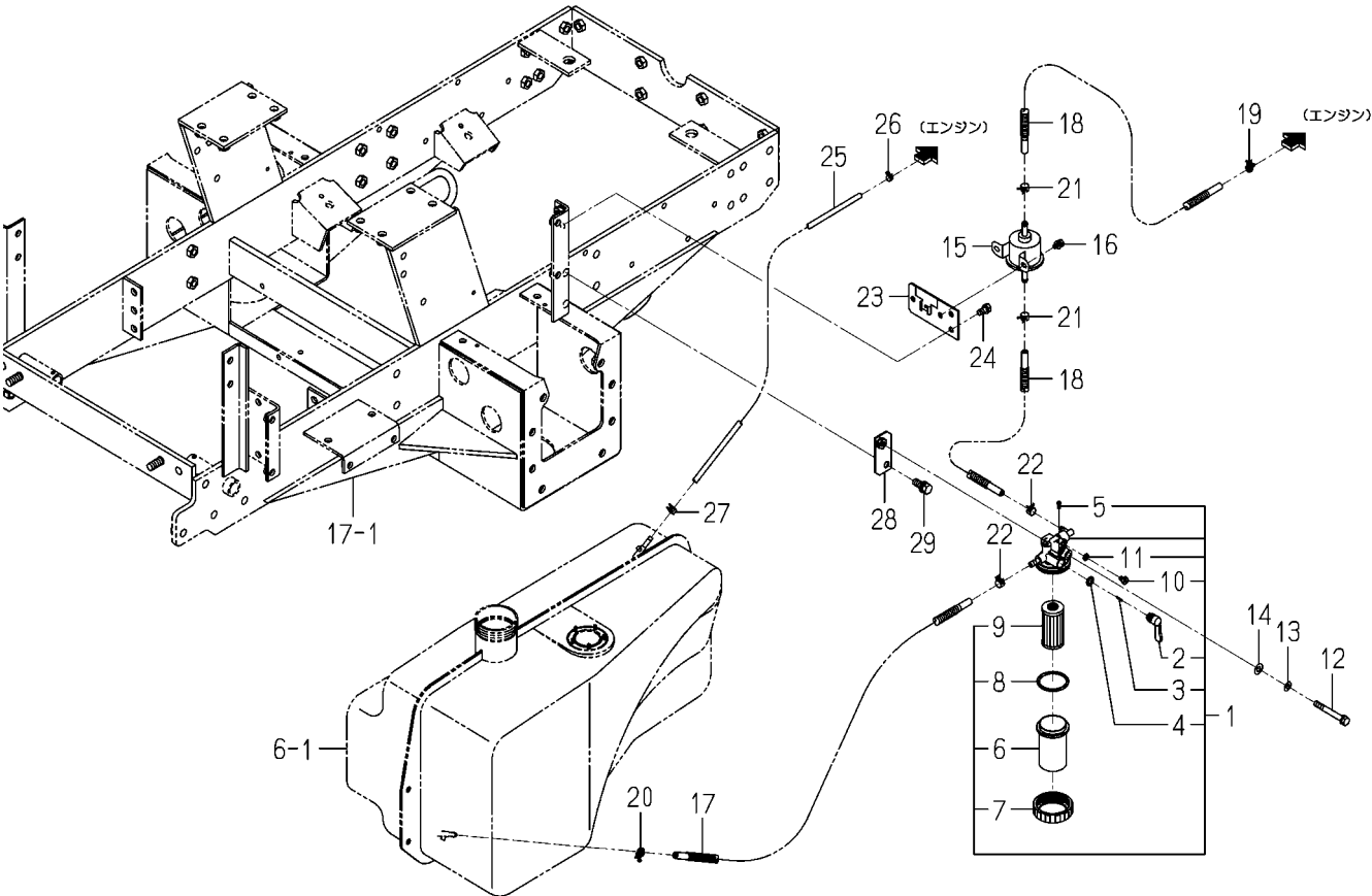
FIG. 5 PUMP(FUEL)SYSTEM
