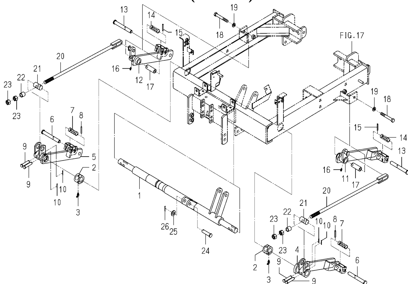
FIG. 25 LINK(MOWER)SYSTEM
