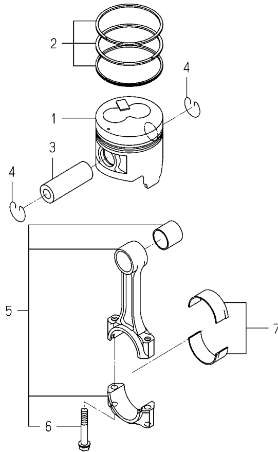
FIG. 14 PISTON
