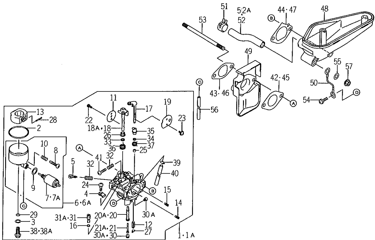
FIG. 8 CARBURETOR
