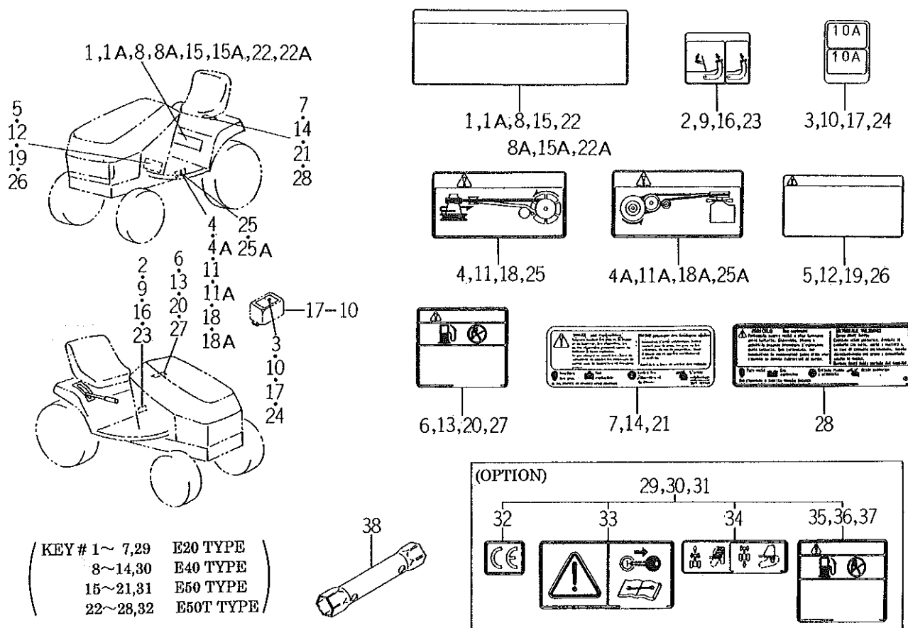
FIG. 19 LABEL
