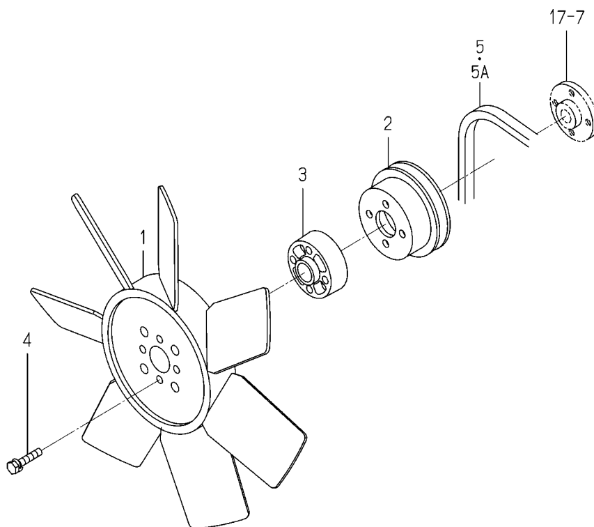
FIG. 18 COOLING FAN
