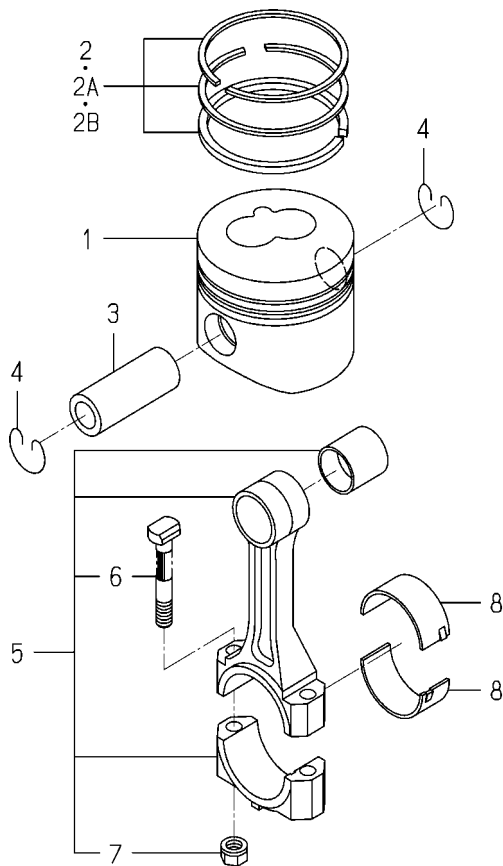
FIG. 13 PISTON
