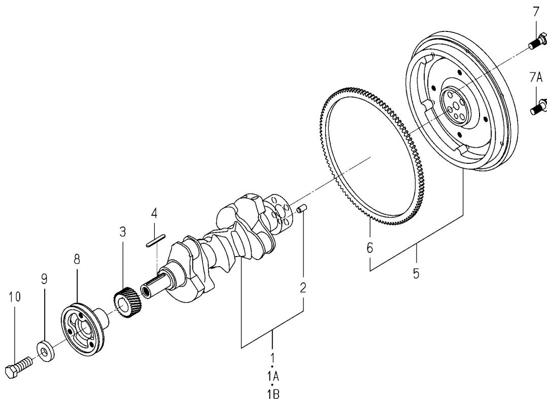
FIG. 15 CRANK SHAFT
