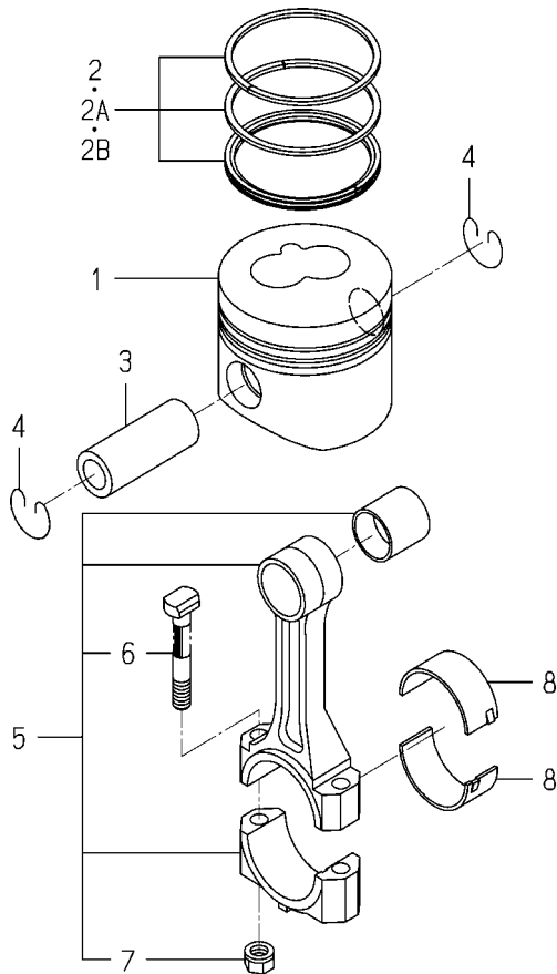
FIG. 13 PISTON
