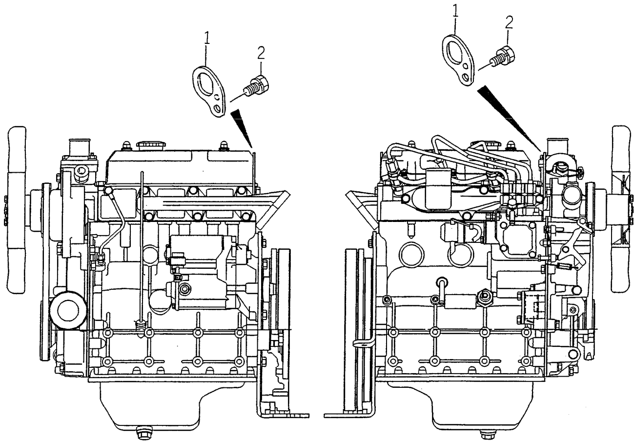
FIG. 10 HANGER
