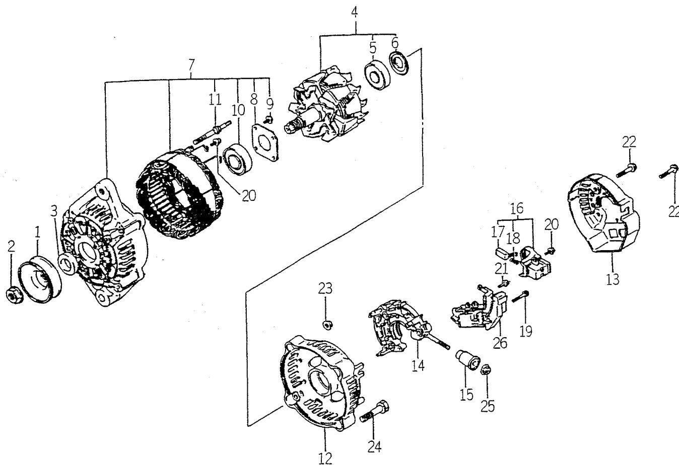
FIG. 28 6281 - 200 - 016 - 00
