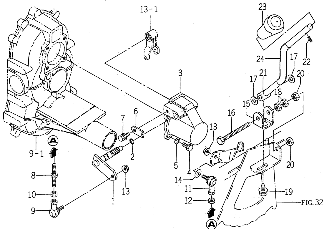
FIG. 12 SHIFT SYSTEM
