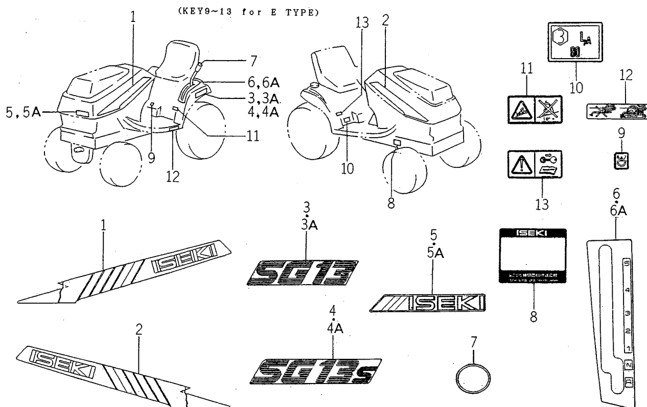
FIG. 43 MARKS (1)
