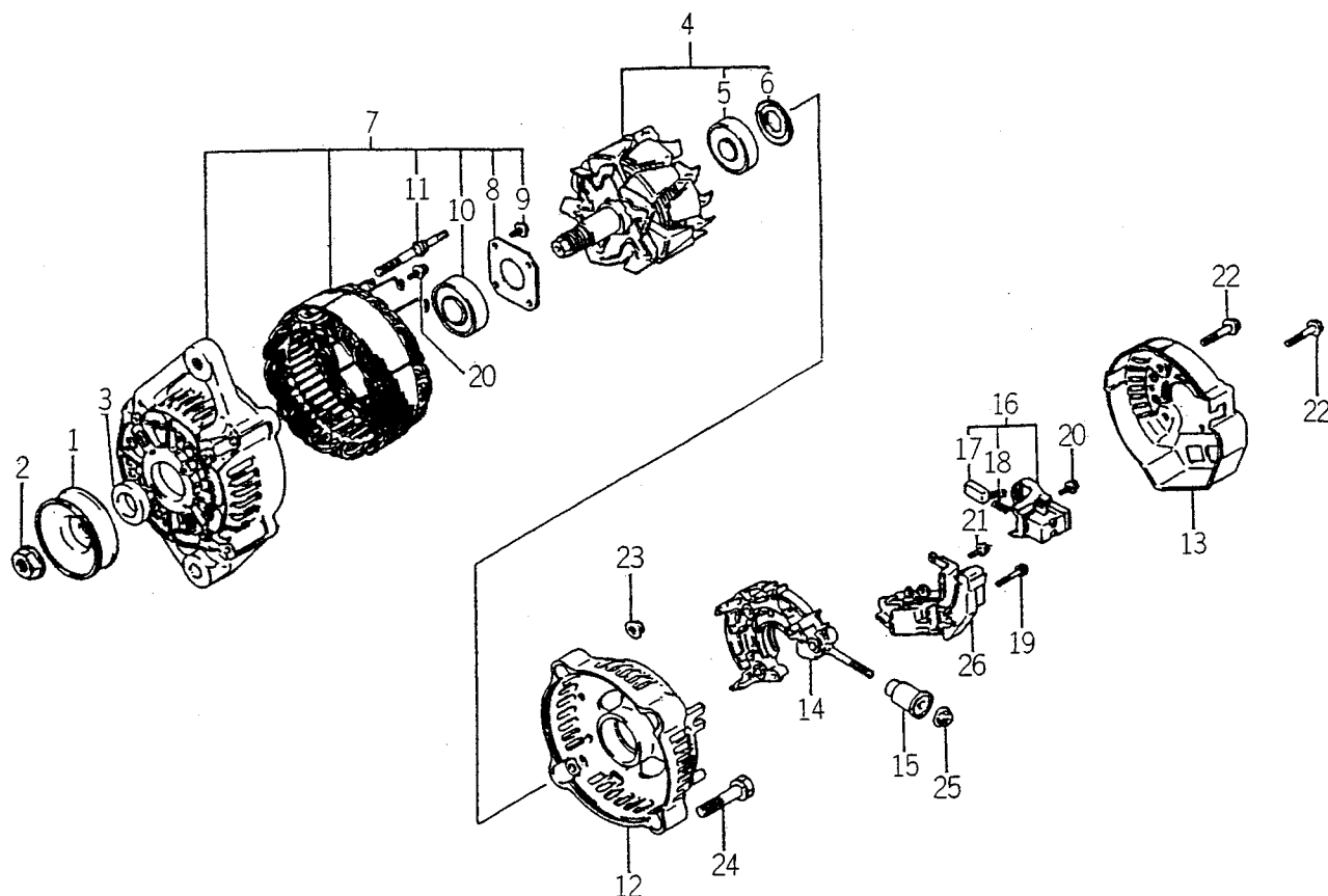
FIG. 28 6281 - 200 - 016 - 00
