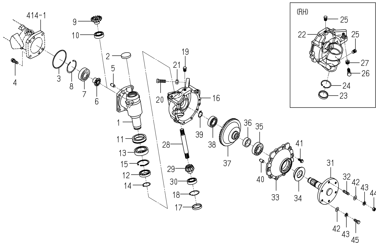
FIG.416 CASE(GEAR/FINAL)SYSTEM(SFH240F)
