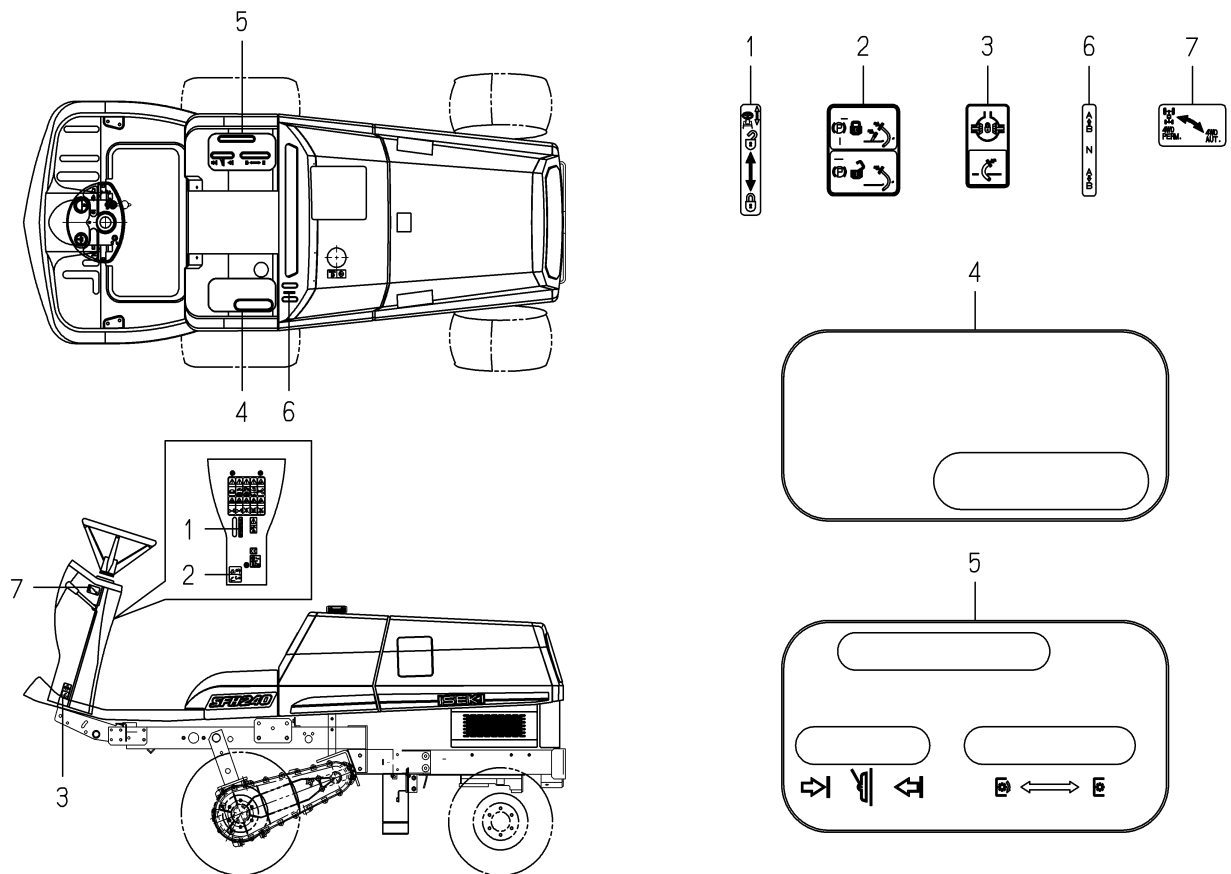
FIG.907 LABEL(CONTROL)(SFH240F-WE42C TYPE)
