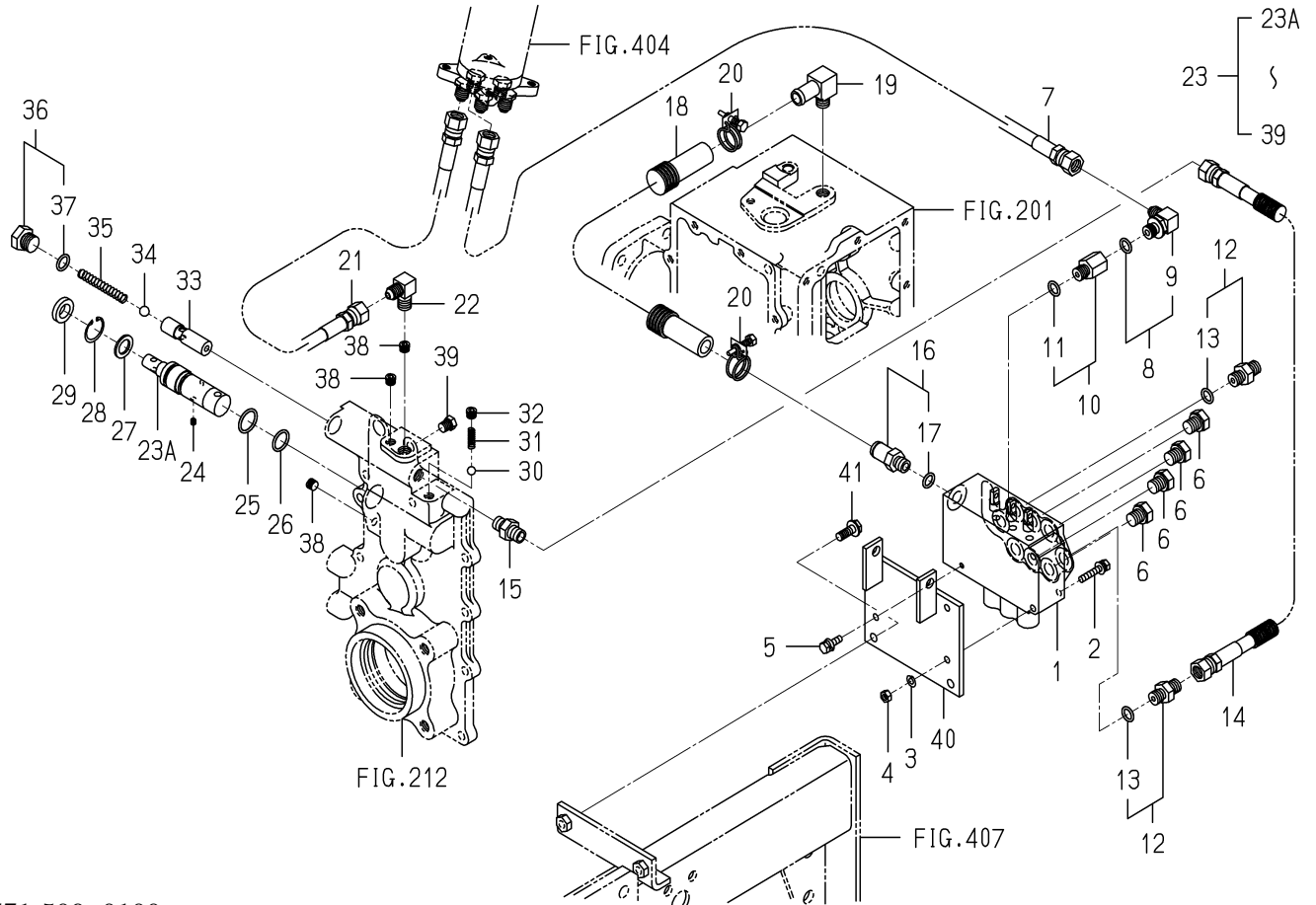
FIG.506 PIPING(CONTROL)SYSTEM
