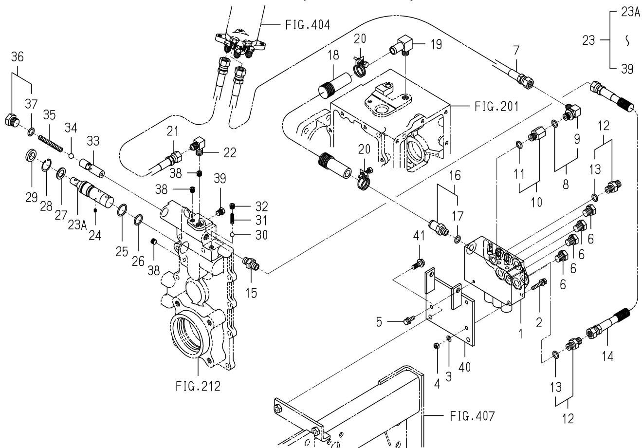
FIG.506 PIPING(CONTROL)SYSTEM
