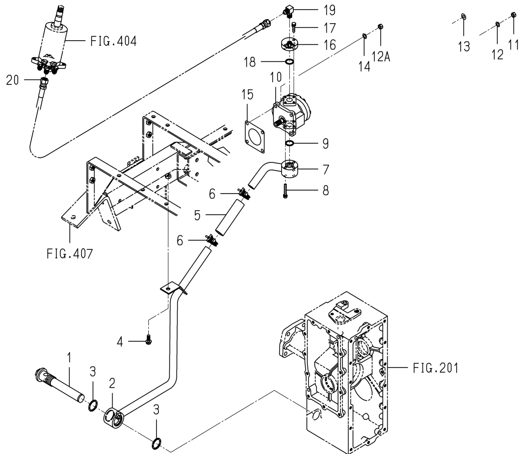
FIG.505 PIPING(PUMP)SYSTEM
