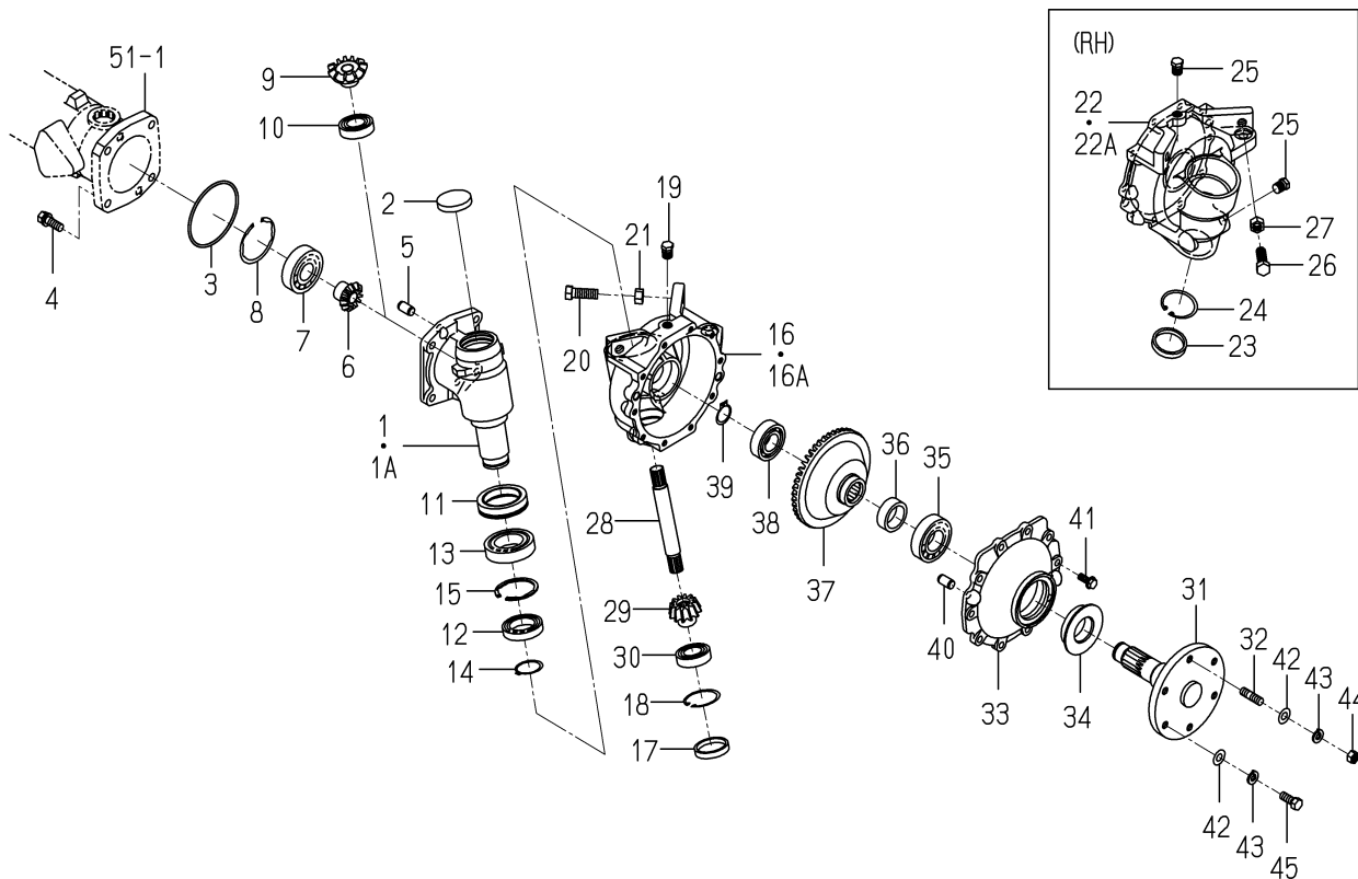
FIG. 53 CASE(GEAR/FINAL)SYSTEM(SFH240)
