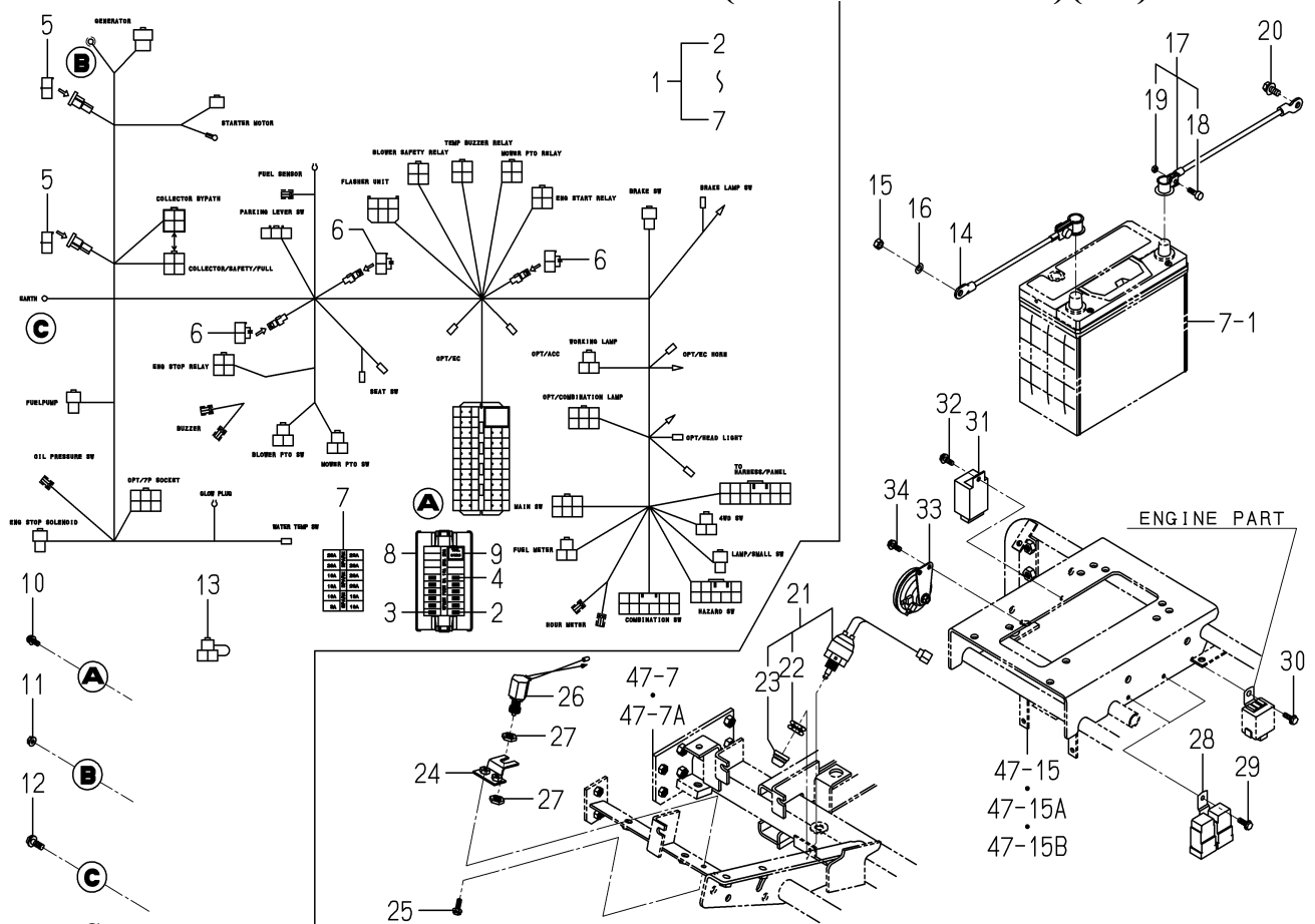
FIG. 79 HARNESS SYSTEM(SFH220:G TYPE)(1/2)
