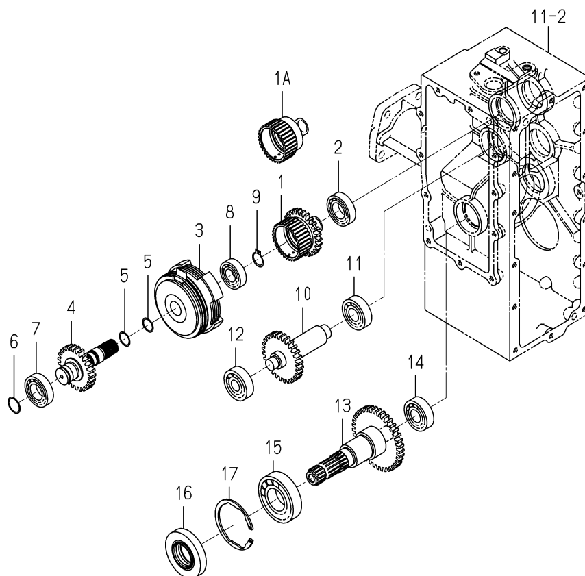
FIG. 24 DRIVE(PTO/BLOWER)SYSTEM
