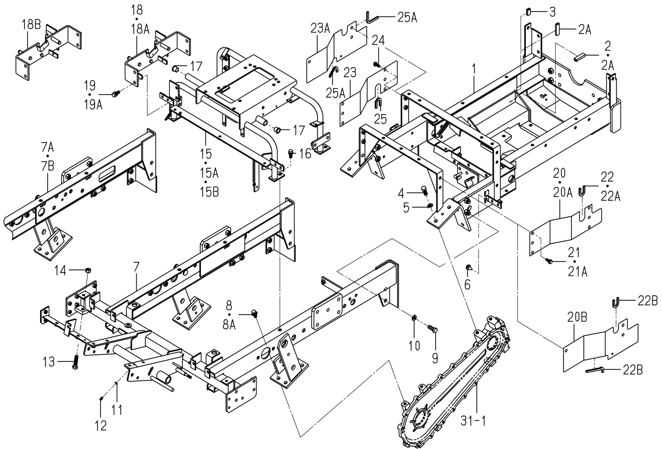
FIG. 46 FRAME SYSTEM(SFH240)
