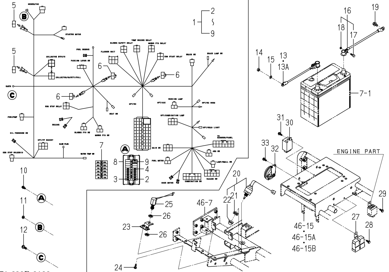
FIG. 78 HARNESS SYSTEM(SFH240:G TYPE)(1/2)
