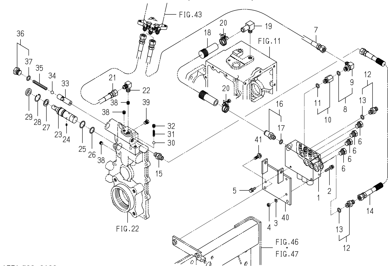
FIG. 62 PIPING(CONTROL)SYSTEM
