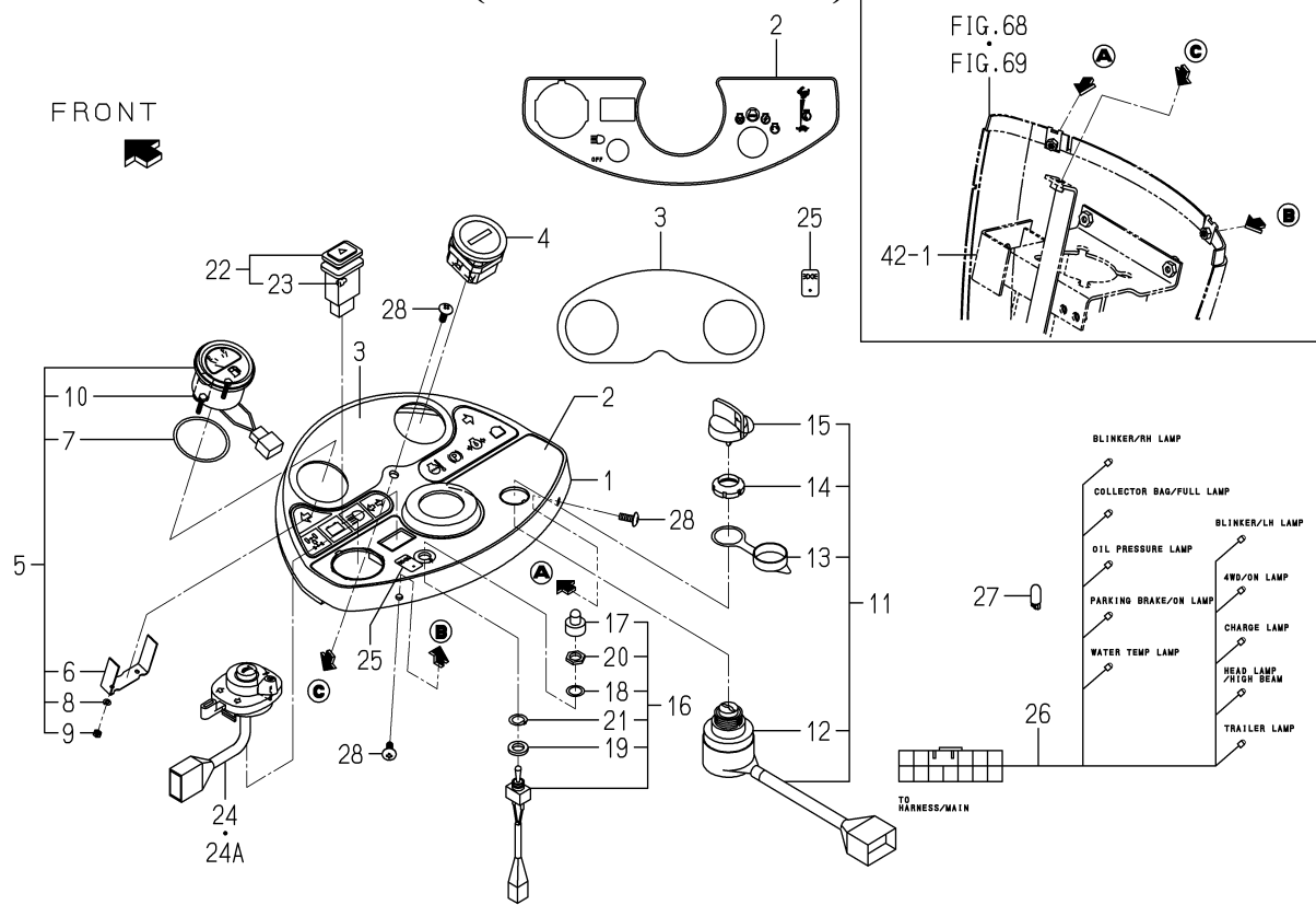
FIG. 75 PANEL SYSTEM (SFH220:G TYPE) (SFH240:G TYPE)
