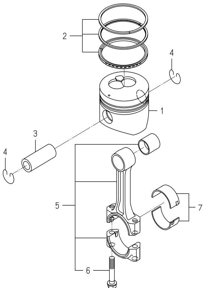
FIG. 14 PISTON
