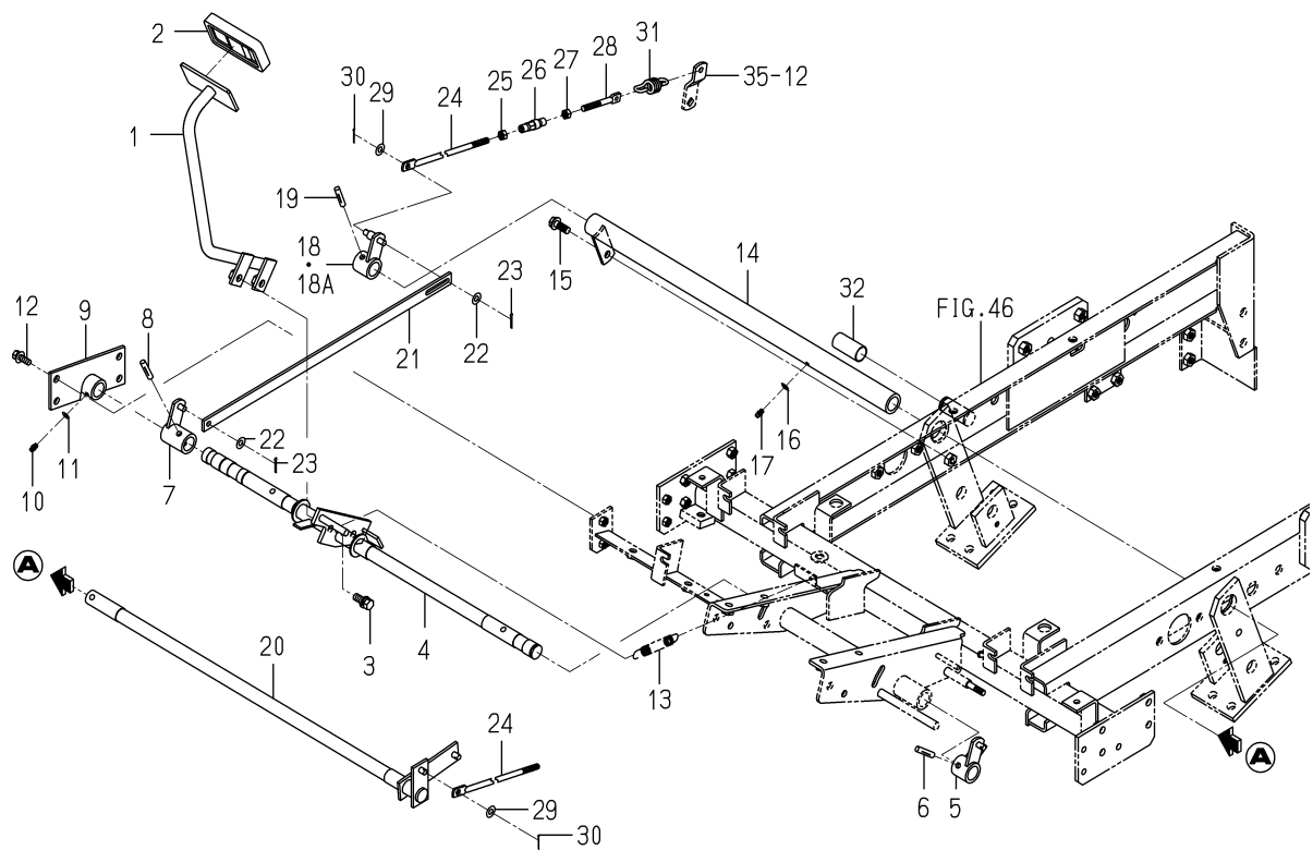
FIG. 37 PEDAL(BRAKE)SYSTEM (SFH220:G TYPE) (SFH240:G TYPE)
