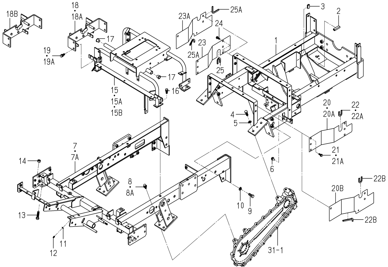
FIG. 47 FRAME SYSTEM(SFH220)
