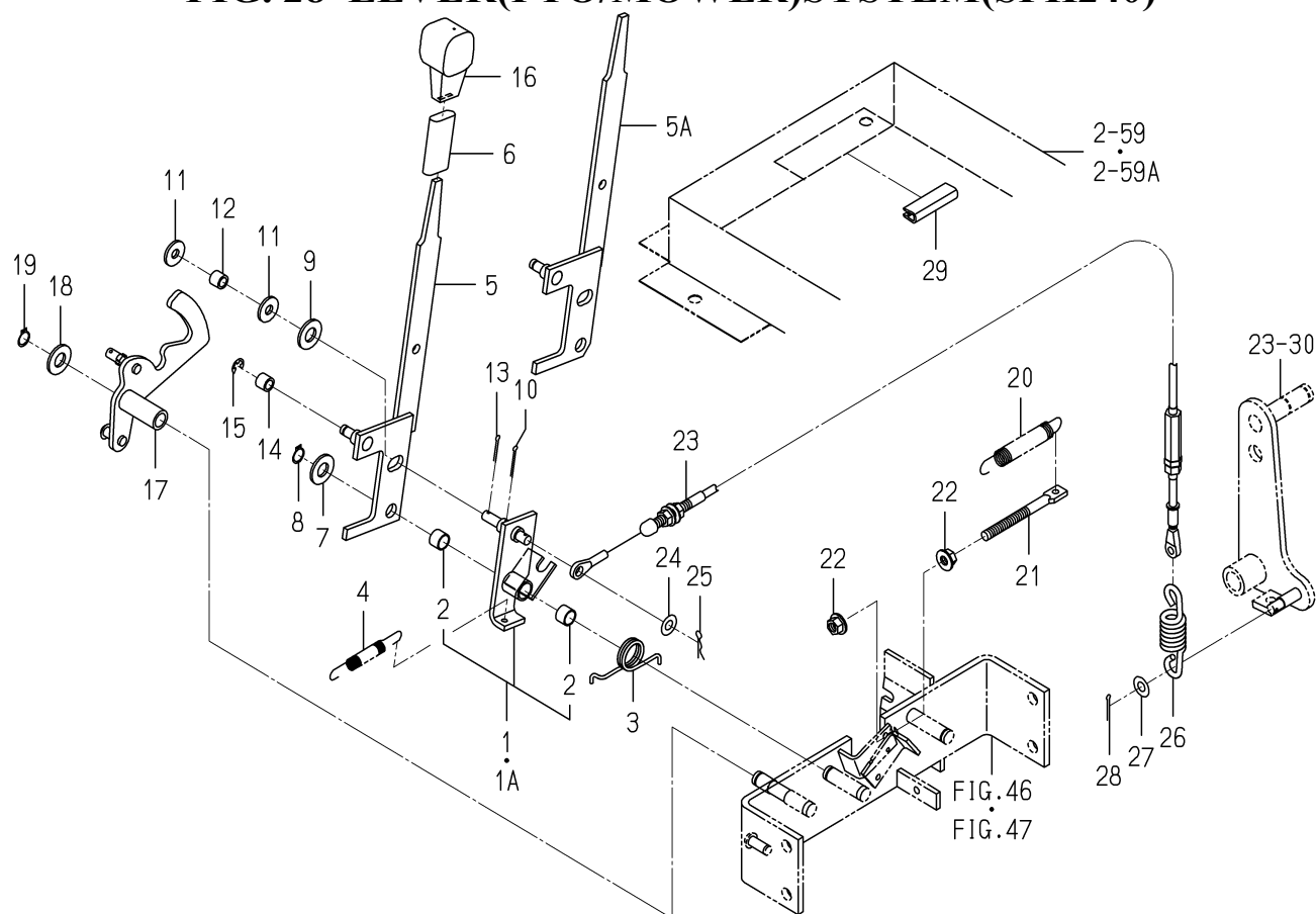
FIG. 28 LEVER(PTO/MOWER)SYSTEM(SFH240)
