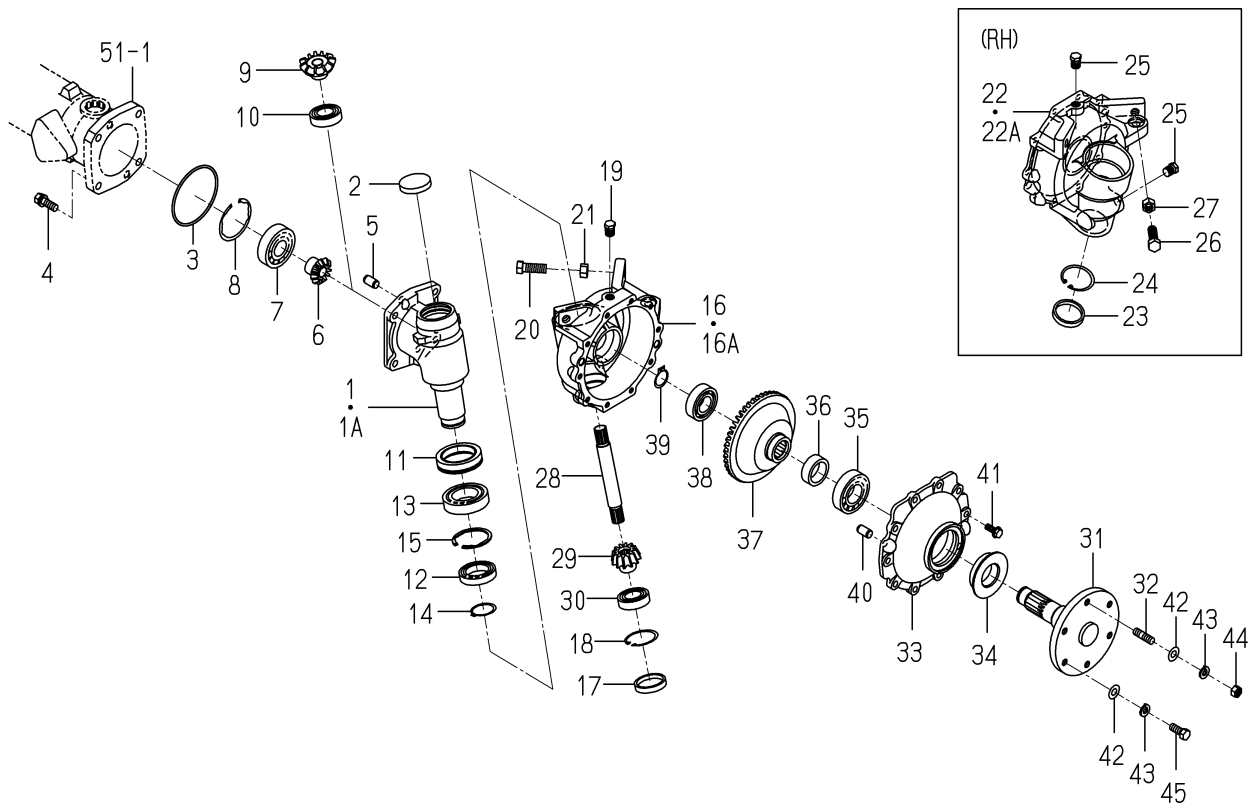
FIG. 53 CASE(GEAR/FINAL)SYSTEM(SFH240)
