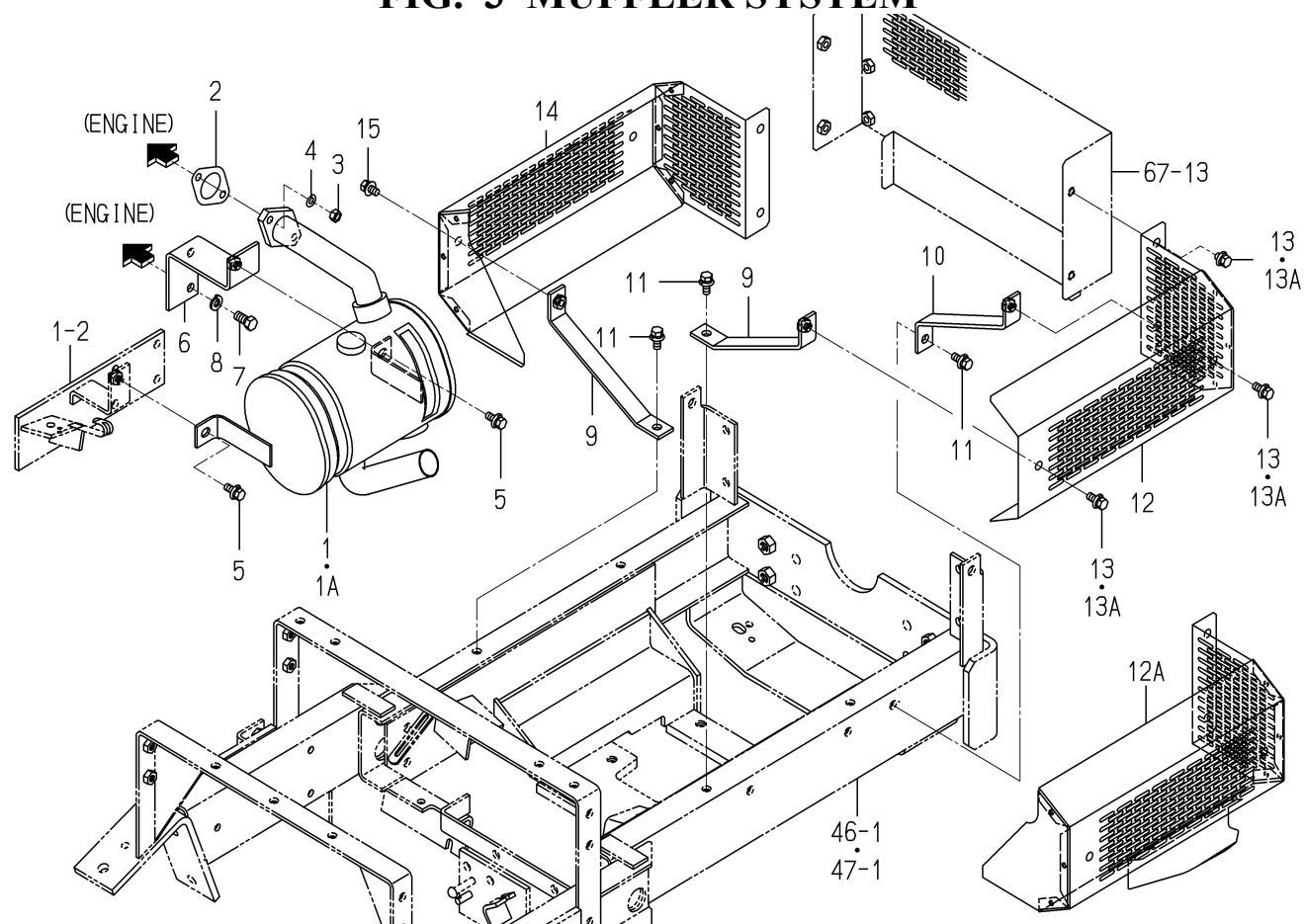
FIG. 3 MUFLER SYSTEM
