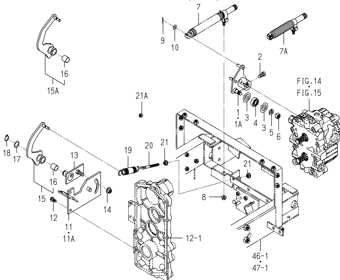
FIG. 26 LINK(HST)SYSTEM
