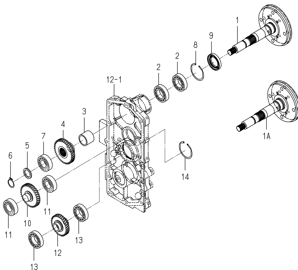
FIG. 13 GEAR(INPUT)SYSTEM
