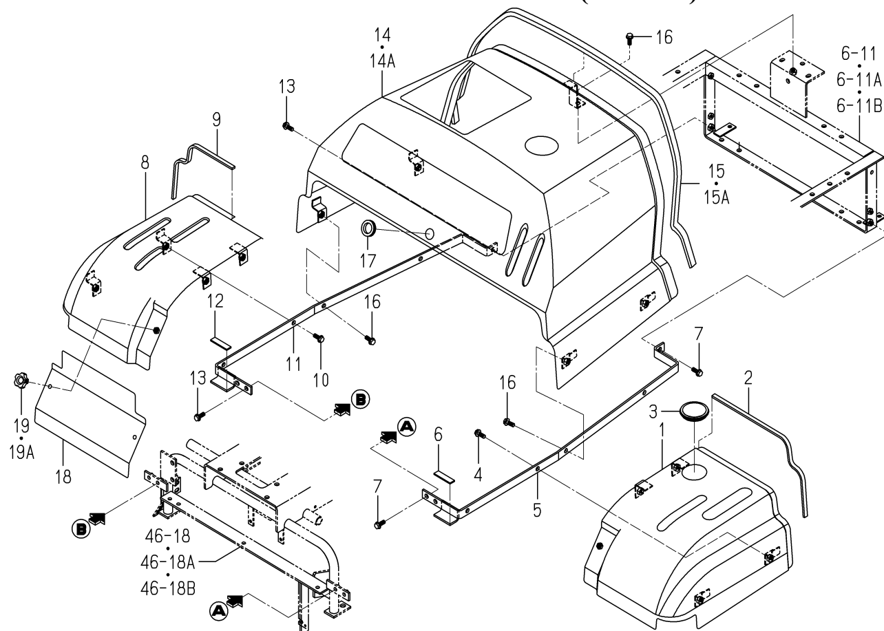
FIG. 70 FENDER SYSTEM(SFH240)
