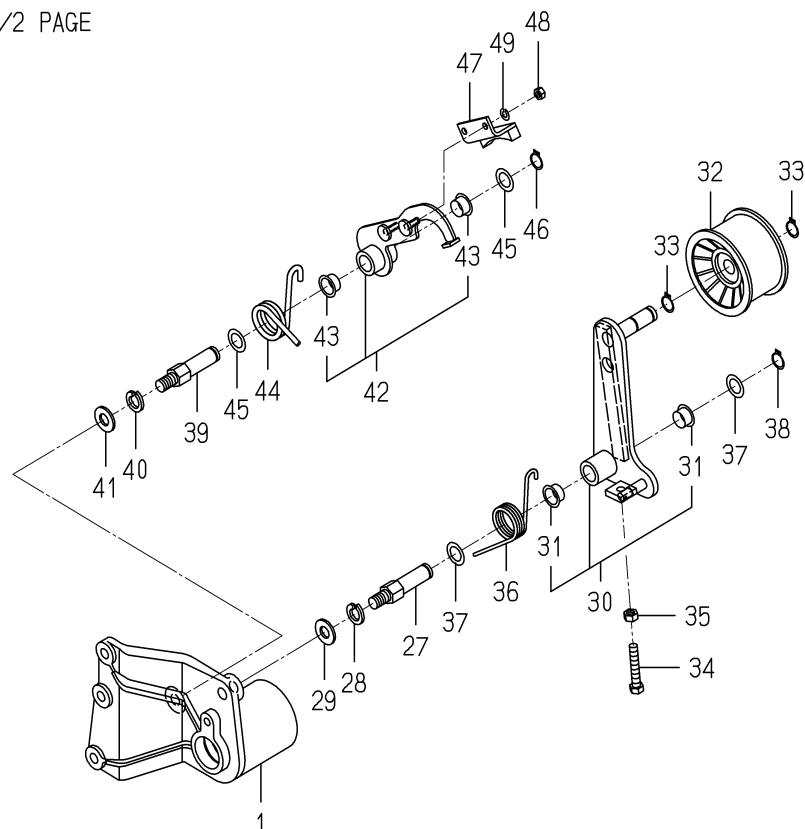
FIG. 23 DRIVE(PTO/MOWER)SYSTEM(SFH240)(2/2)
