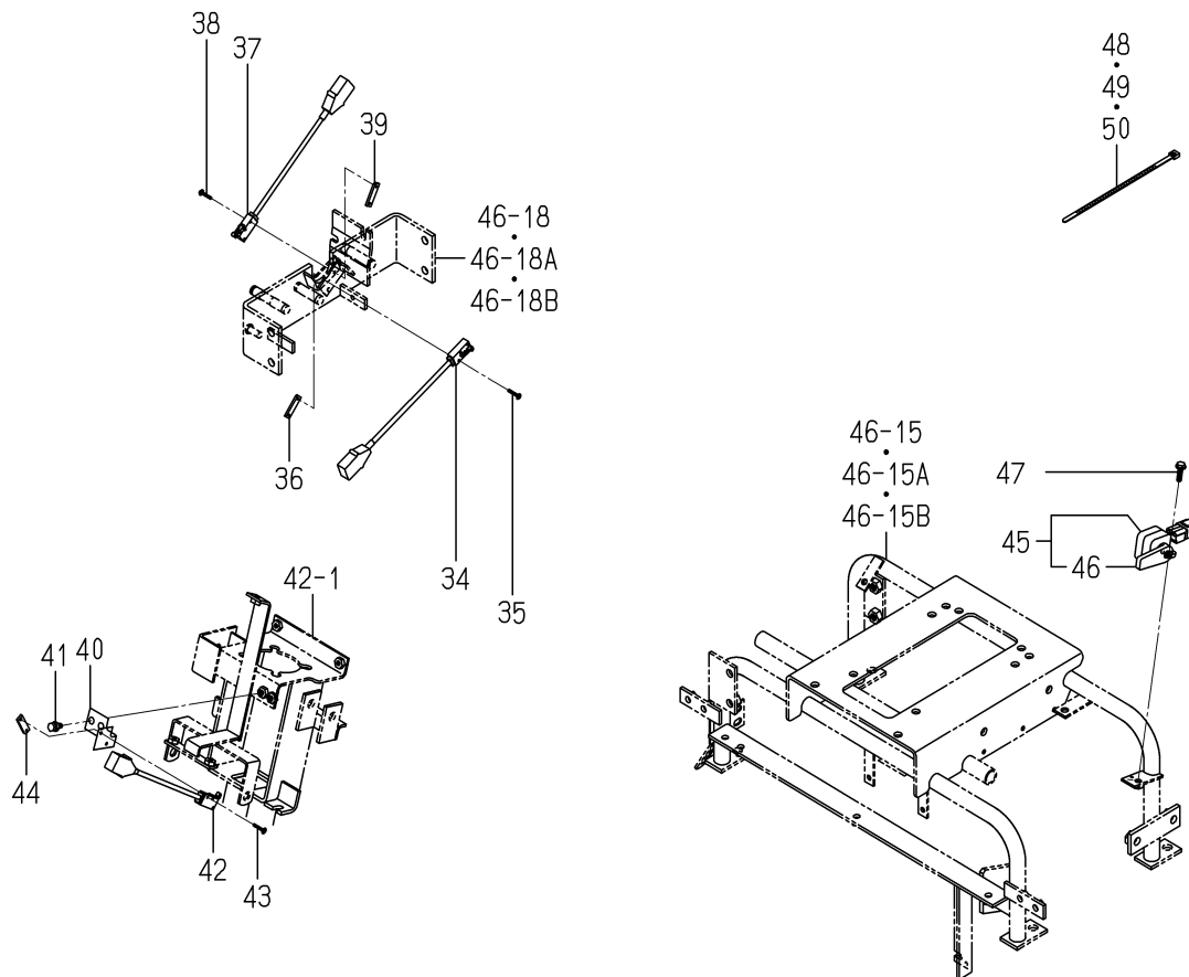
FIG. 78 HARNESS SYSTEM(SFH240:G TYPE)(2/2)
