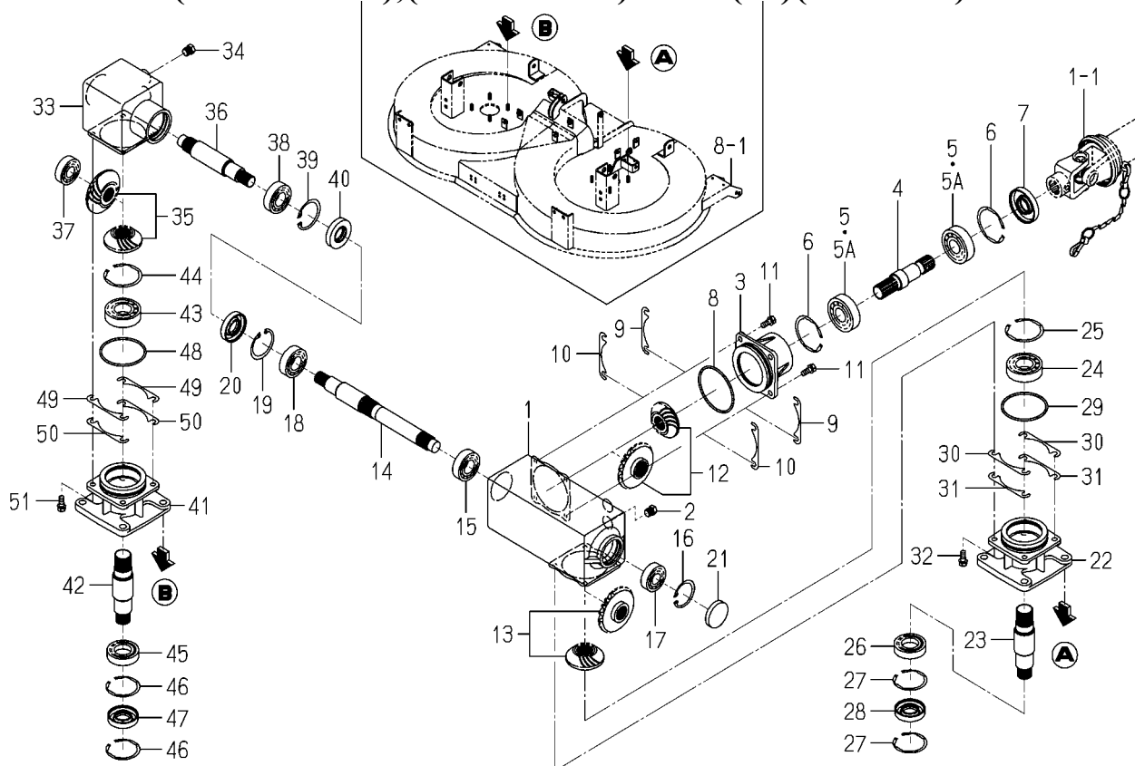
FIG. 16 CASE (BEVEL/LH),(BEVEL/RH)ASSY(54)(REPAIR)
