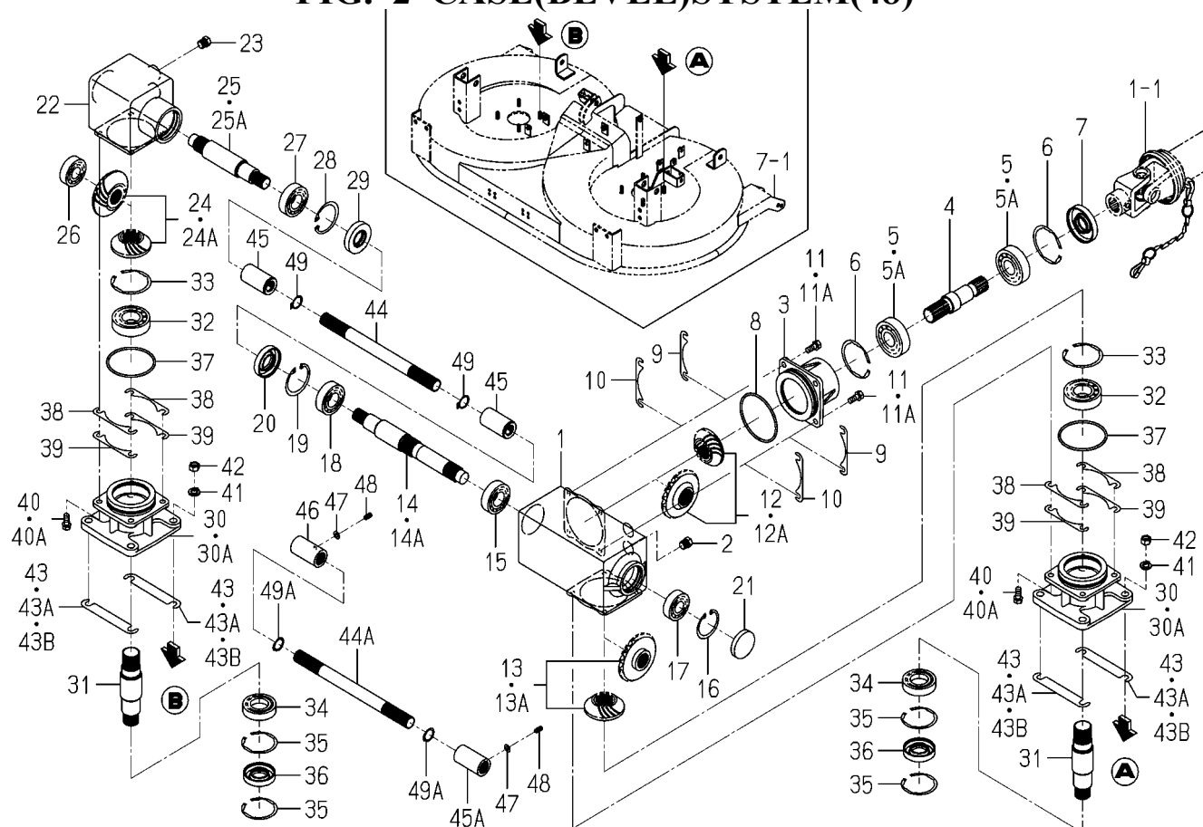
FIG. 2 CASE(BEVEL)SYSTEM(48)
