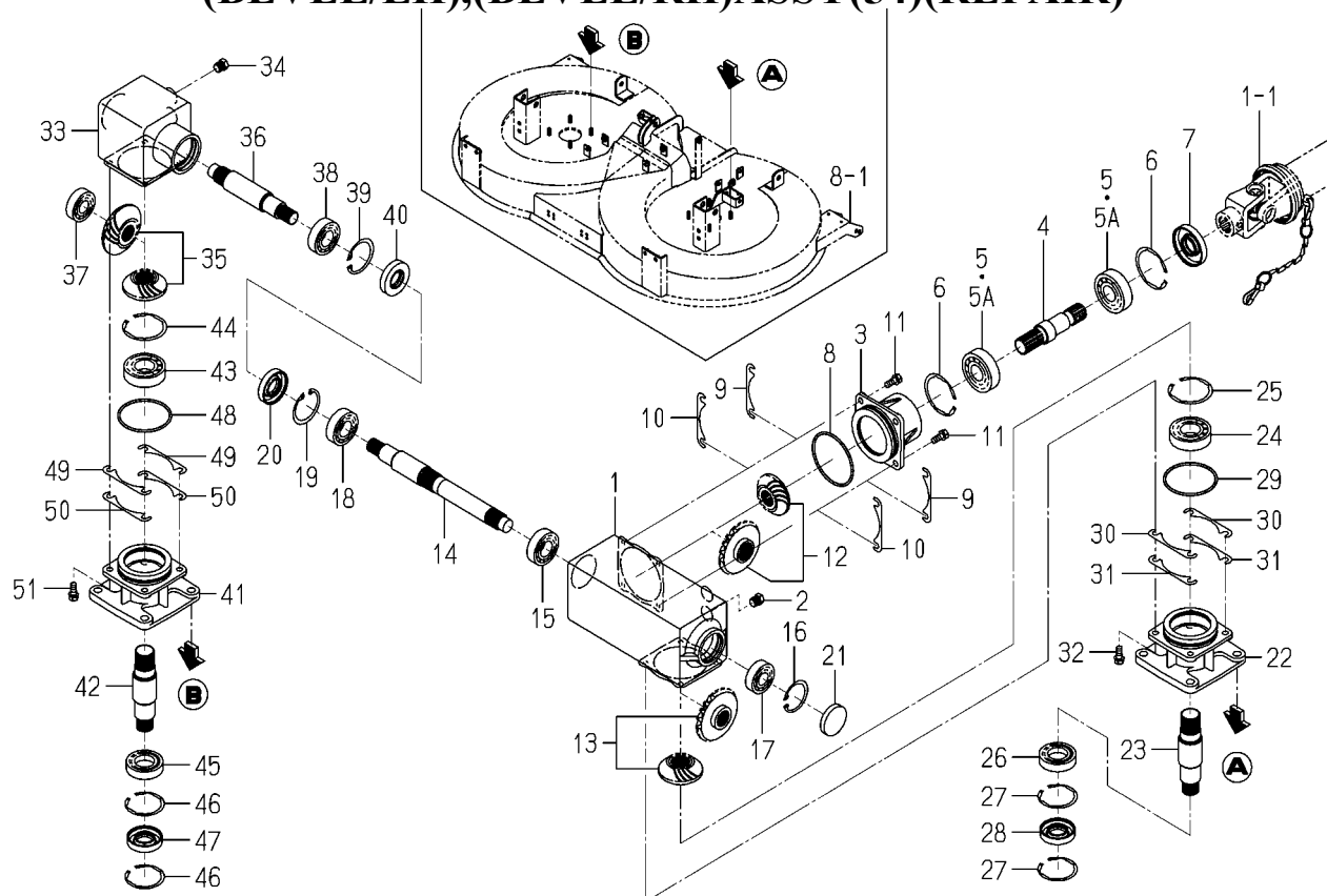
FIG. 16 CASE (BEVEL/LH),(BEVEL/RH)ASSY(54)(REPAIR)
