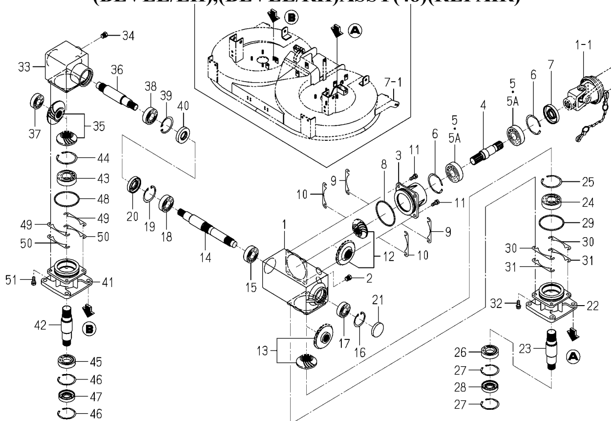
FIG. 15 CASE (BEVEL/LH),(BEVEL/RH)ASSY(48)(REPAIR)
