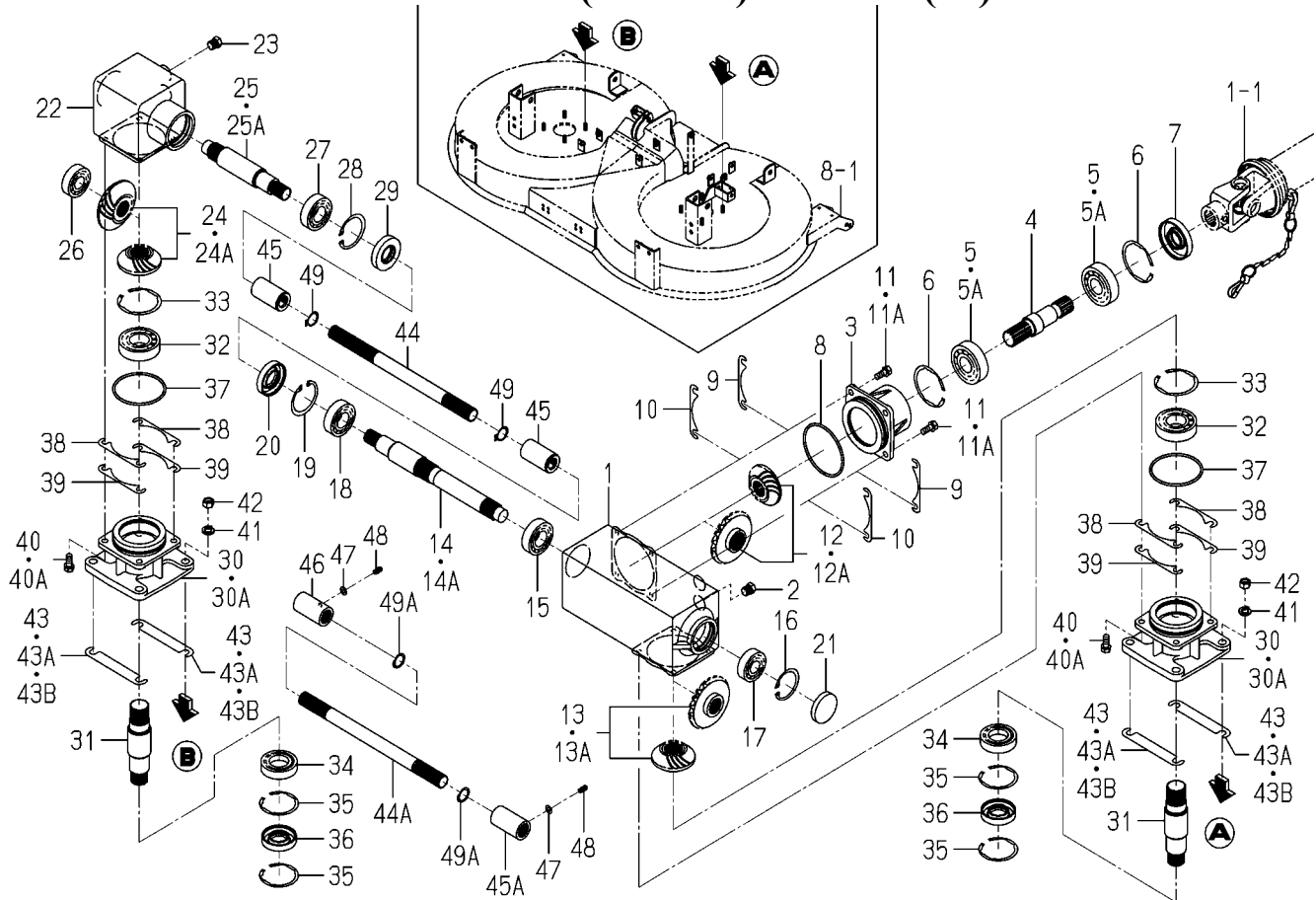
FIG. 3 CASE(BEVEL)SYSTEM(54)
