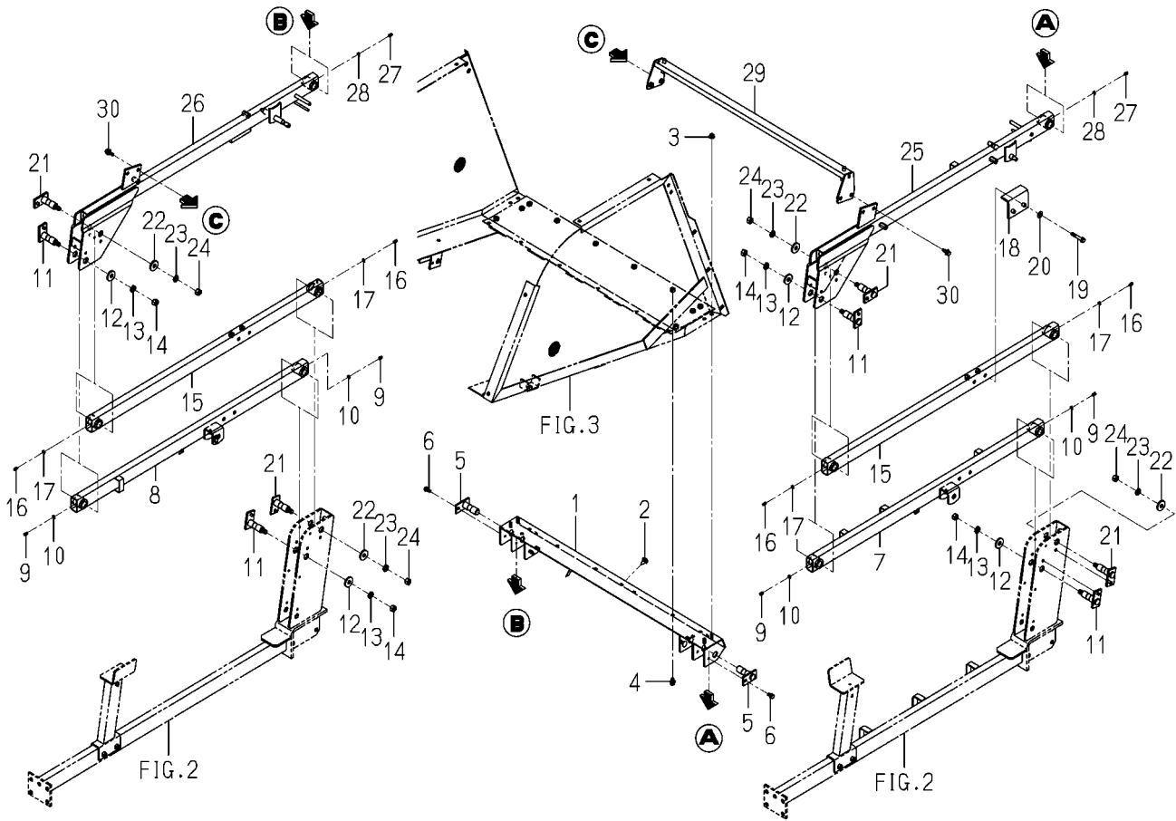
FIG. 7 LINK SYSTEM(H TYPE)
