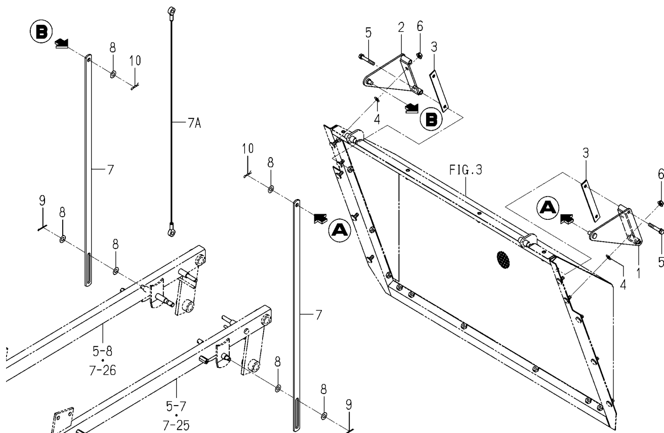
FIG. 4 DOOR SYSTEM
