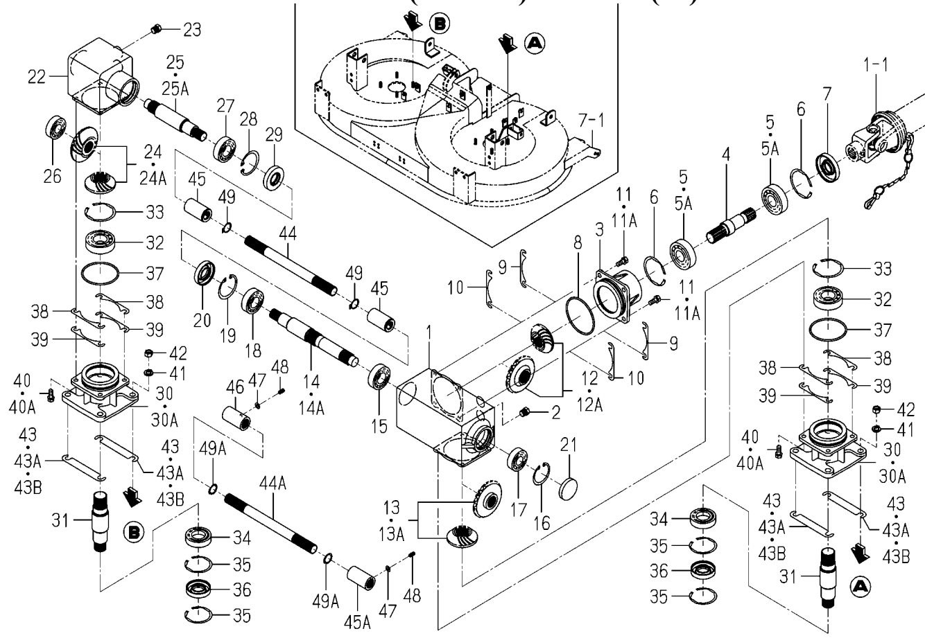
FIG. 2 CASE(BEVEL)SYSTEM(48)
