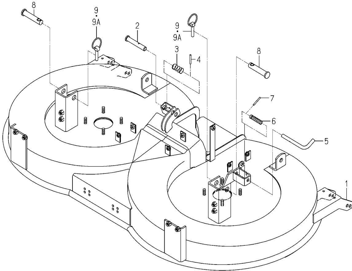
FIG. 8 DECK(MOWER)SYSTEM(54)
