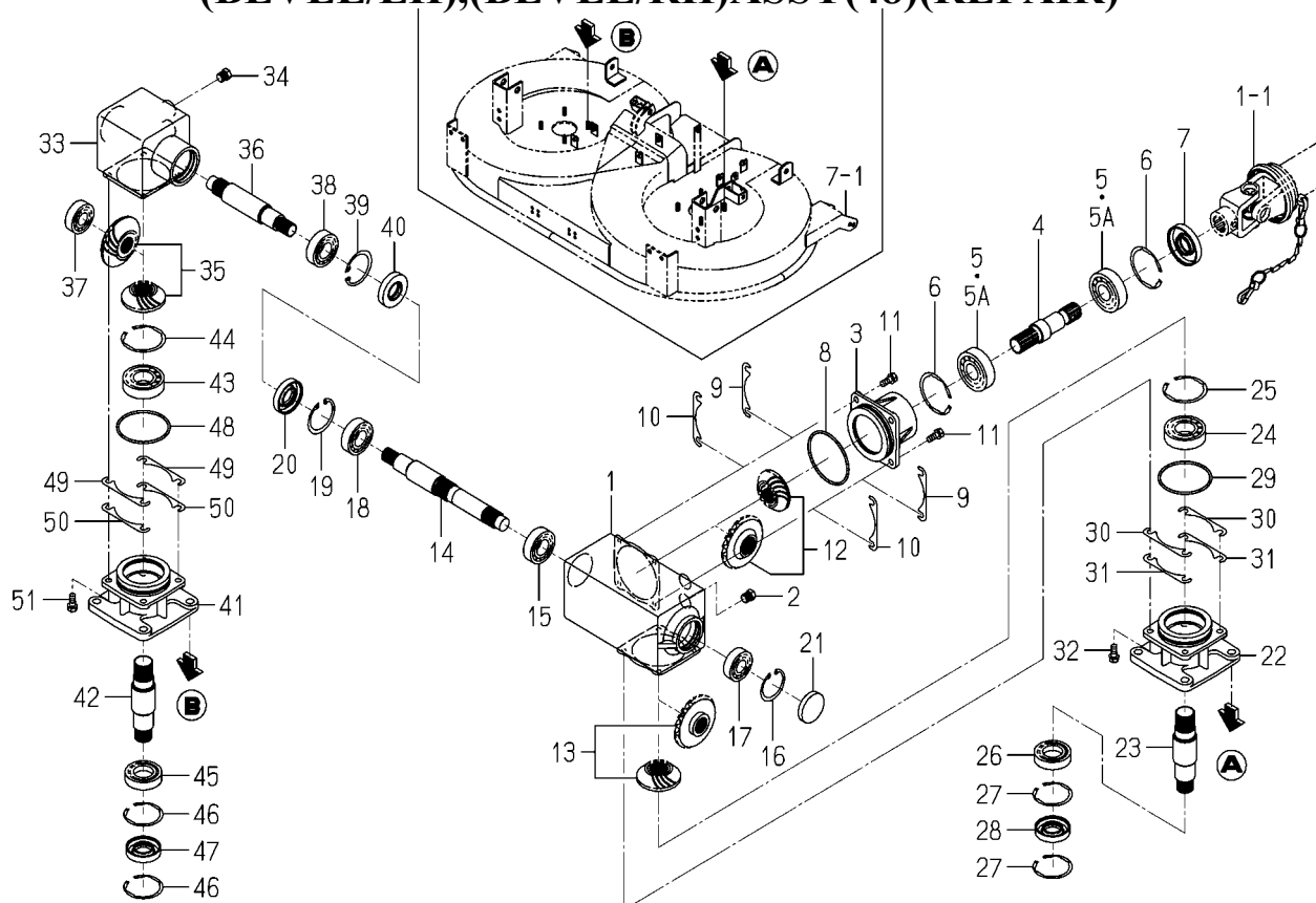
FIG. 15 CASE (BEVEL/LH),(BEVEL/RH)ASSY(48)(REPAIR)
