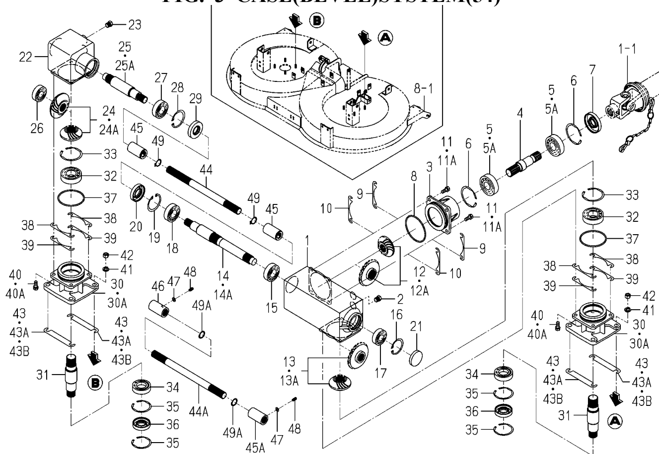
FIG. 3 CASE(BEVEL)SYSTEM(54)
