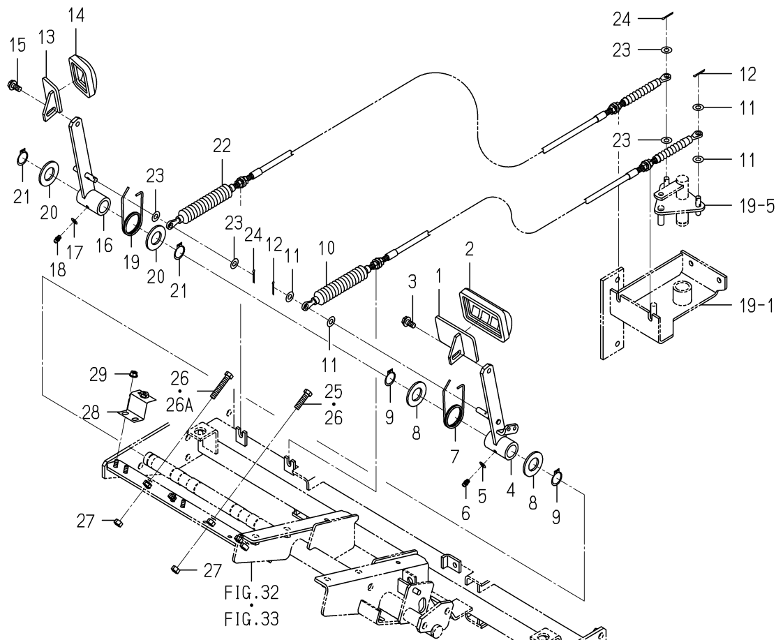
FIG. 20 PEDAL(HST)SYSTEM
