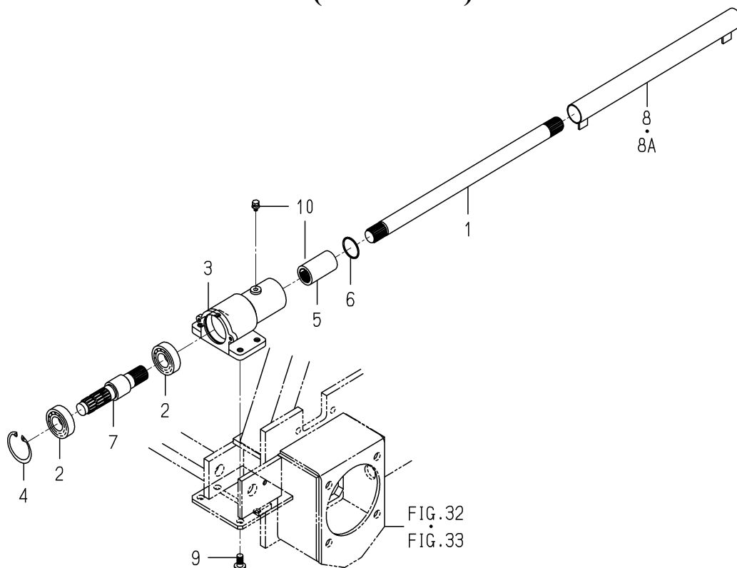
FIG. 17 SHAFT(PTO/SIDE)SYSTEM
