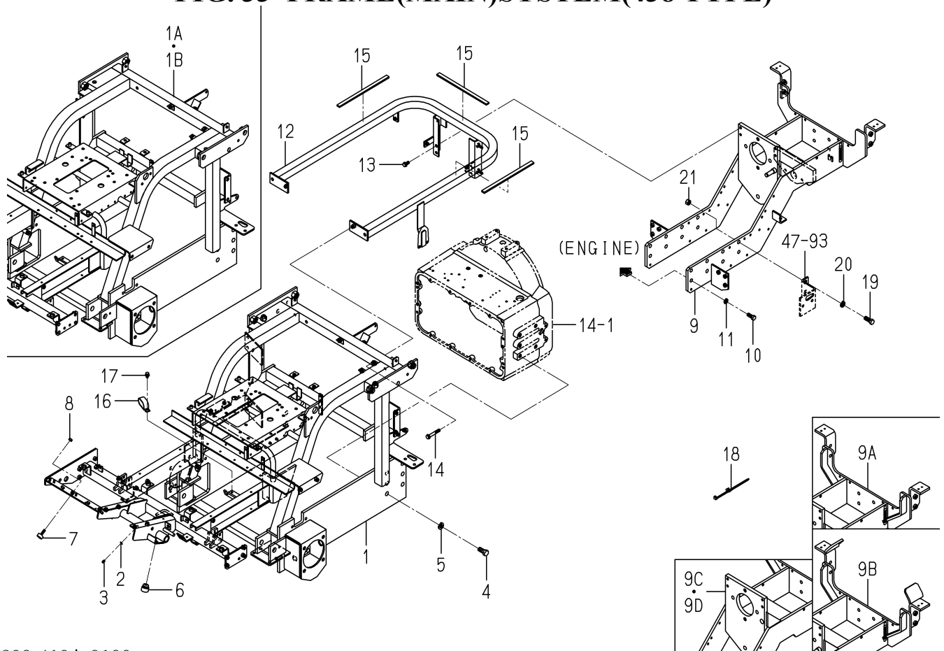
FIG. 33 FRAME(MAIN)SYSTEM(438 TYPE)
