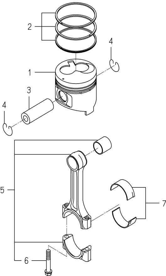
FIG. 16 PISTON
