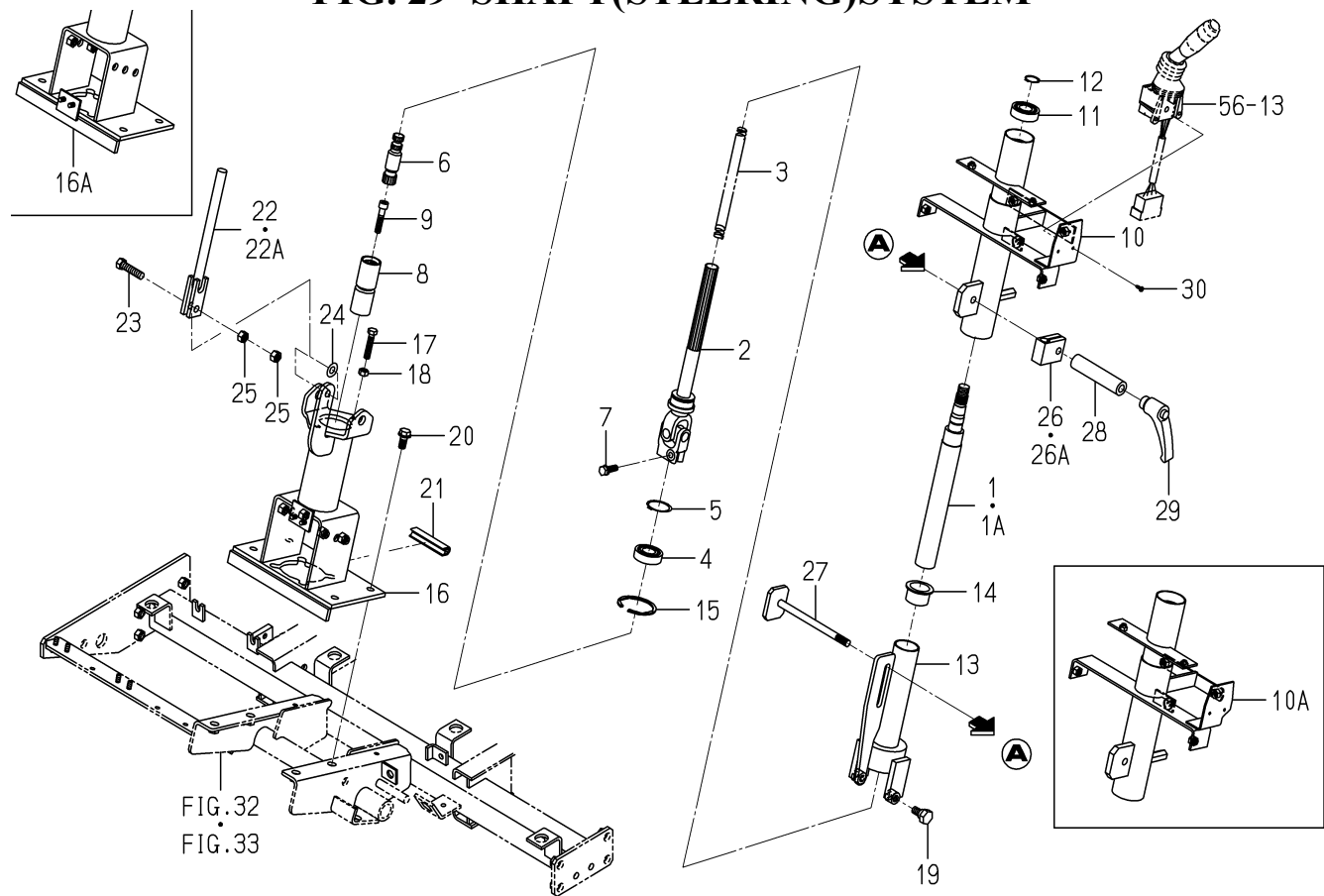
FIG. 29 SHAFT(STEERING)SYSTEM
