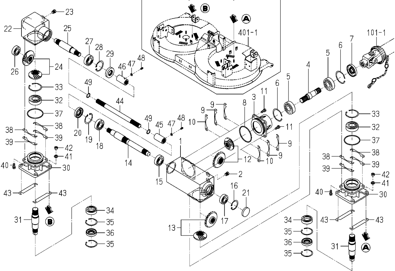
FIG.201 CASE(BEVEL)SYSTEM
