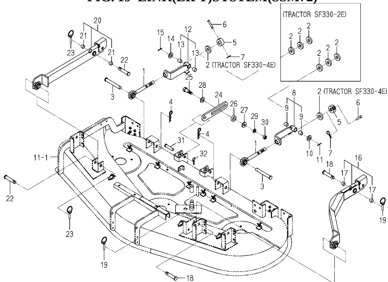
FIG. 19 LINK(LIFT)SYSTEM(SSM72)
