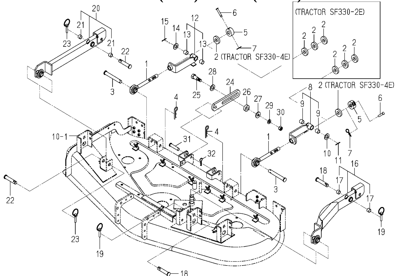
FIG. 18 LINK(LIFT)SYSTEM(SSM60)
