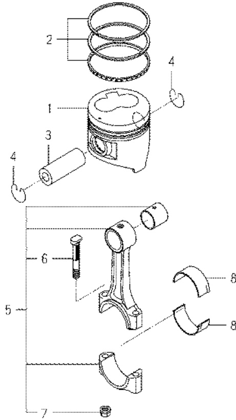
FIG. 13 PISTON
