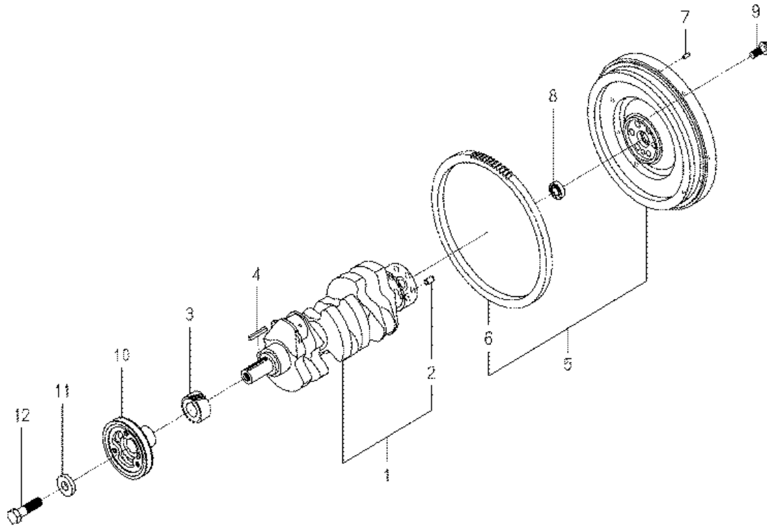
FIG. 15 CRANK SHAFT
