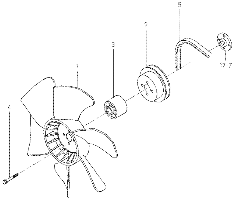
FIG. 18 COOLING FAN
