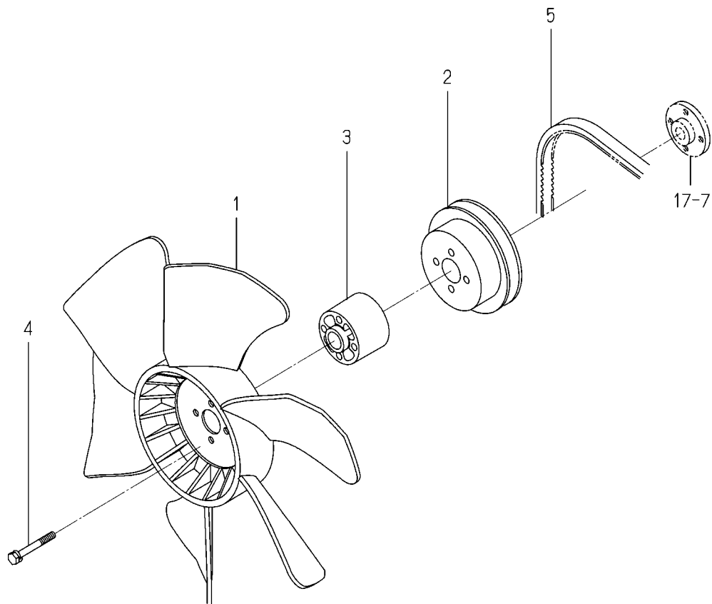
FIG. 18 COOLING FAN
