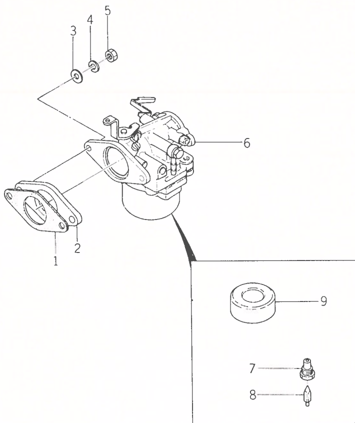
Fig. 5 CARBURETOR Carburateur
